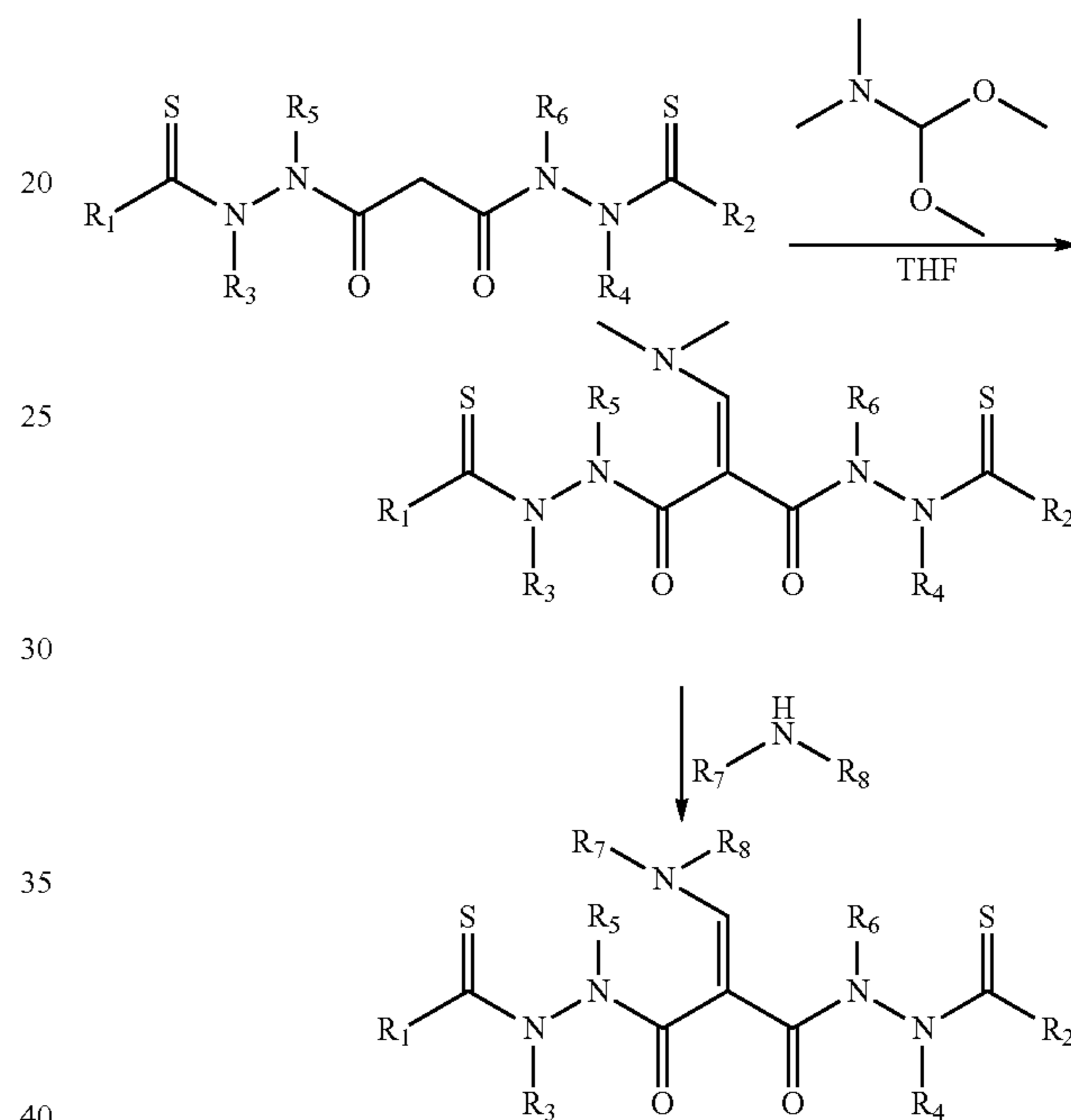
15 Scheme V:
