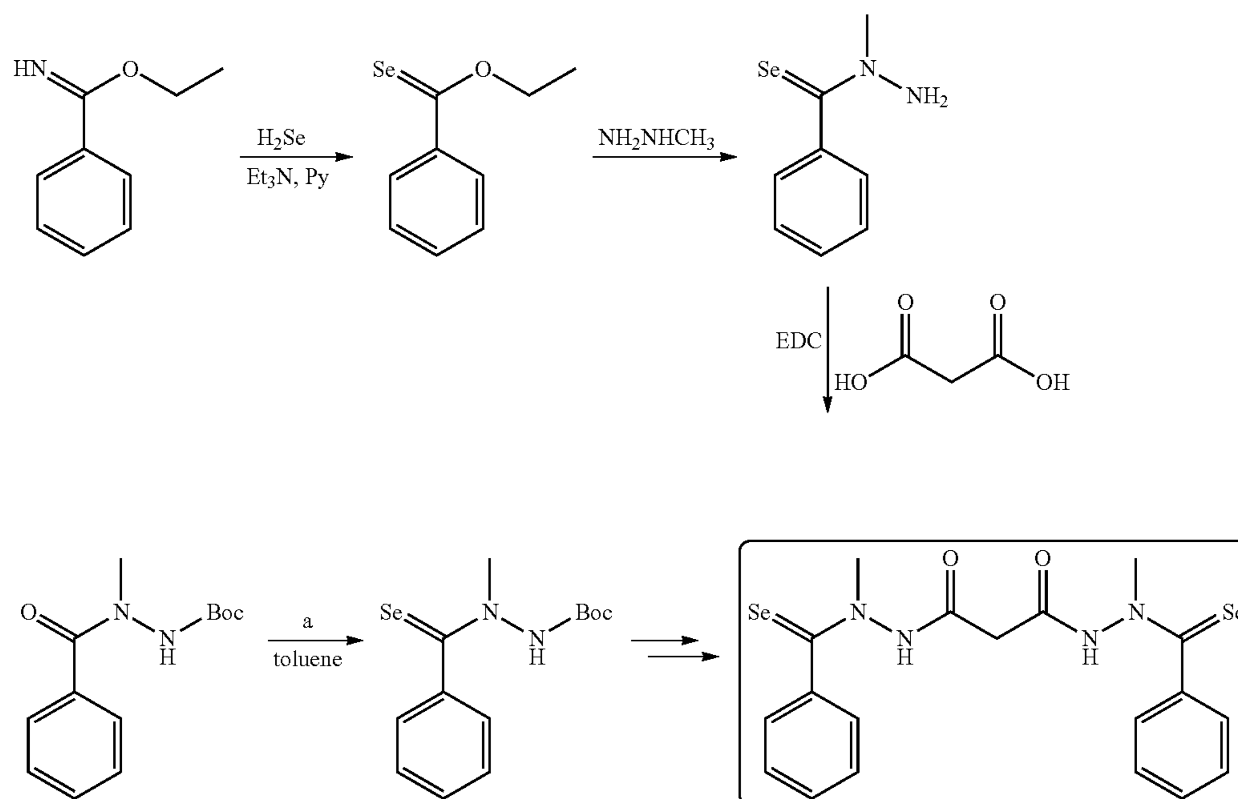
Scheme I:
