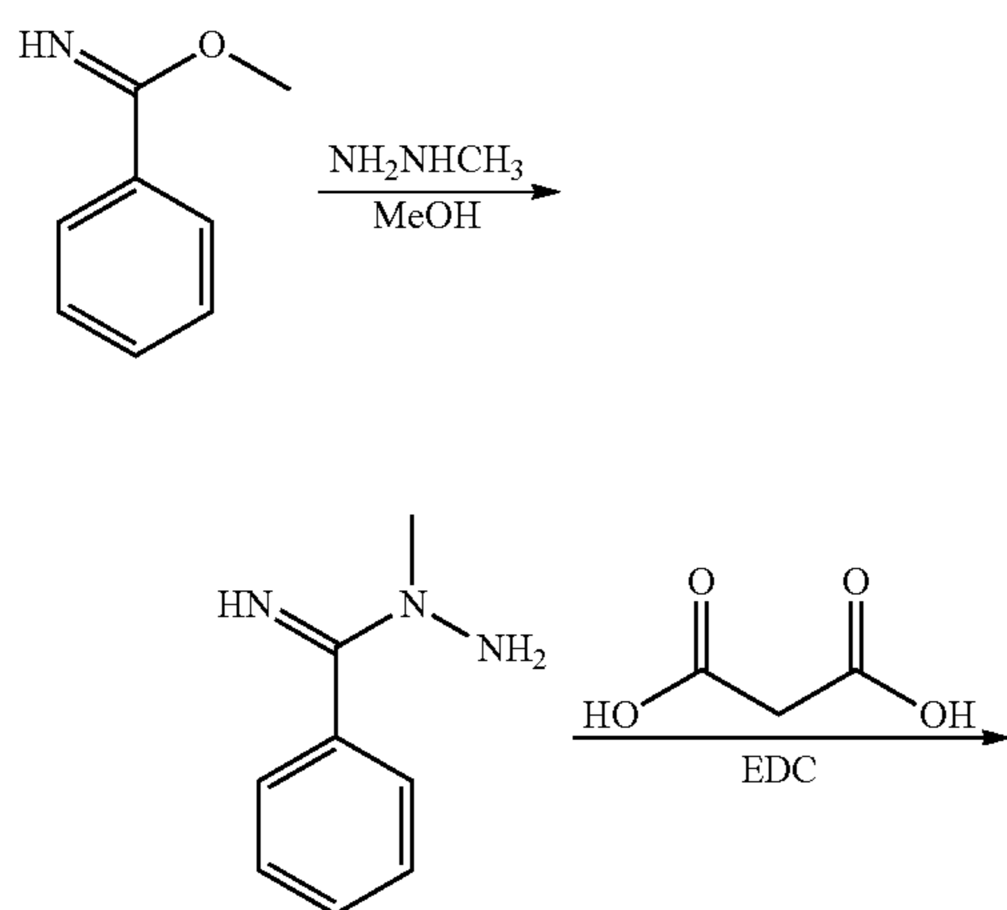
Scheme III:
