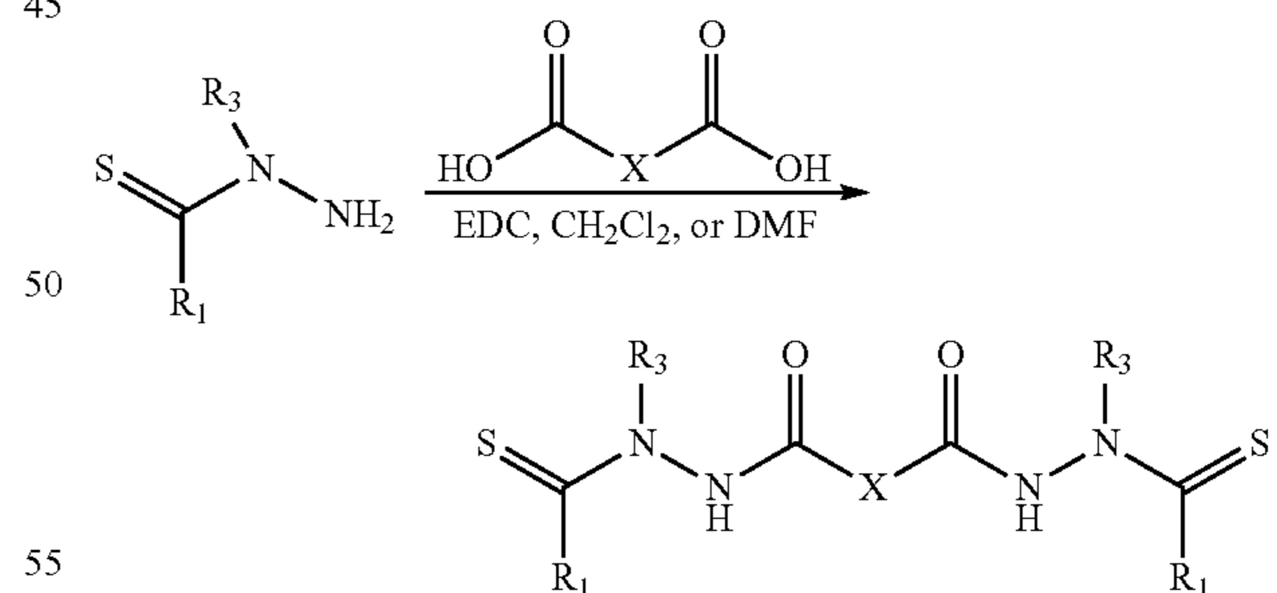
Scheme VI:
