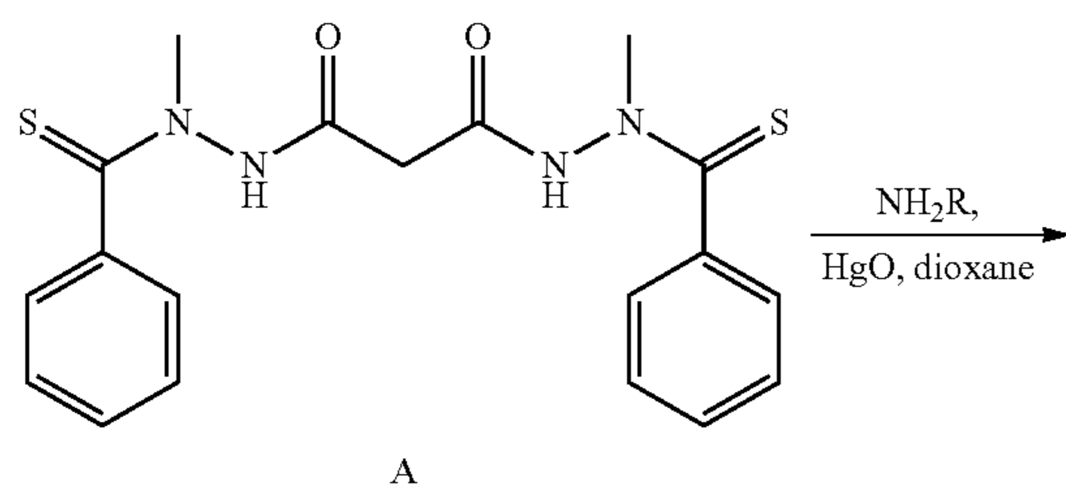
Scheme IV:
