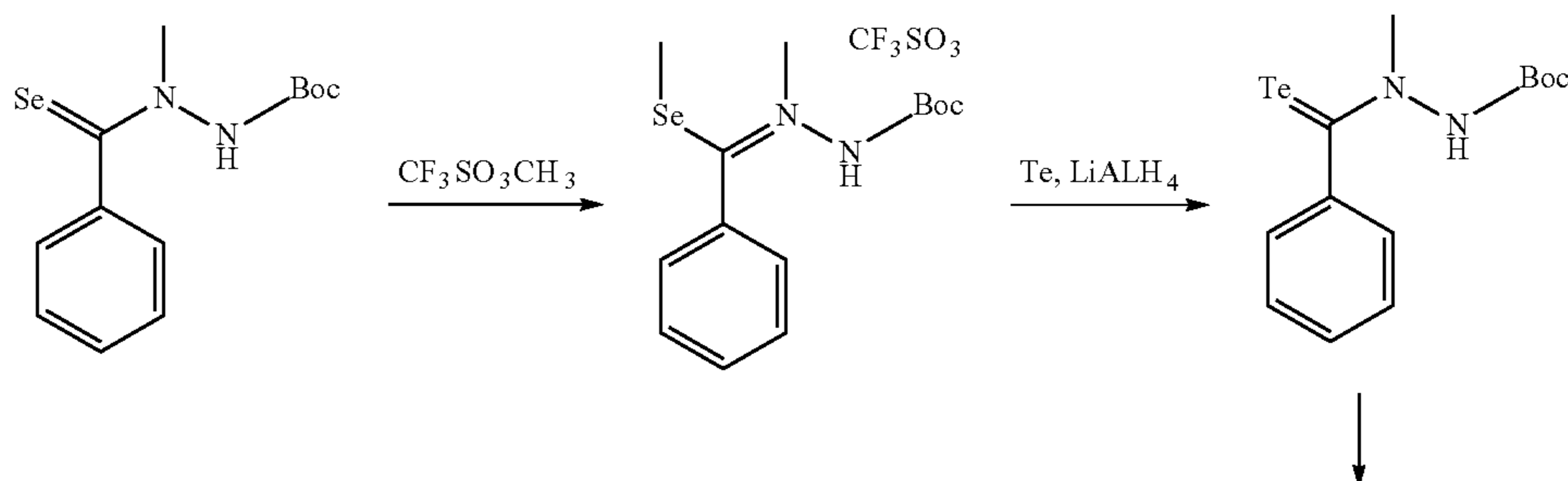
Scheme II:
