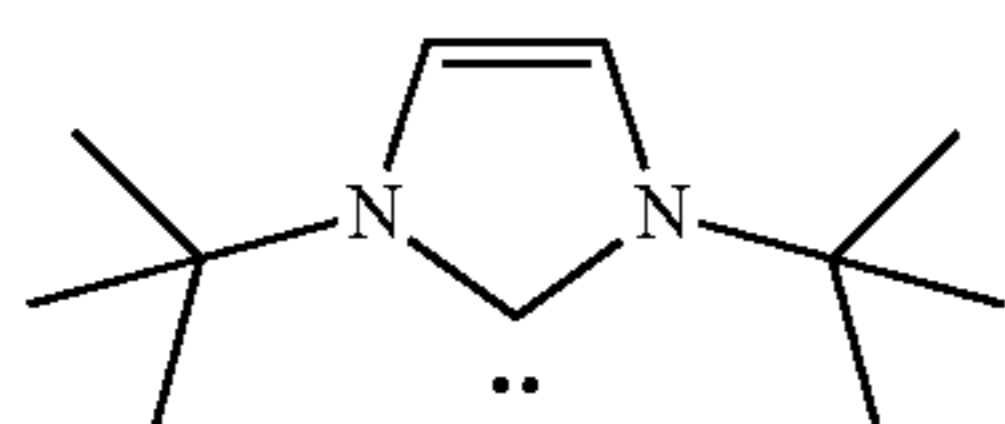
1,3-Di-t-butylimidazol-2-ylidene (Im-6)
