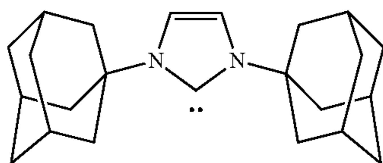
1,3-Bis(1-adamantyl)imidazol-2-ylidene (Im-4)
