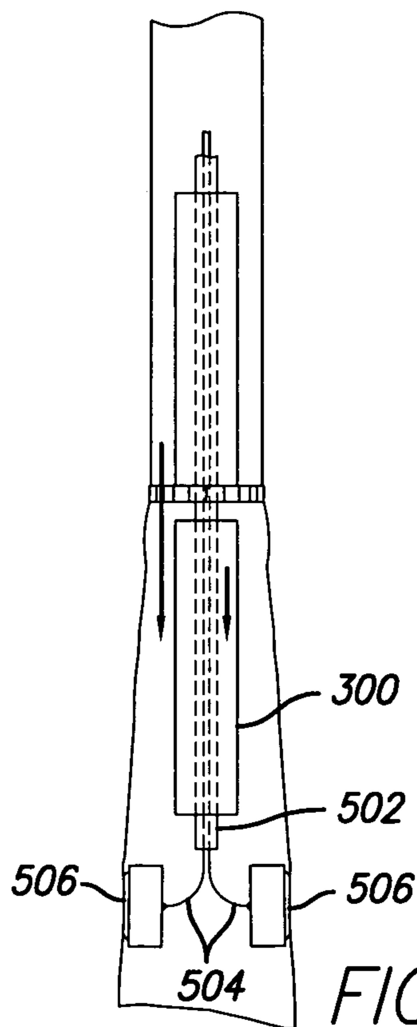
FIG. 55B
