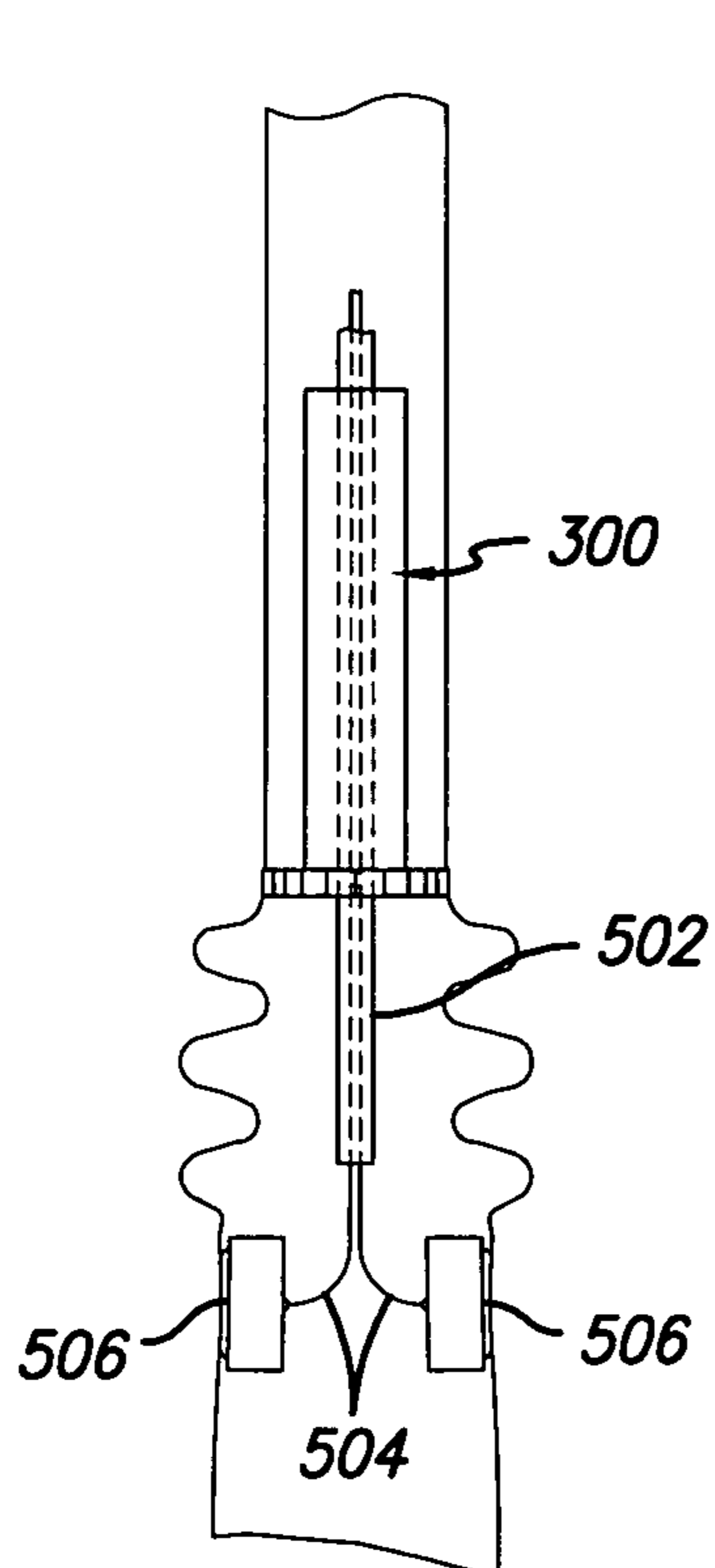
FIG. 55C
