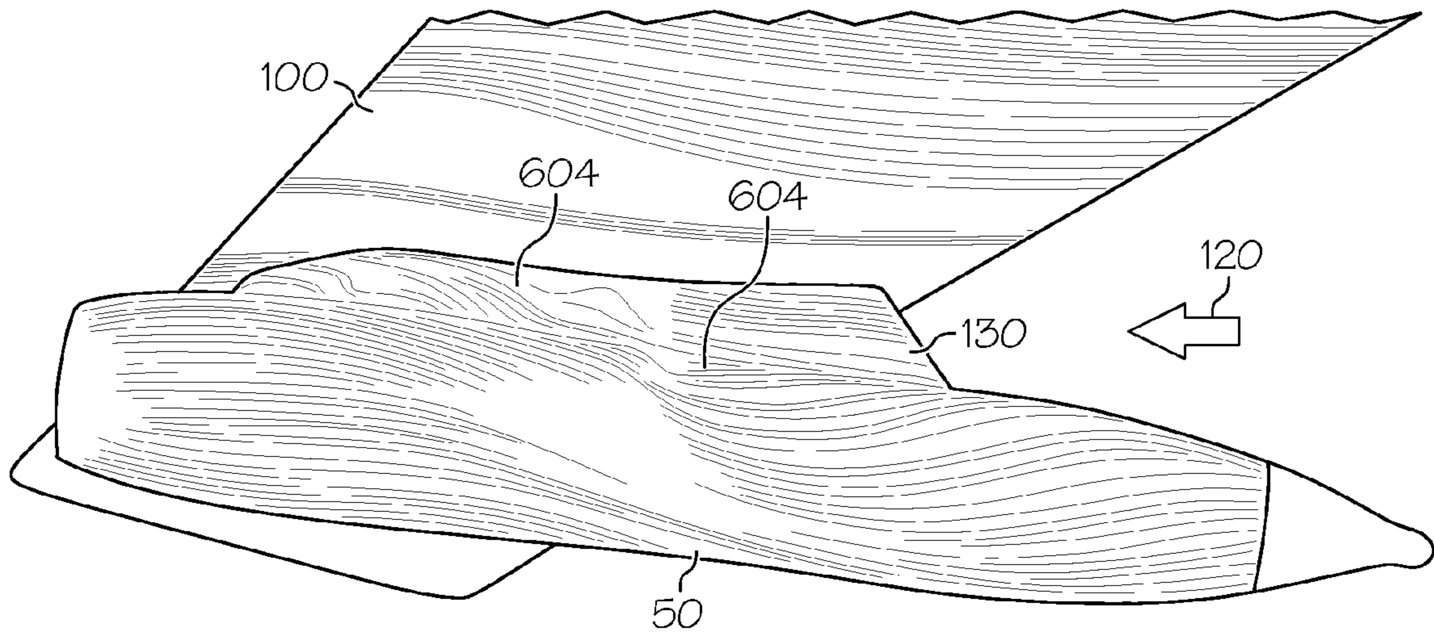
FIG. 12A
