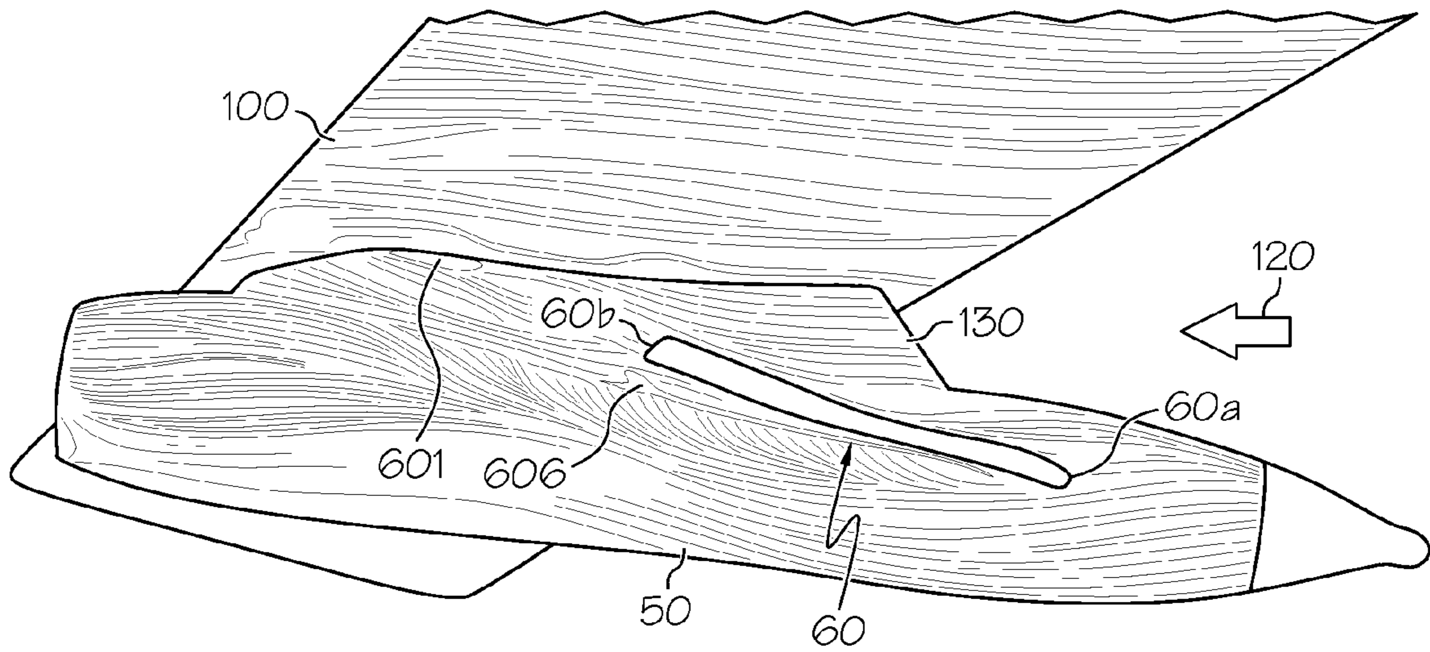
FIG. 12B
