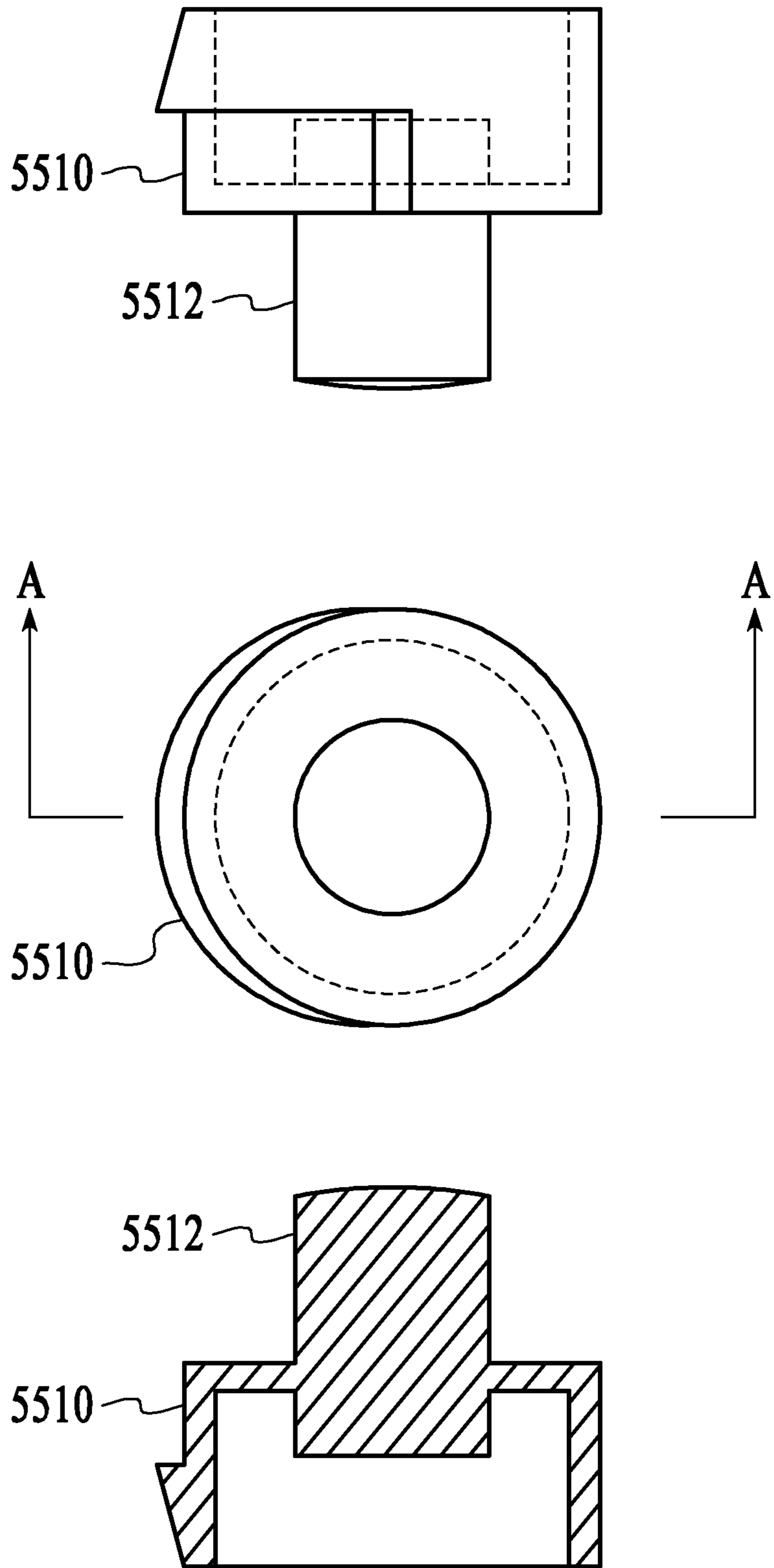
Section A-A
