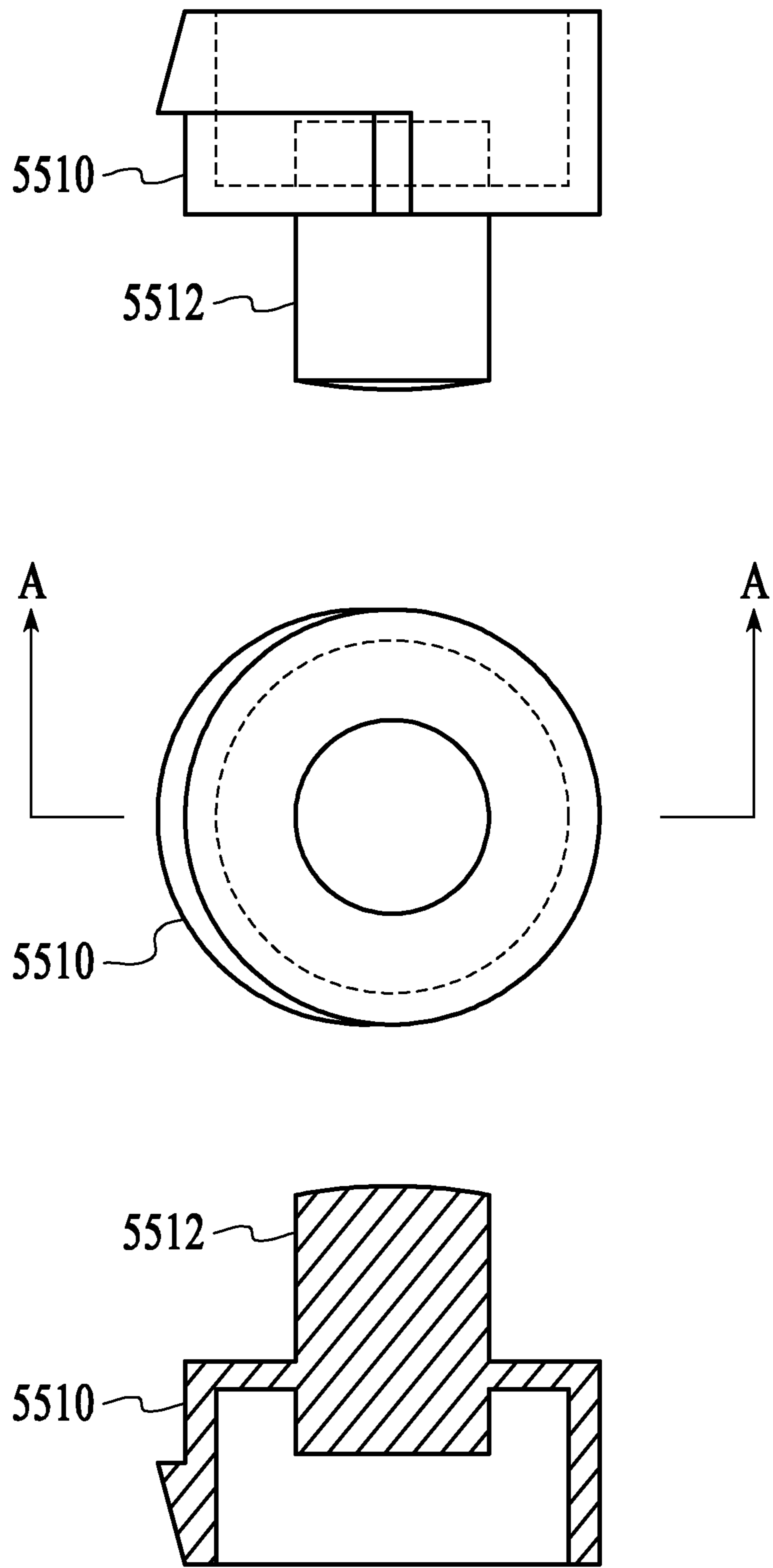
Section A-A
