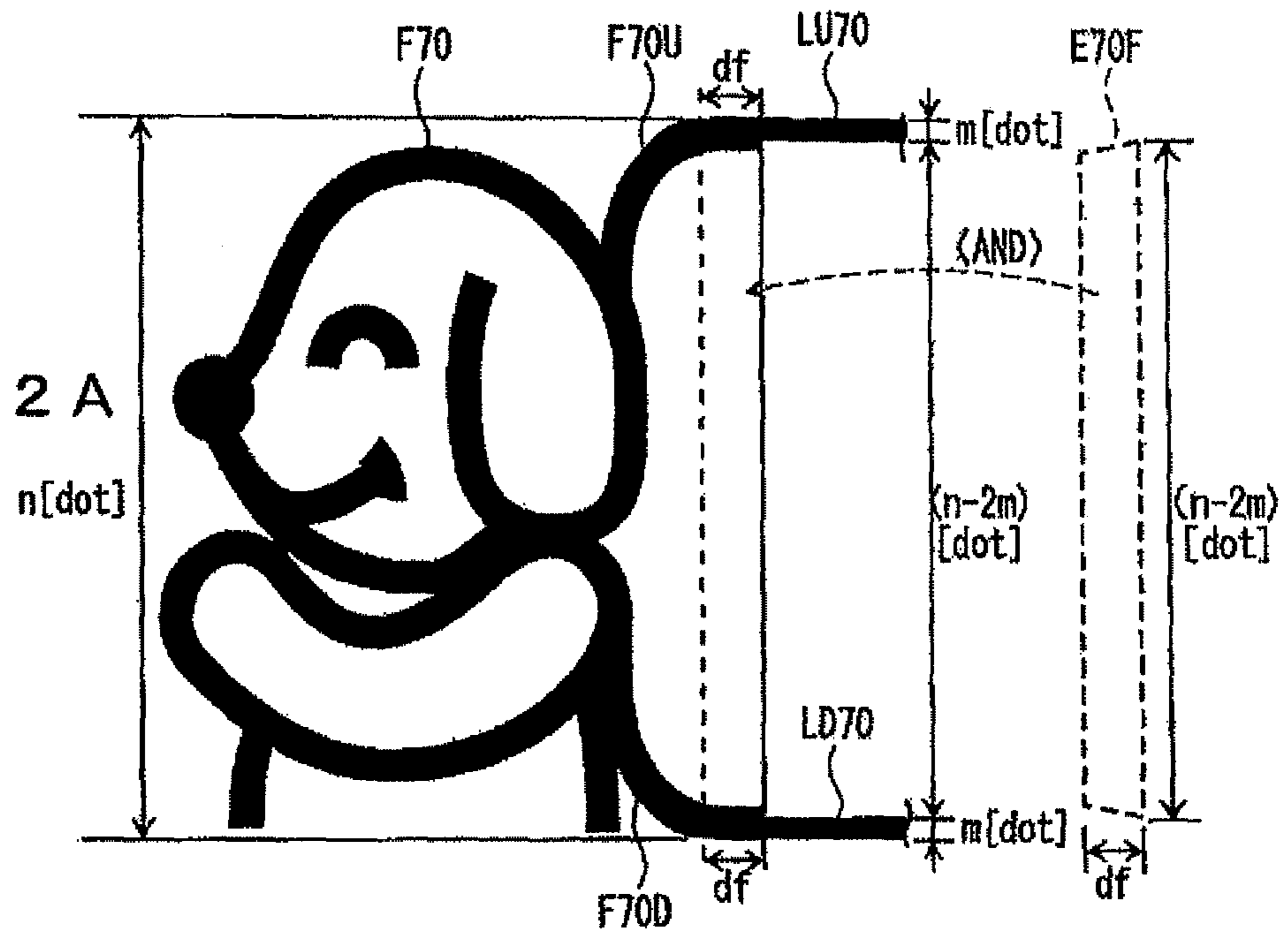
FIG. 12B
