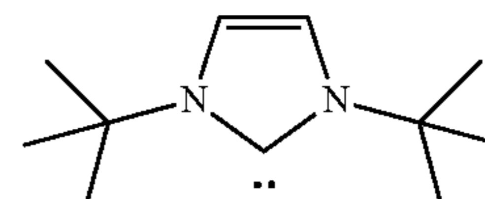
1,3-Di-t-butylimidazol-2-ylidene (Im-6)
