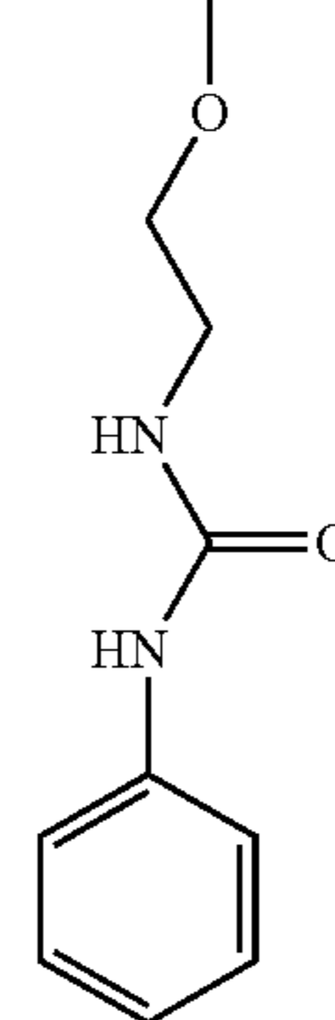
(MTCU)
