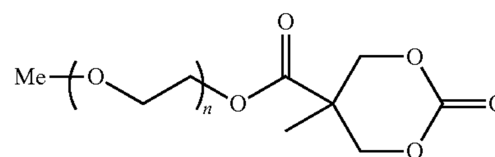
(MTCOMPEG)
