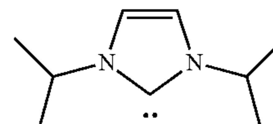
1,3-Di-i-propylimidazol-2-ylidene (Im-5)
