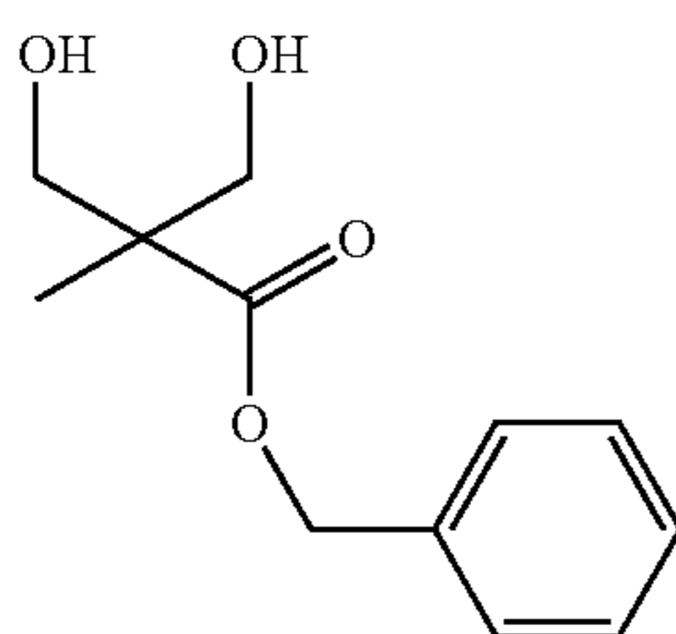
(BnMPA)
