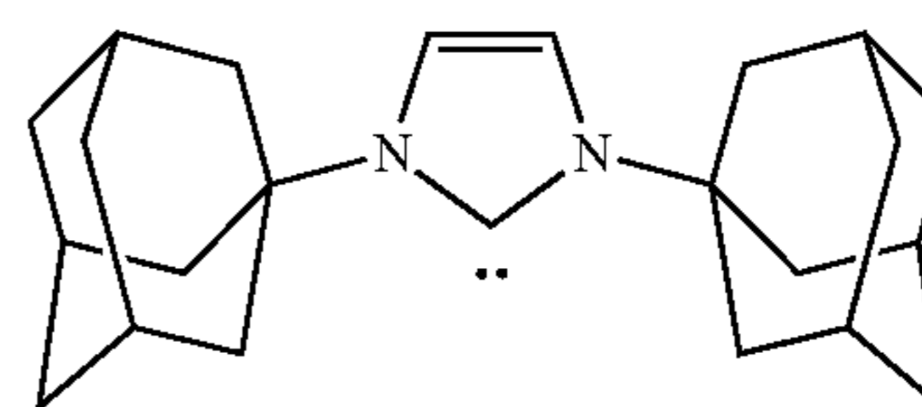
1,3-Bis(1-adamantyl)imidazol-2-yliden (Im-4)
