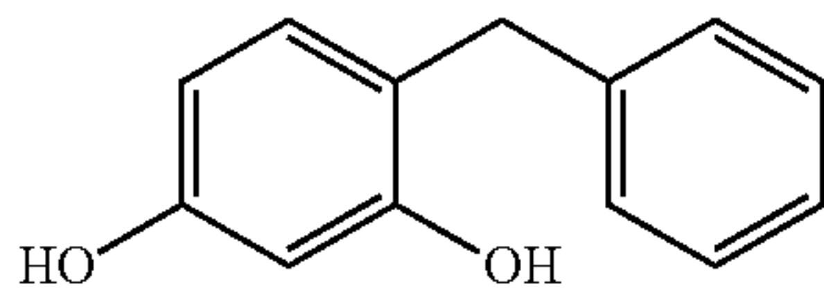
4-benzyl-benzene-1,3-diol
