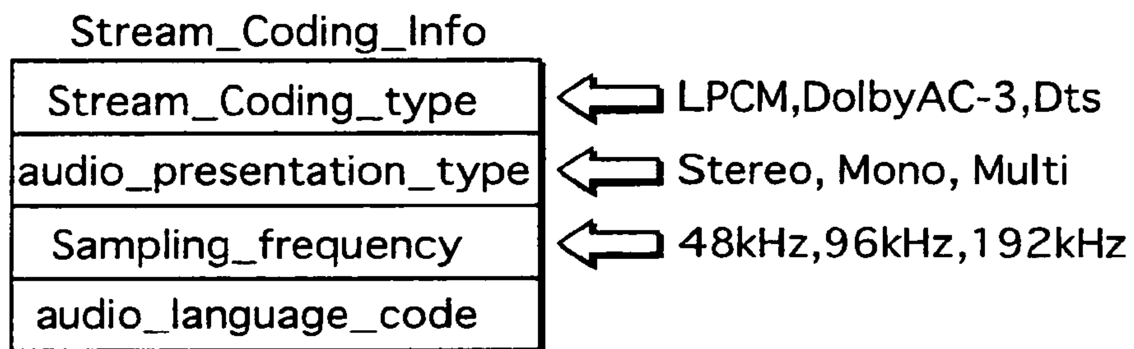
FIG. 11 B
