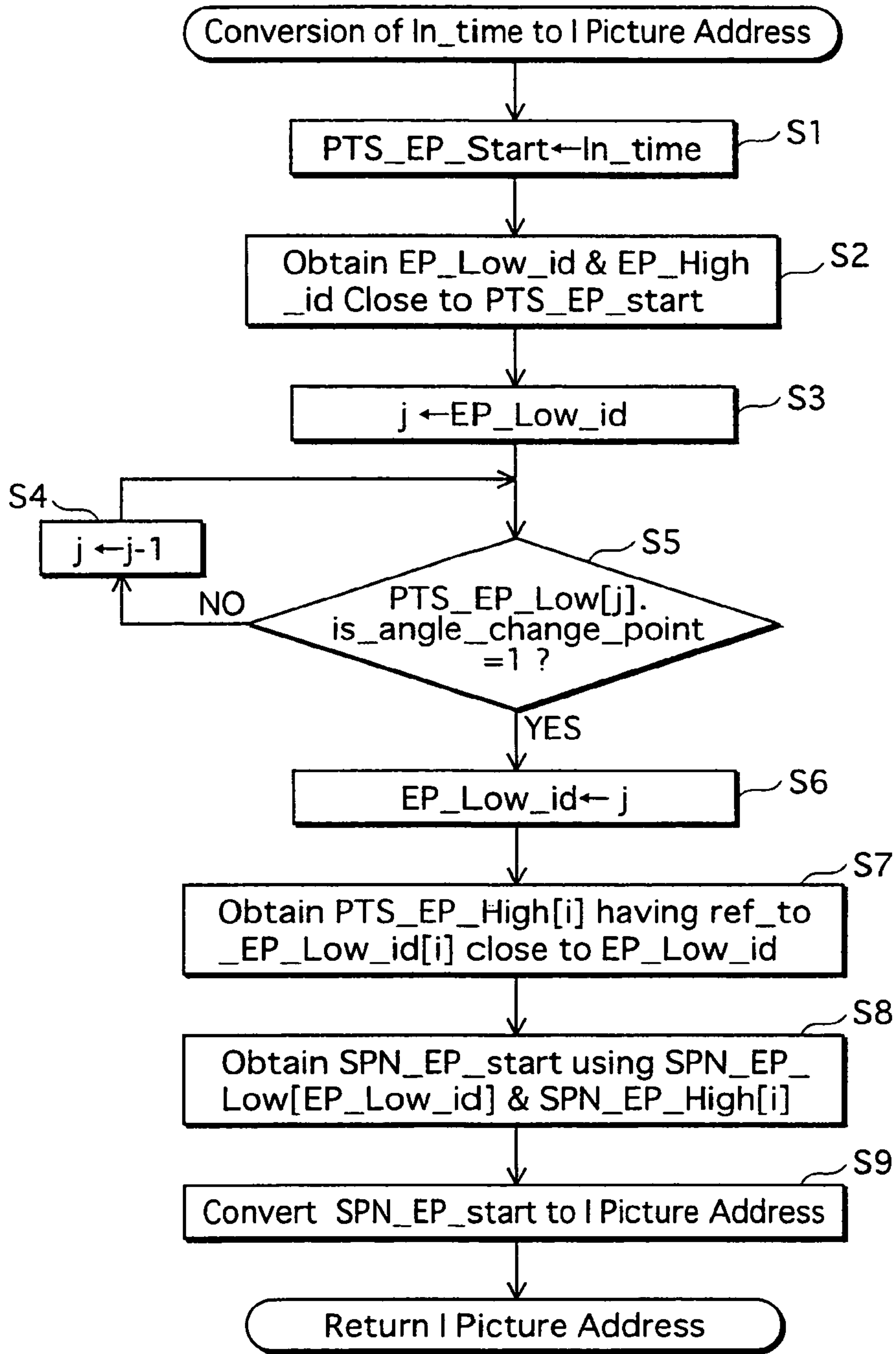
FIG. 22
