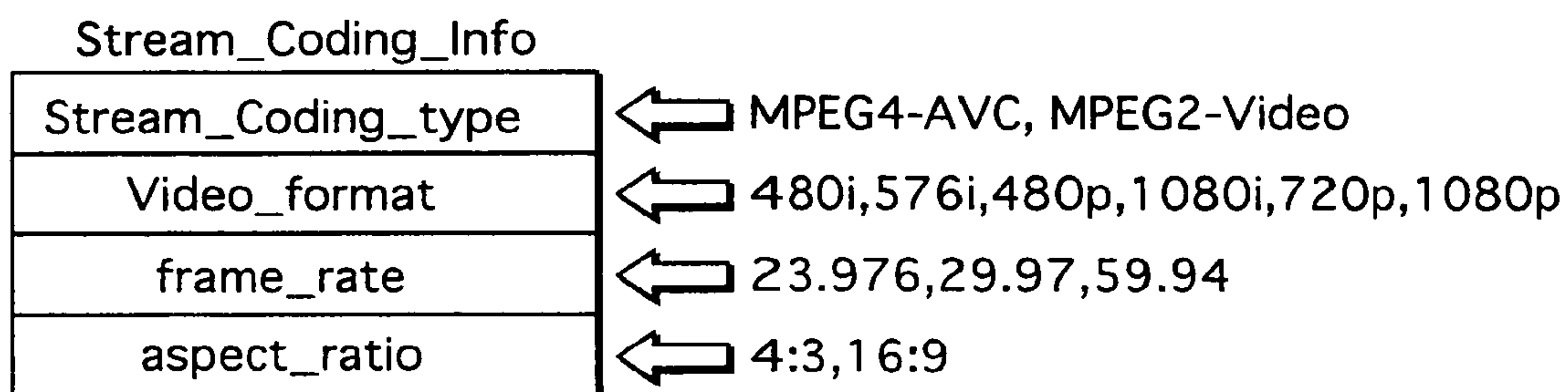
FIG. 11 A
