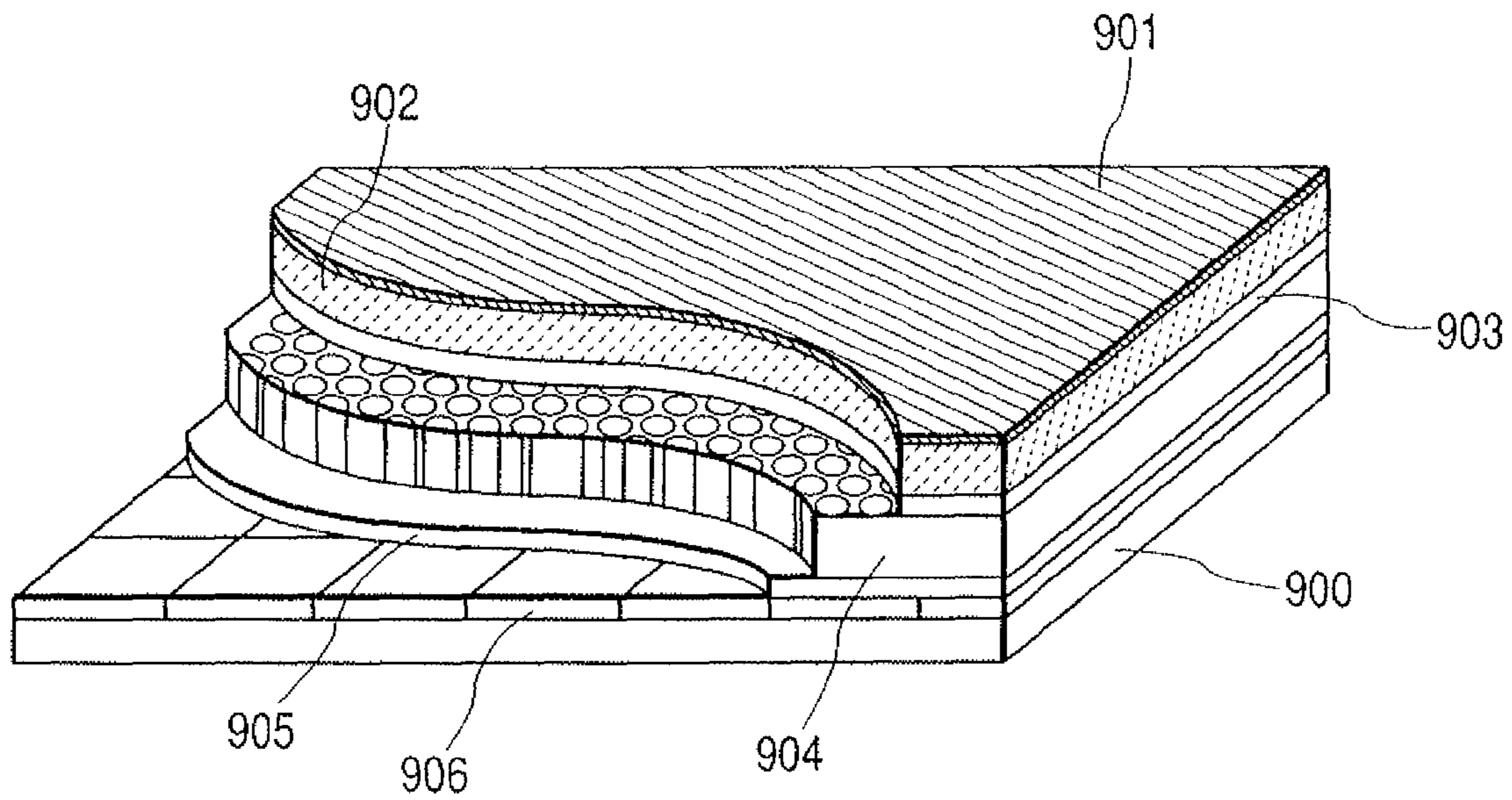
FIG. 11
