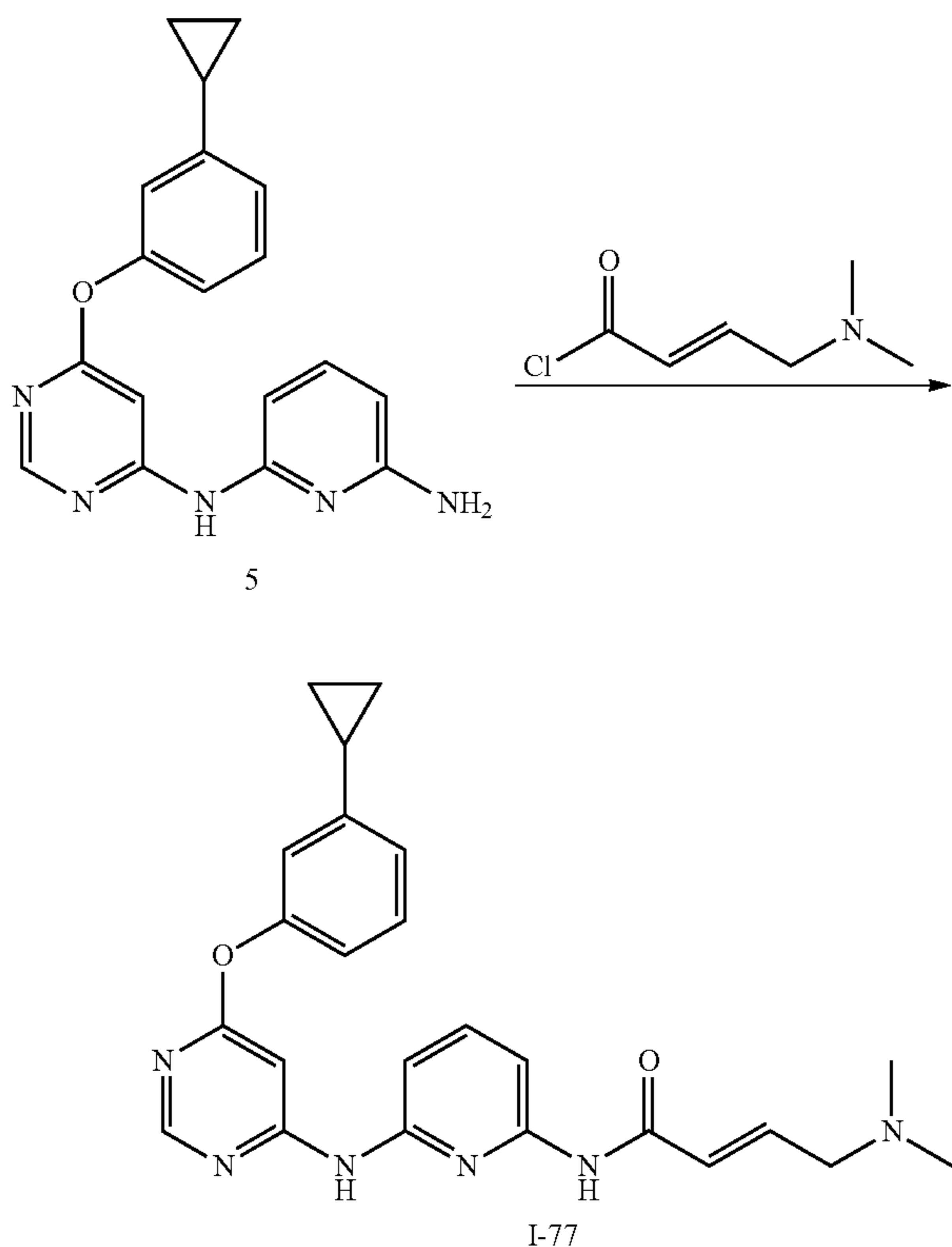
SCHEME 20a
