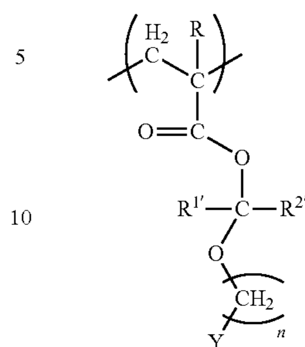
(a1-0-1)
