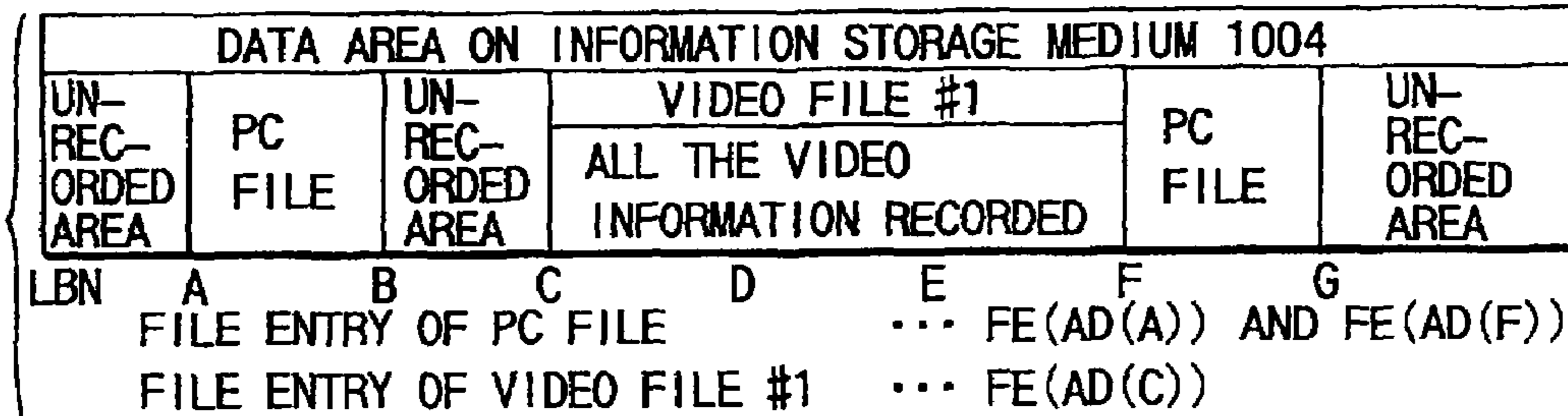
FIG. 19A
