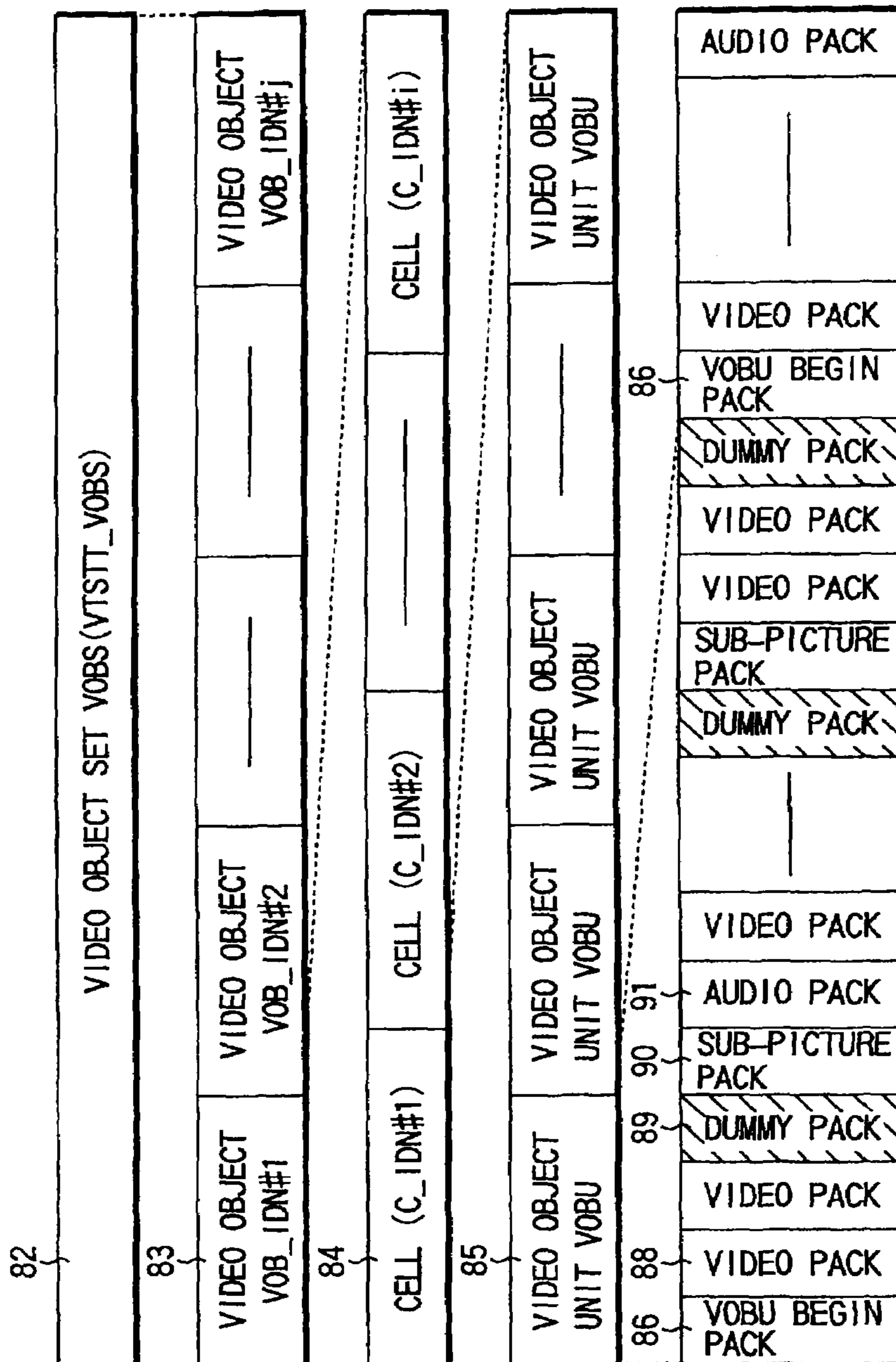
FIG. 7
