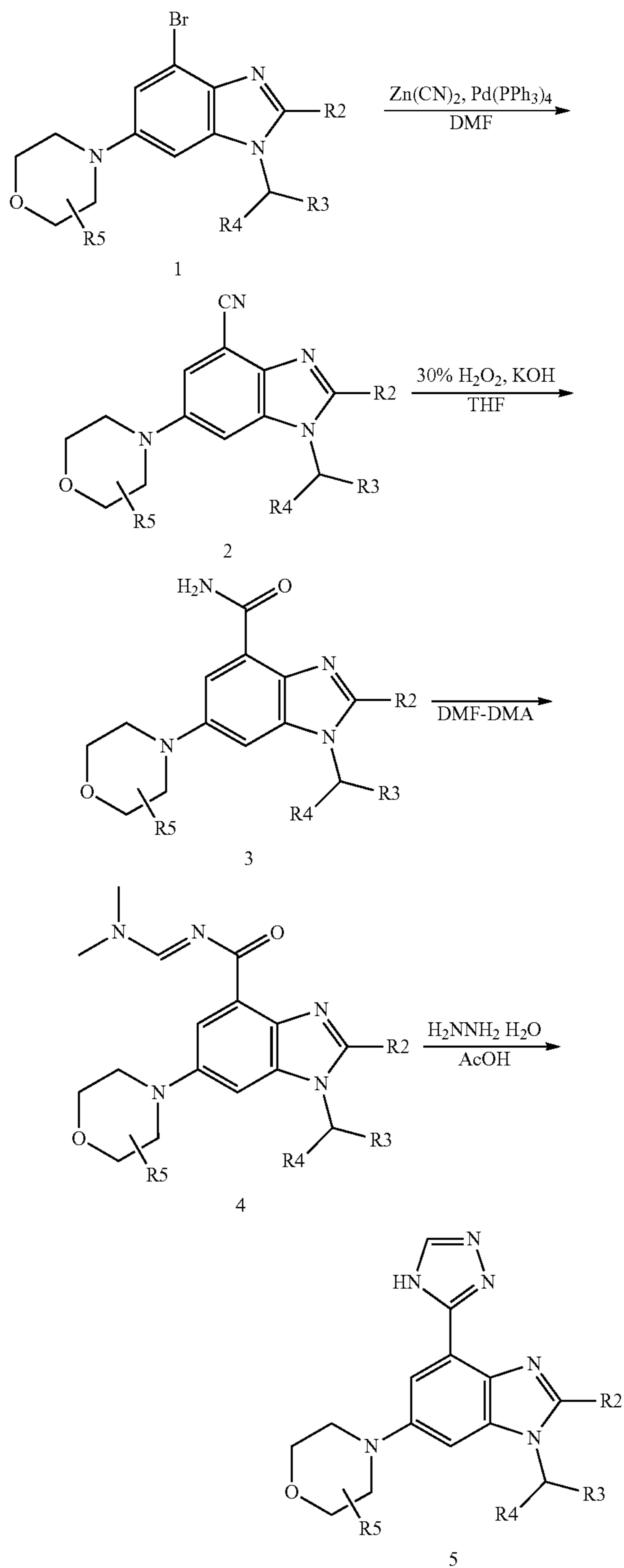
Scheme VI
