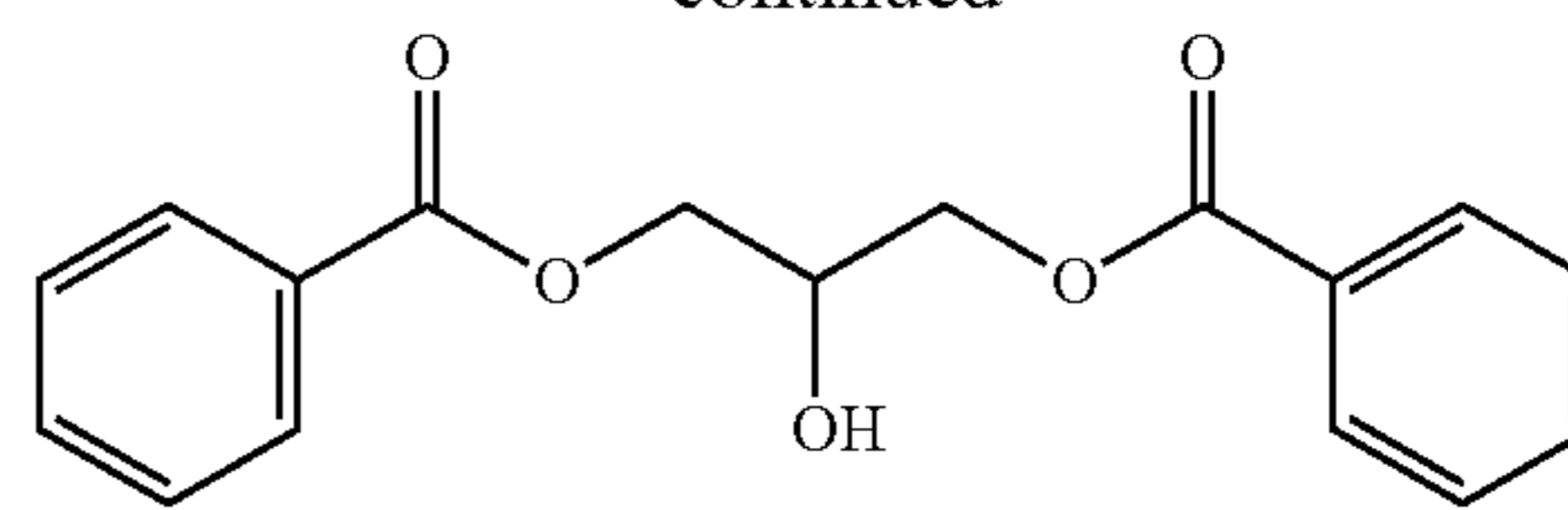
Glycerol Di-Benzoate
