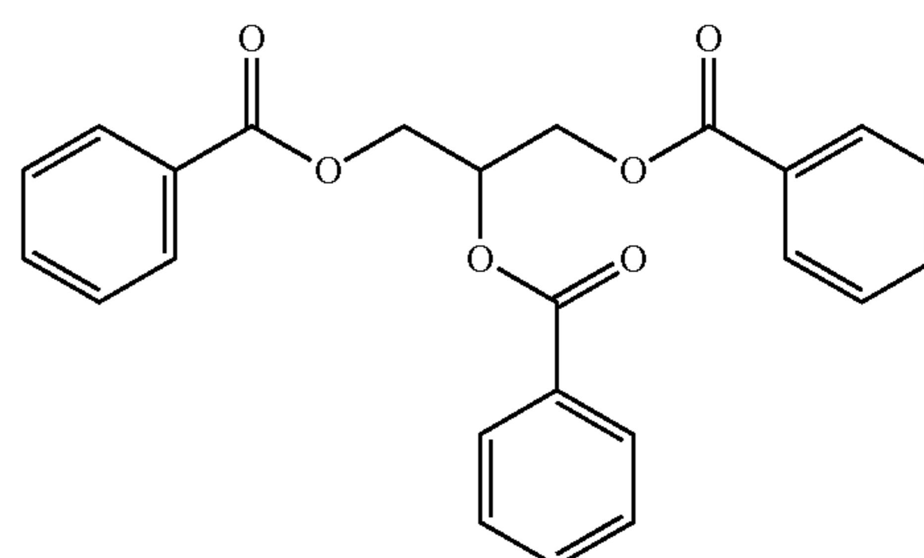
Glycerol Tri-Benzoate
