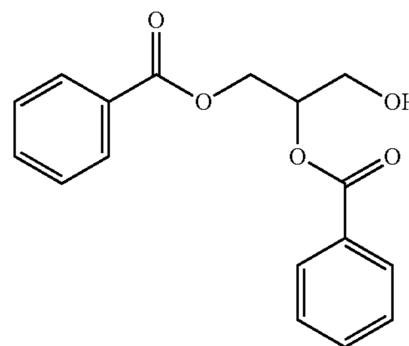
Glycerol Di-Benzoate
