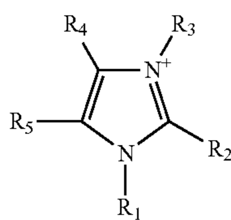
imidazolium
