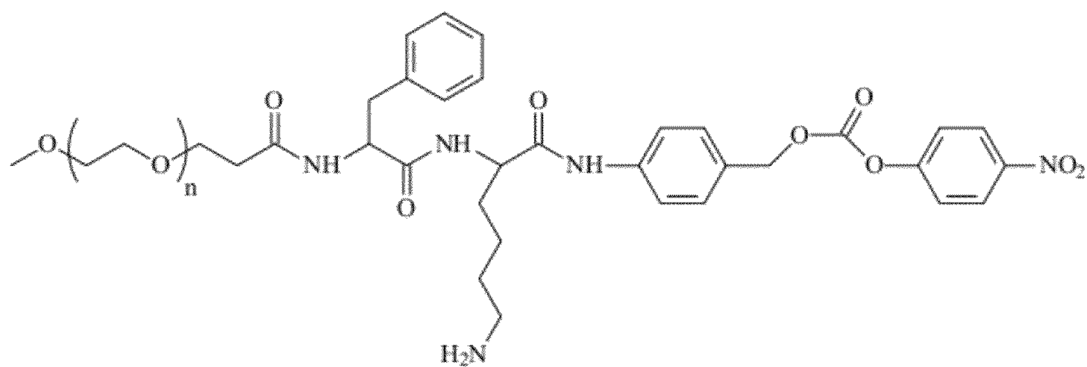
PEG-PheLys-PABC-PNP
