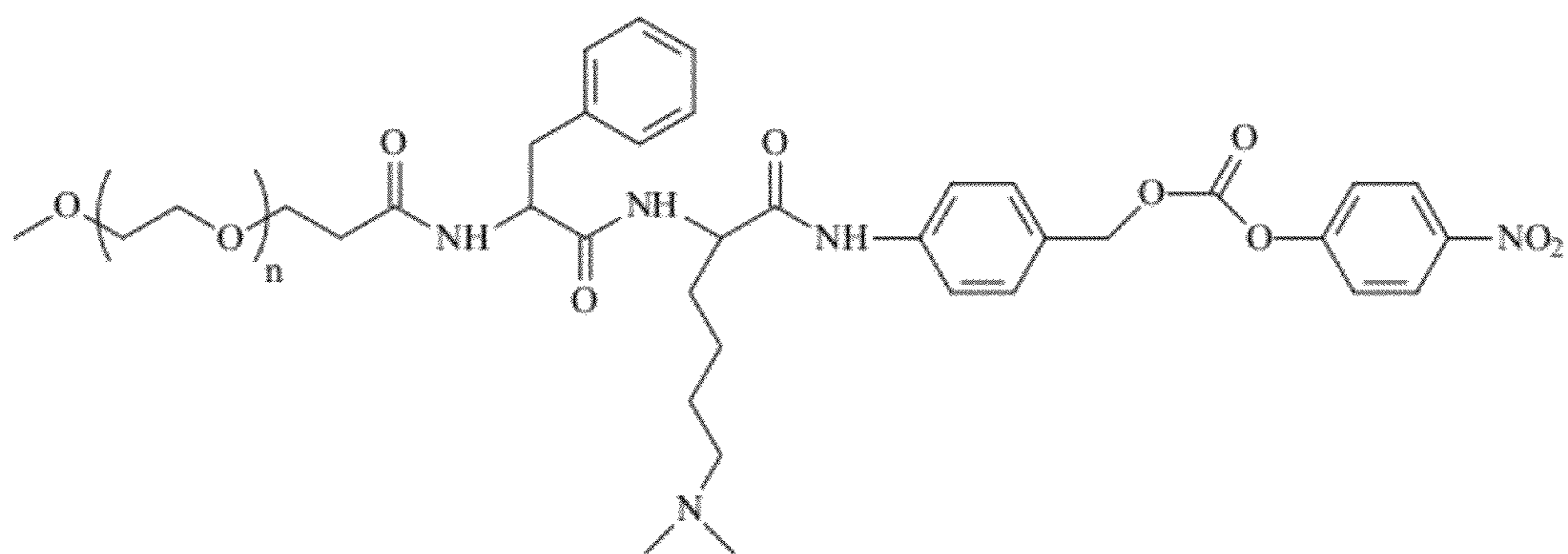
PEG-PheLys(CH 3 ) 2 -PABC-PNP
