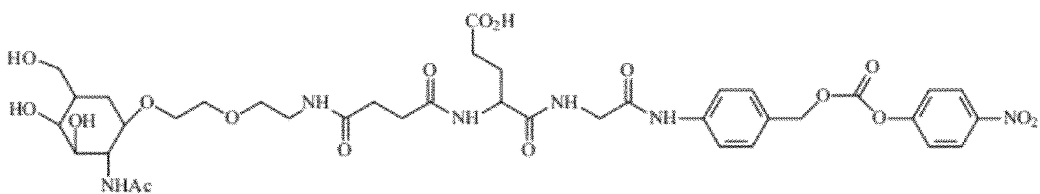
NAG-GluGly-PABC-PNP
