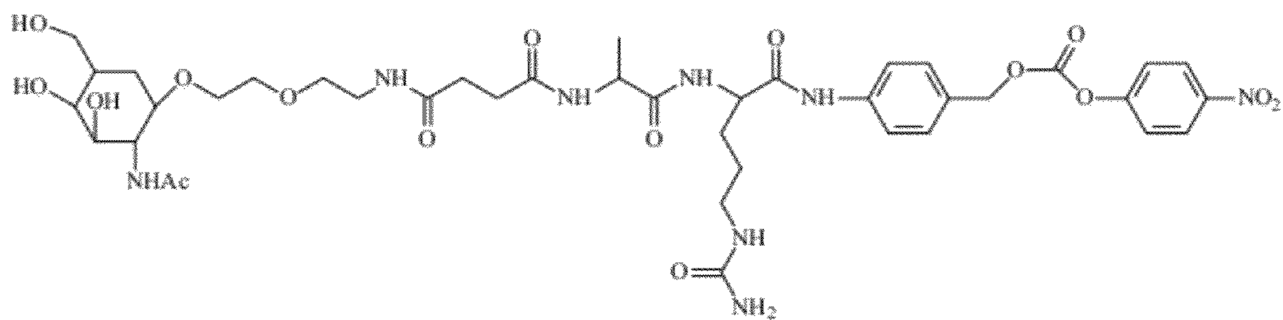
NAG-AlaCit-PABC-PNP
