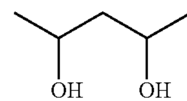
2,4-Pentanediol
