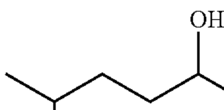
1,5-Hexanediol
