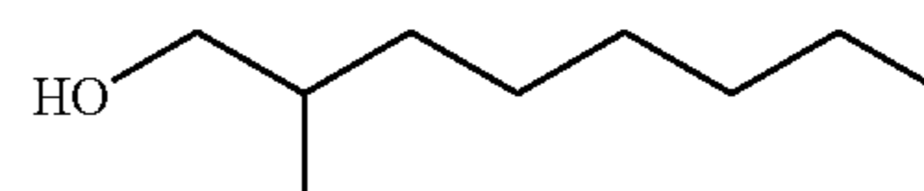
1,2-Octanediol
