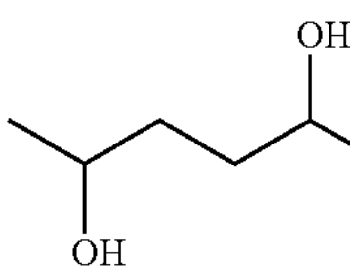
2,5-Hexanediol
