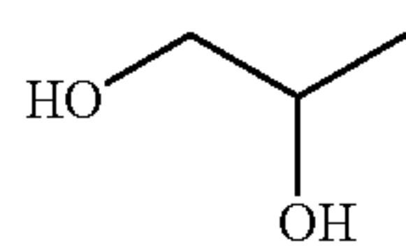
1,2-Propanediol
