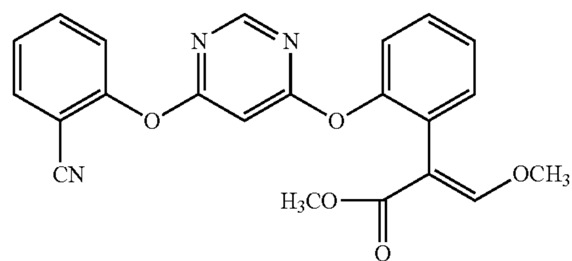
(azoxystrobin)
