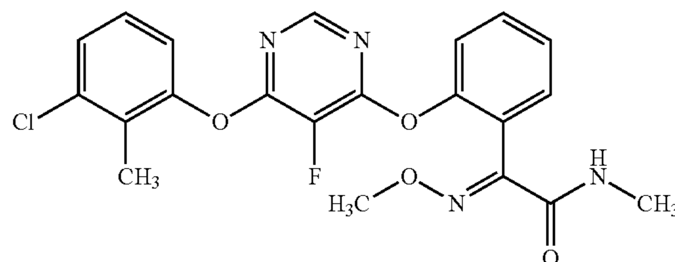
(metominostrobin)
