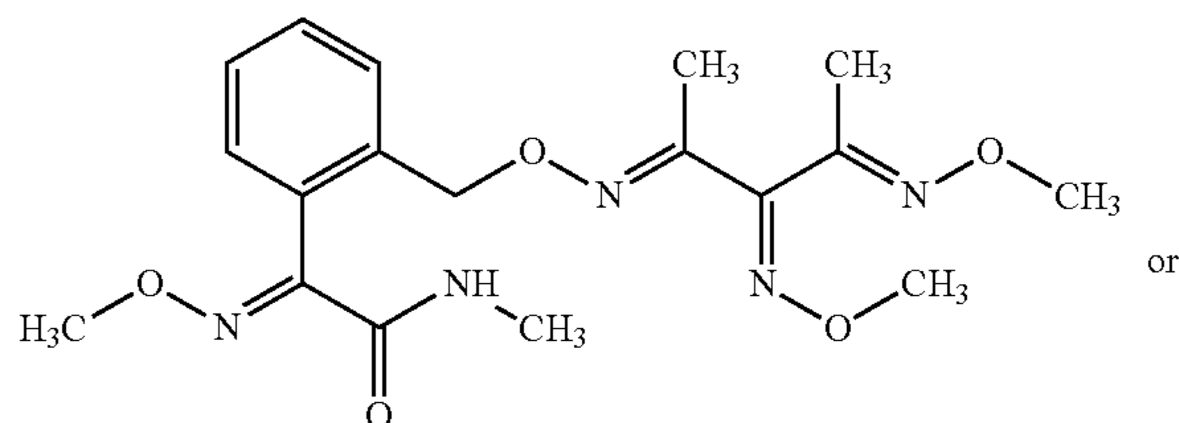
(orysastrobin)
