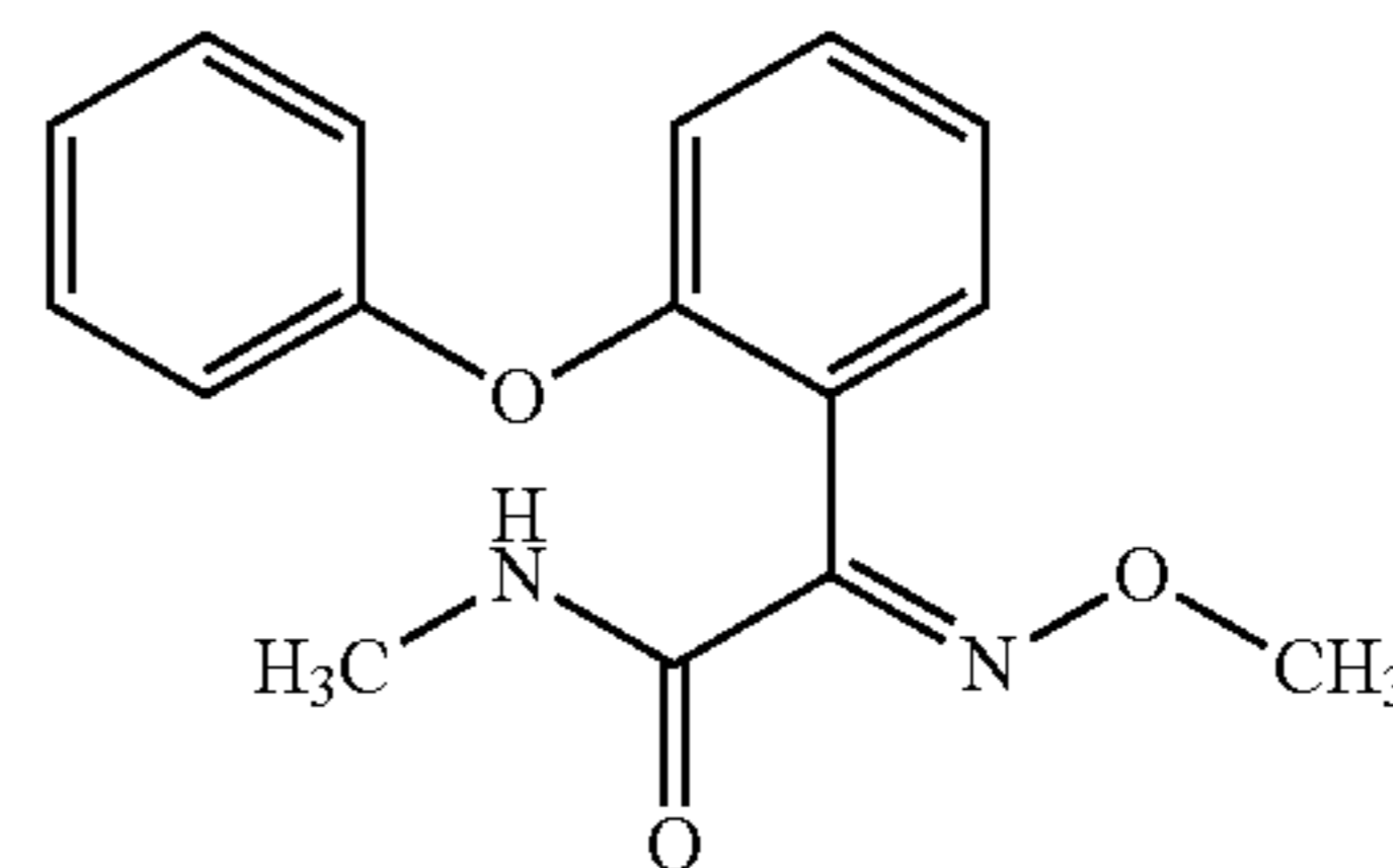
(metominostrobin)
