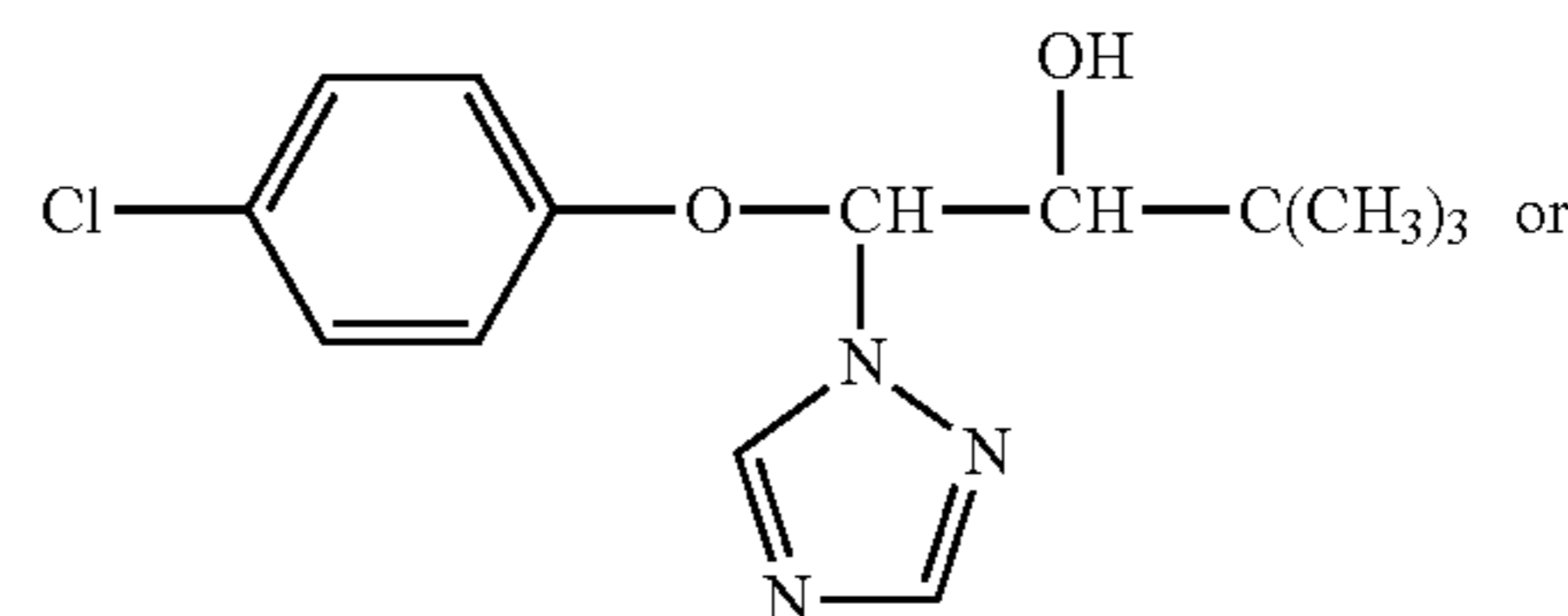
(triadimenol)
