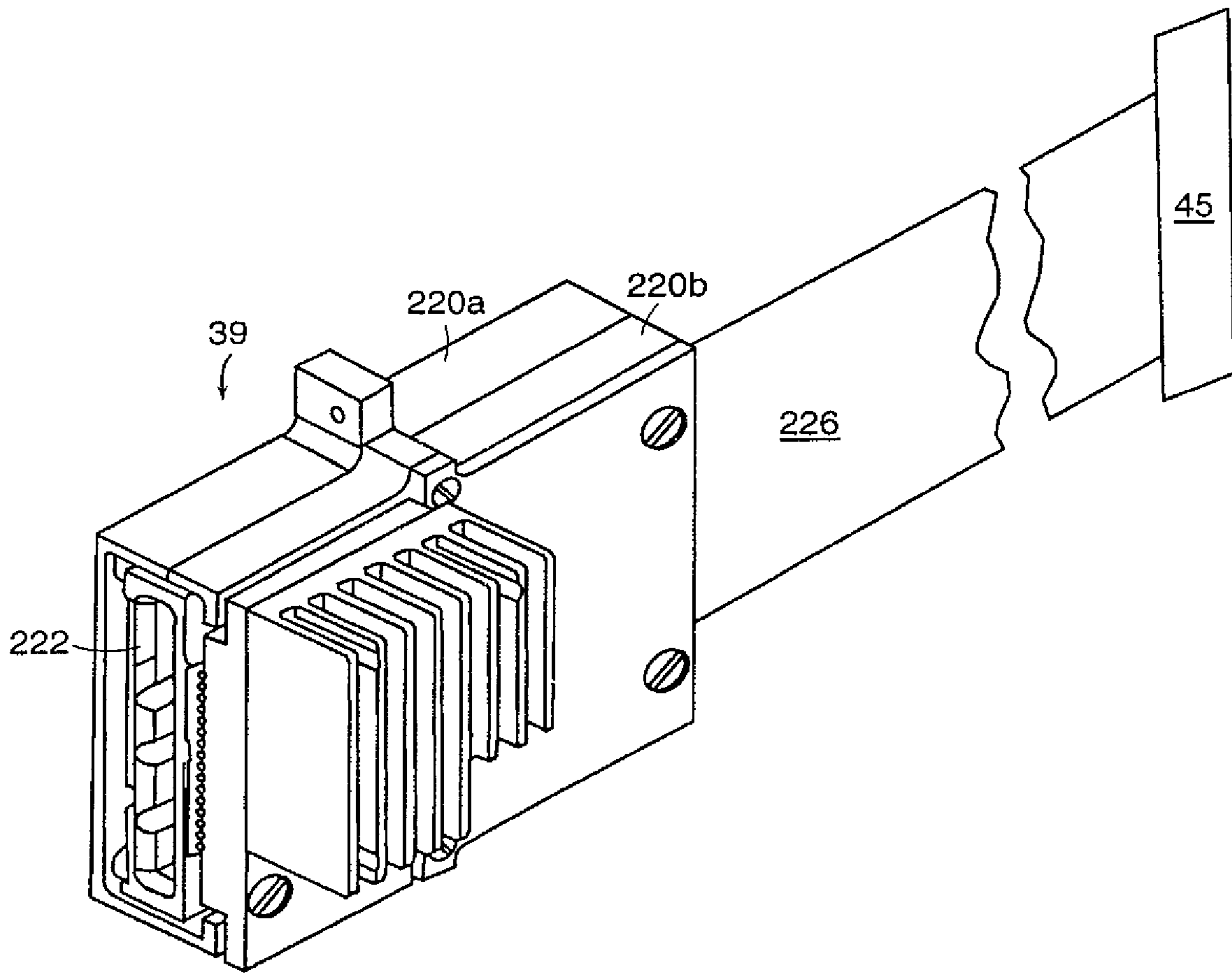
FIG. 7A
