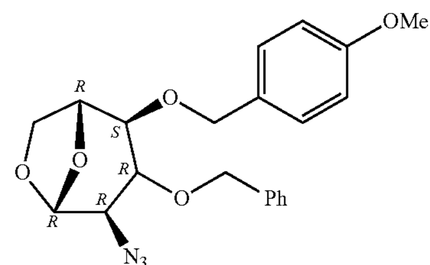
Monomer A-2 IntA5
