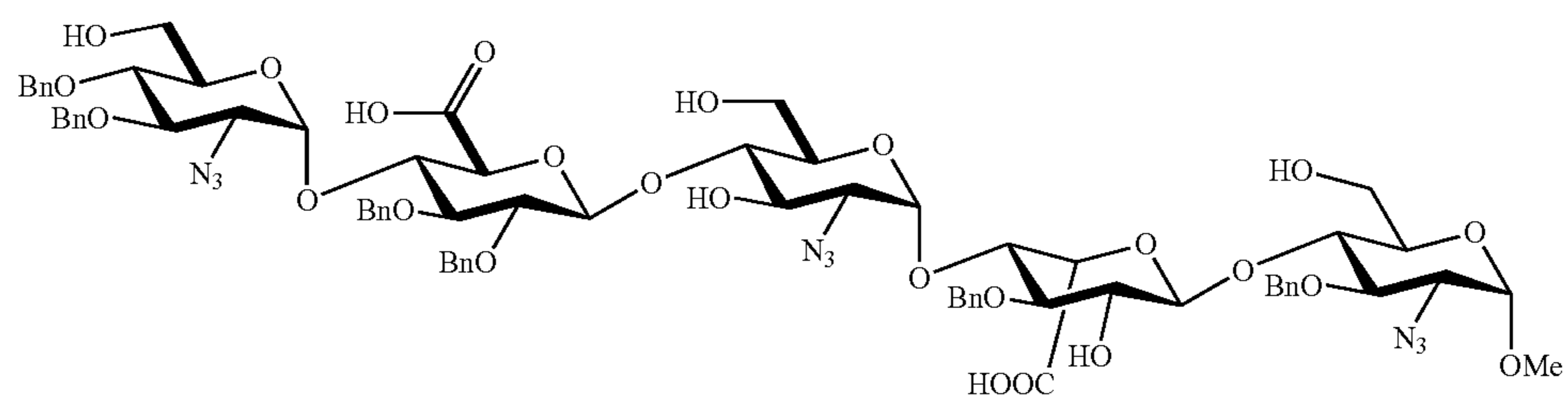
API-1-CB C_{73}H_{83}N_9O_{25} Mol. Wt.: 1486.49
