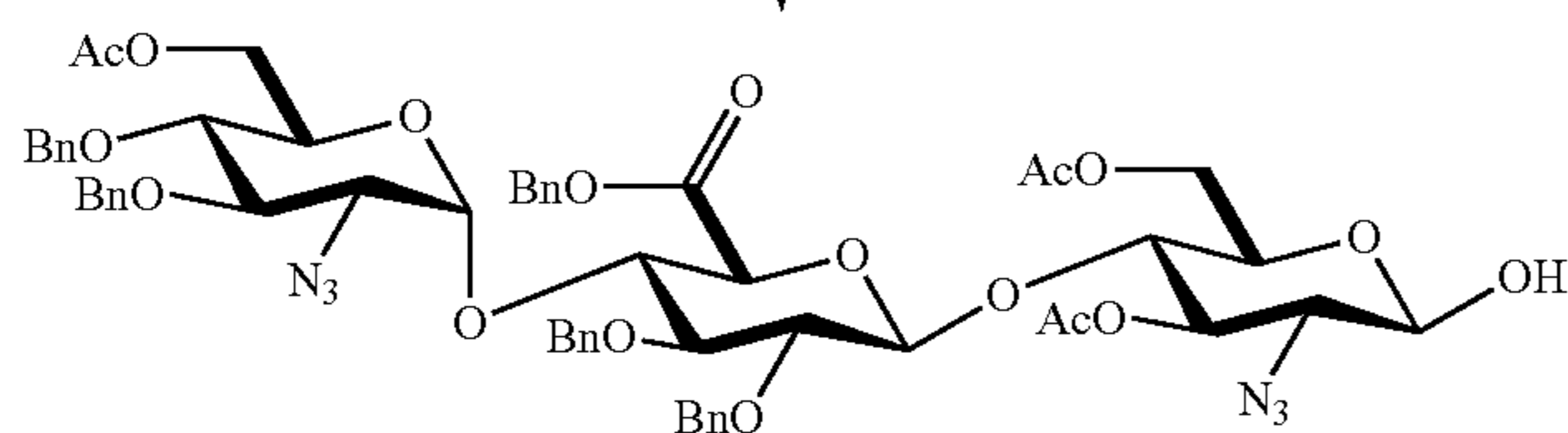
EDC-2-CB C_{57}H_{64}N_6O_{20} Mol. Wt.: 1153.15
