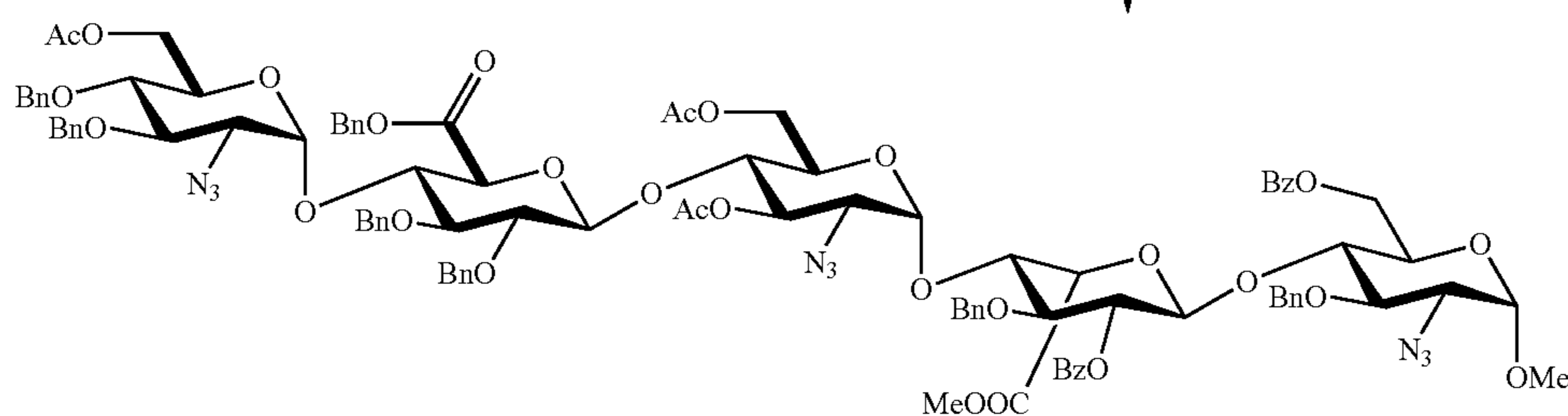
EDCBA Pentamer-CB C_{101}H_{105}N_9O_{30} Mol. Wt.: 1924.96
