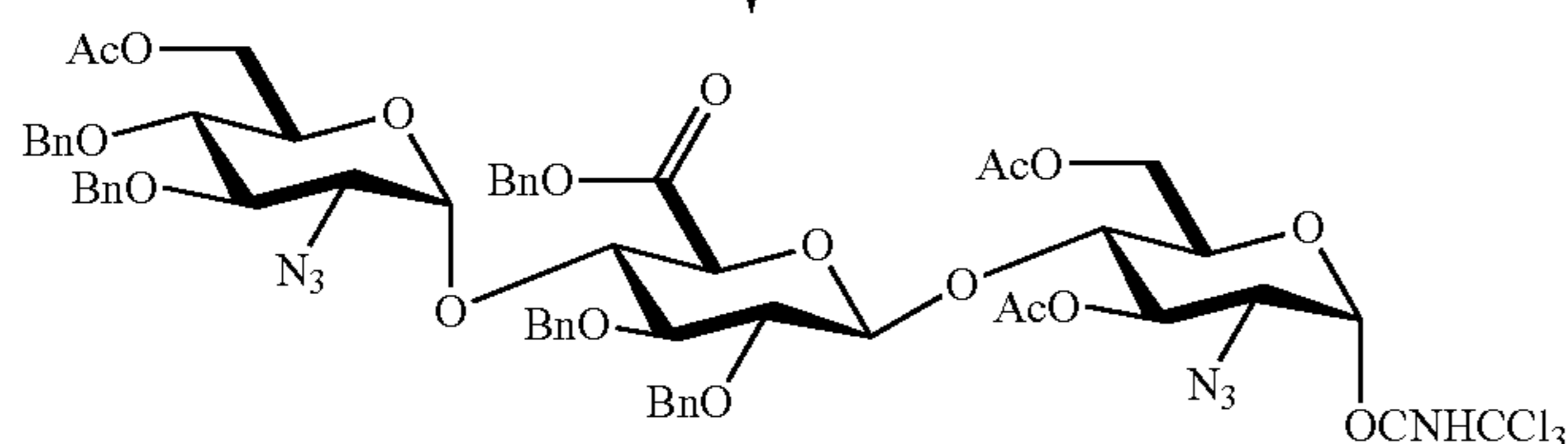
EDC-3-CB C_{61}H_{64}Cl_3N_7O_{18} Mol. Wt.: 1289.56
