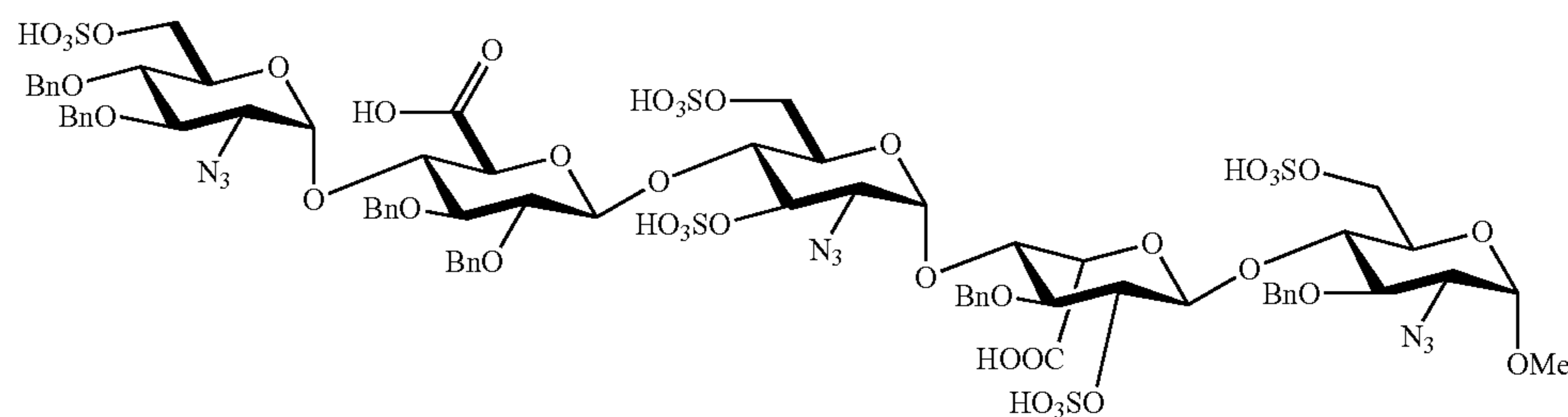
API-2-CB C_{73}H_{83}N_9O_{40}S_5 Mol. Wt.: 1886.81
