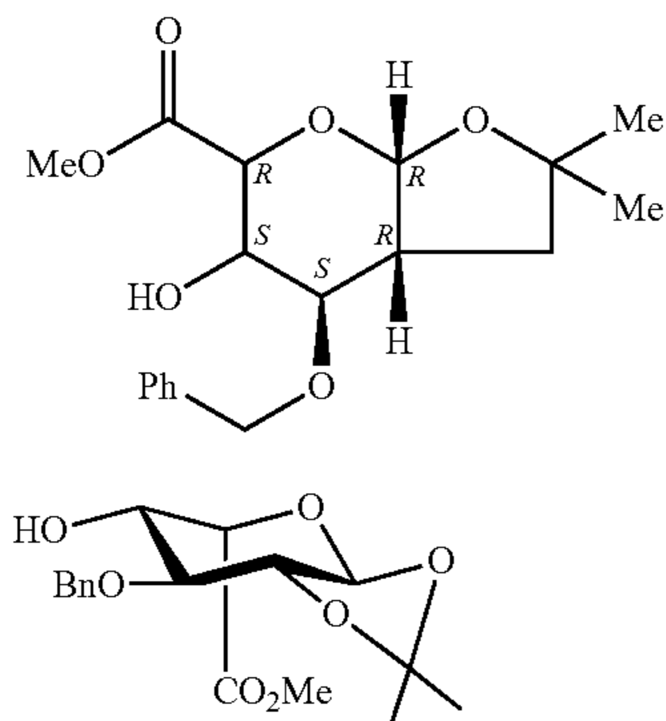
Monomer B-1
