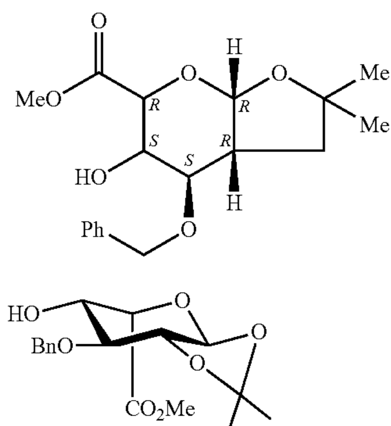
Monomer B-1
