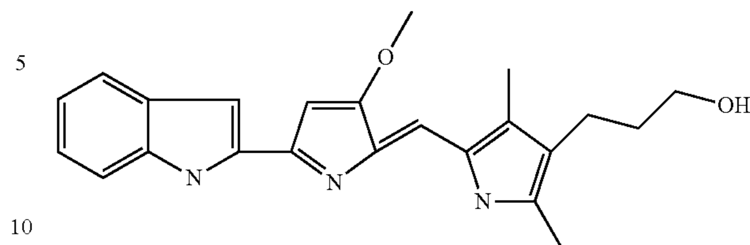
3-{5-[5-(1H-indol-2-yl)-3-methoxy-pyrrol-2-ylidenemethyl]-2,4-dimethyl-1H-pyrrol-3-yl}-propan-1-ol
