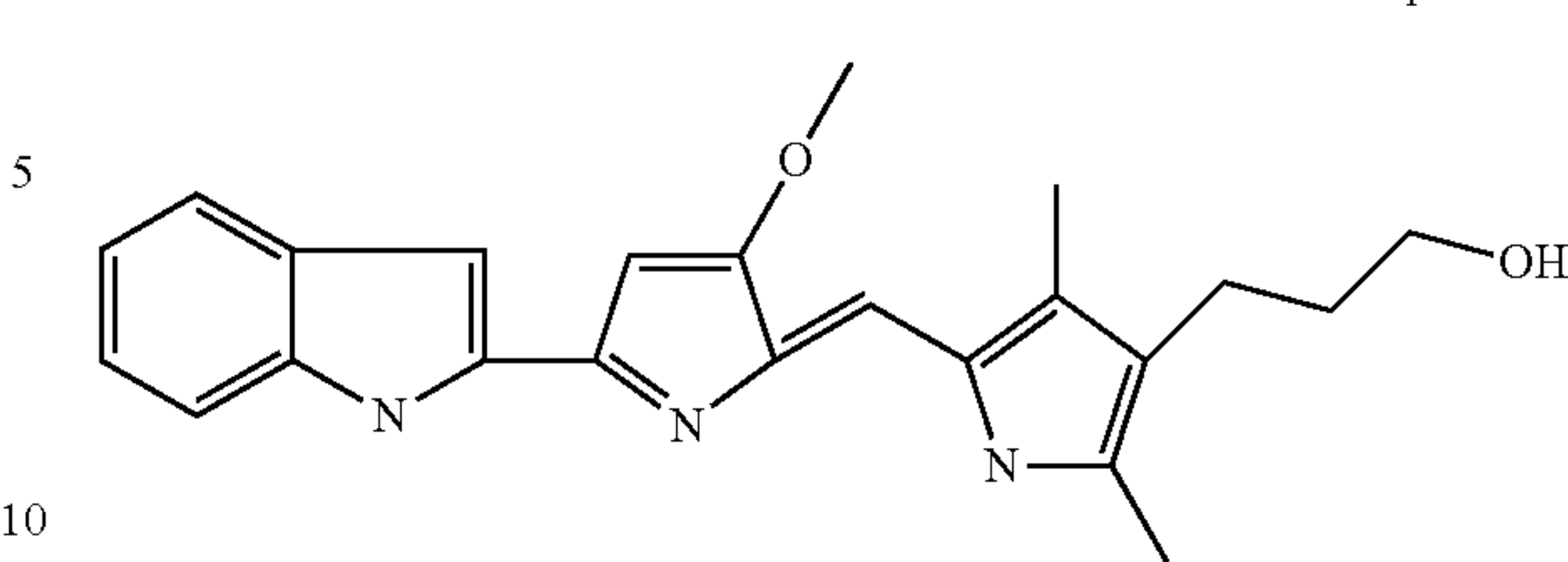
3-{5-[5-(1H-indol-2-yl)-3-methoxy-pyrrol-2-ylidenemethyl]-2,4-dimethyl-1H-pyrrol-3-yl}-propan-1-ol
