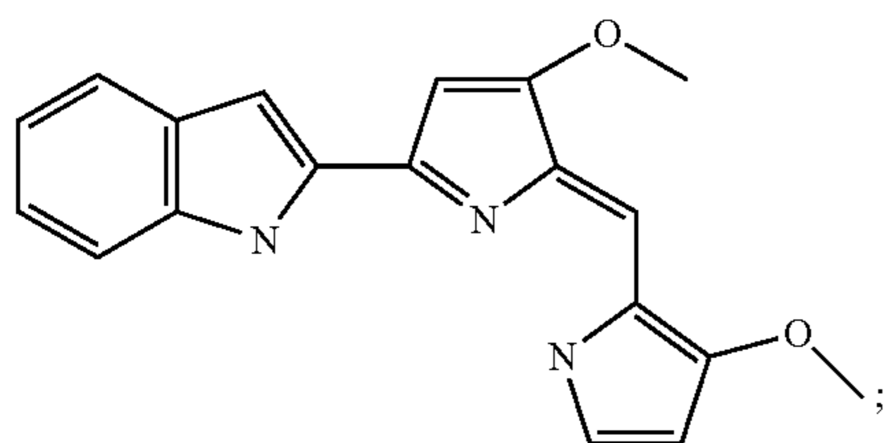
2-[4-Methoxy-5-(3-methoxy-1H-pyrrol-2-ylmethylene)-5H-pyrrol-2-yl]-1H-indole
