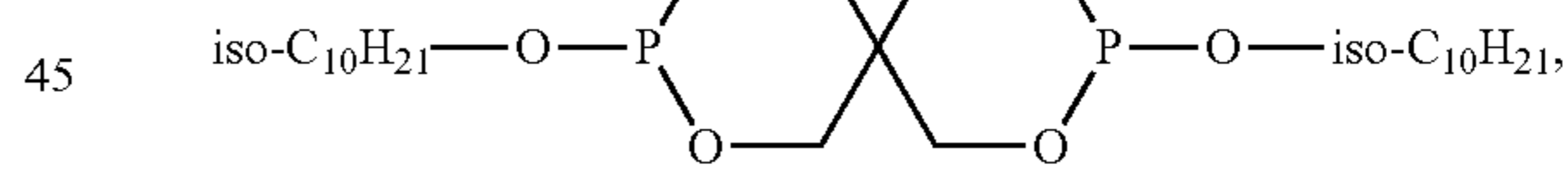
[CAS RN 26544-27-4]
