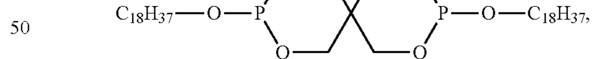
[CAS RN 3806-34-6]
