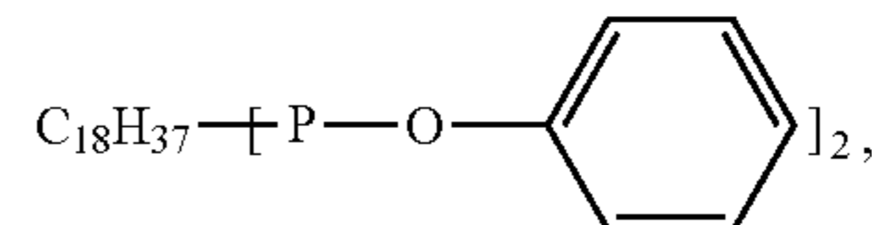
[CAS RN 2082-80-6]
