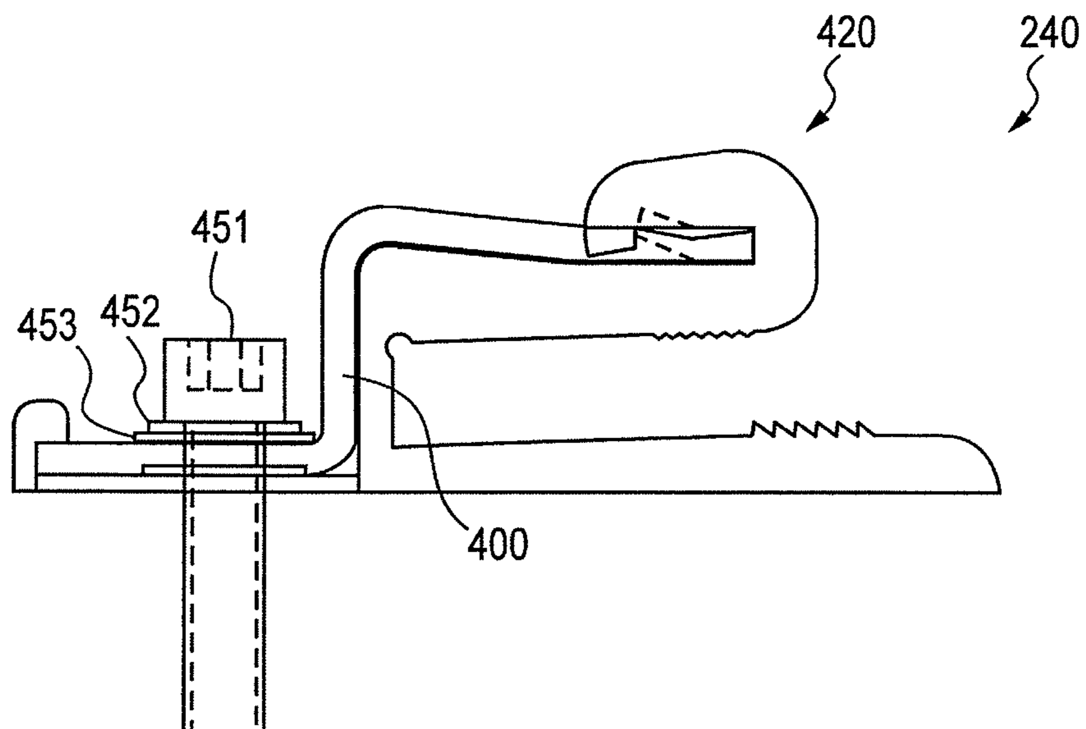
FIG. 4B
