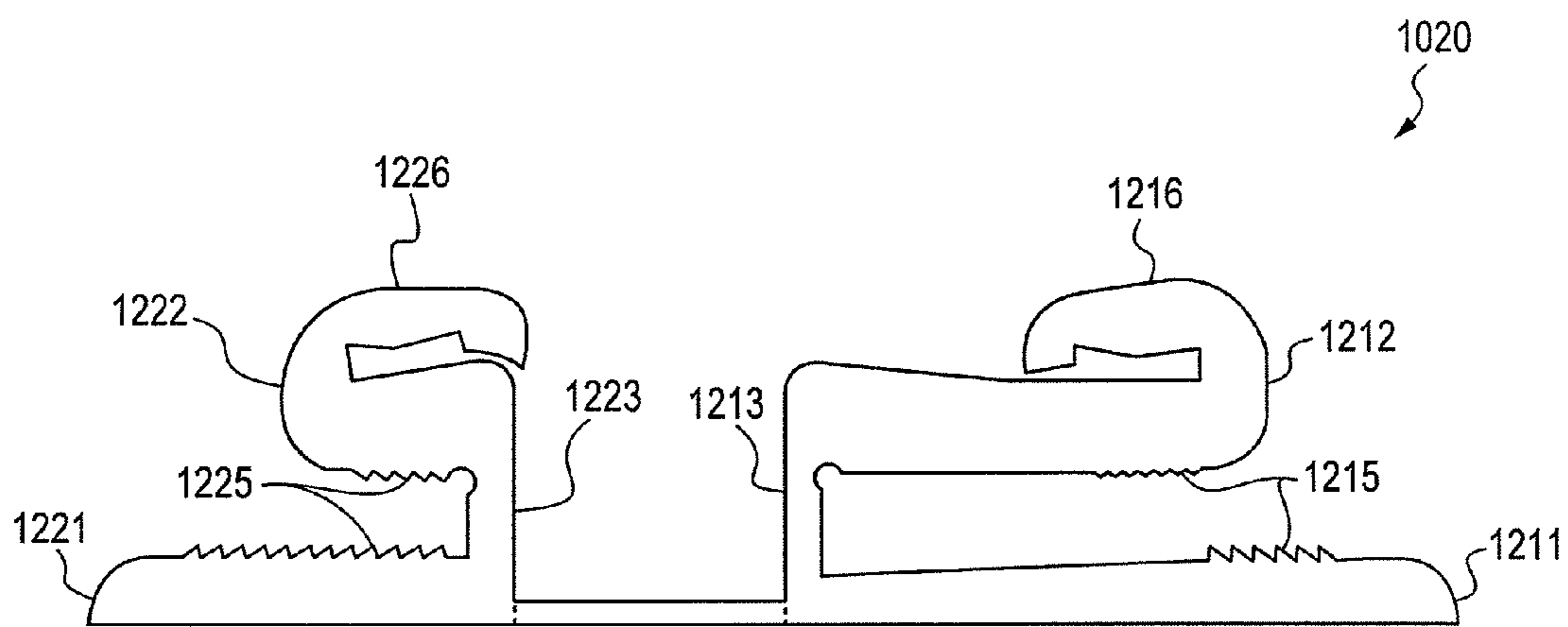
FIG. 12B
