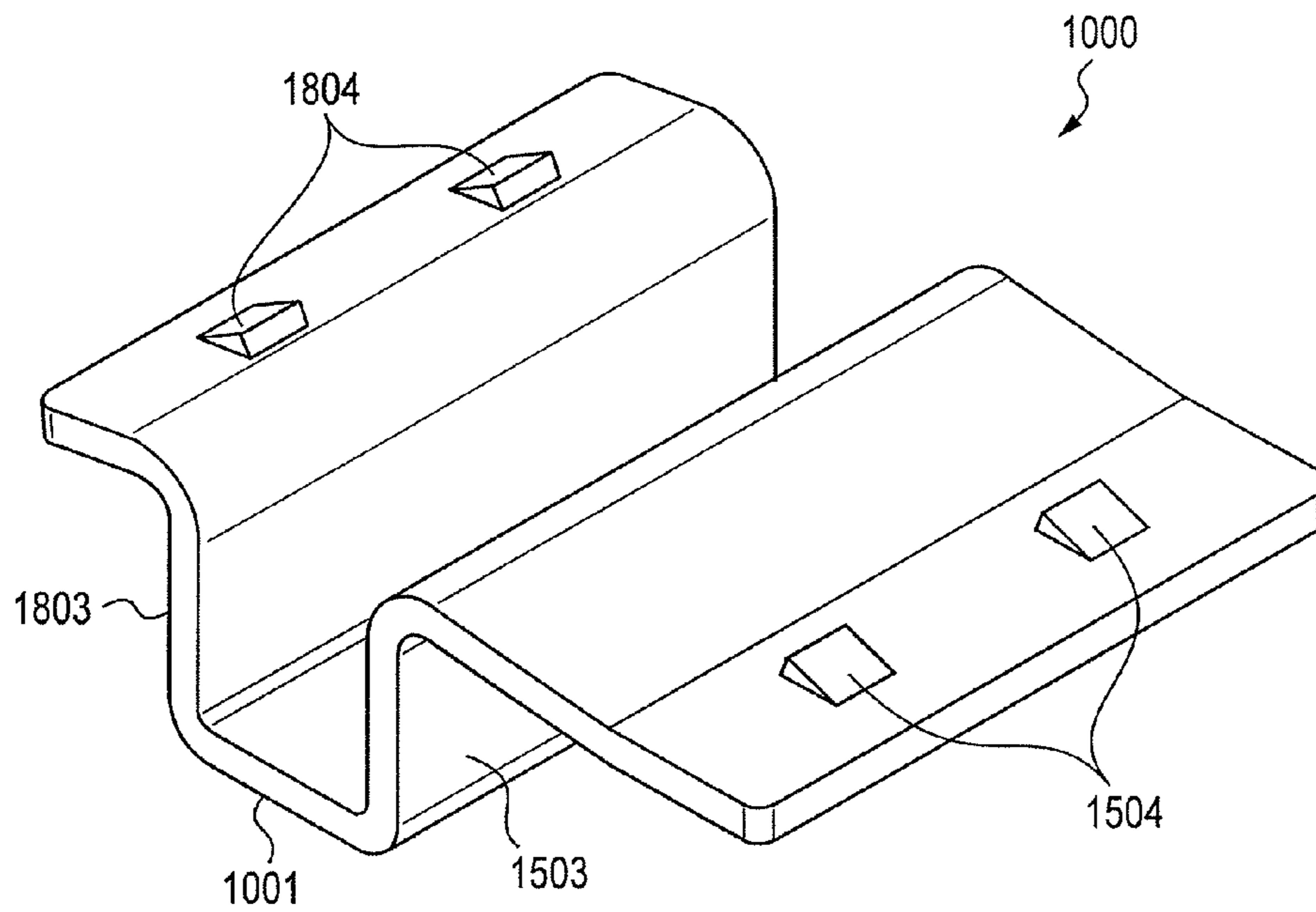
FIG. 11A
