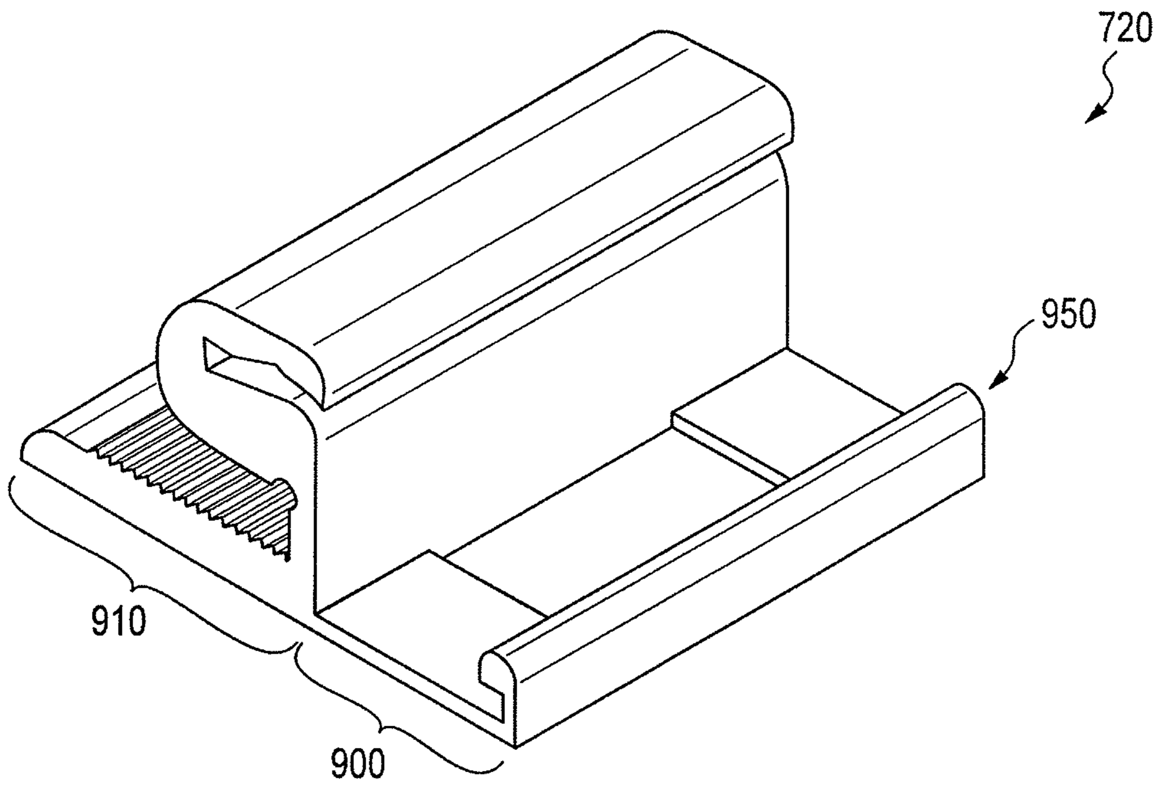
FIG. 9A
