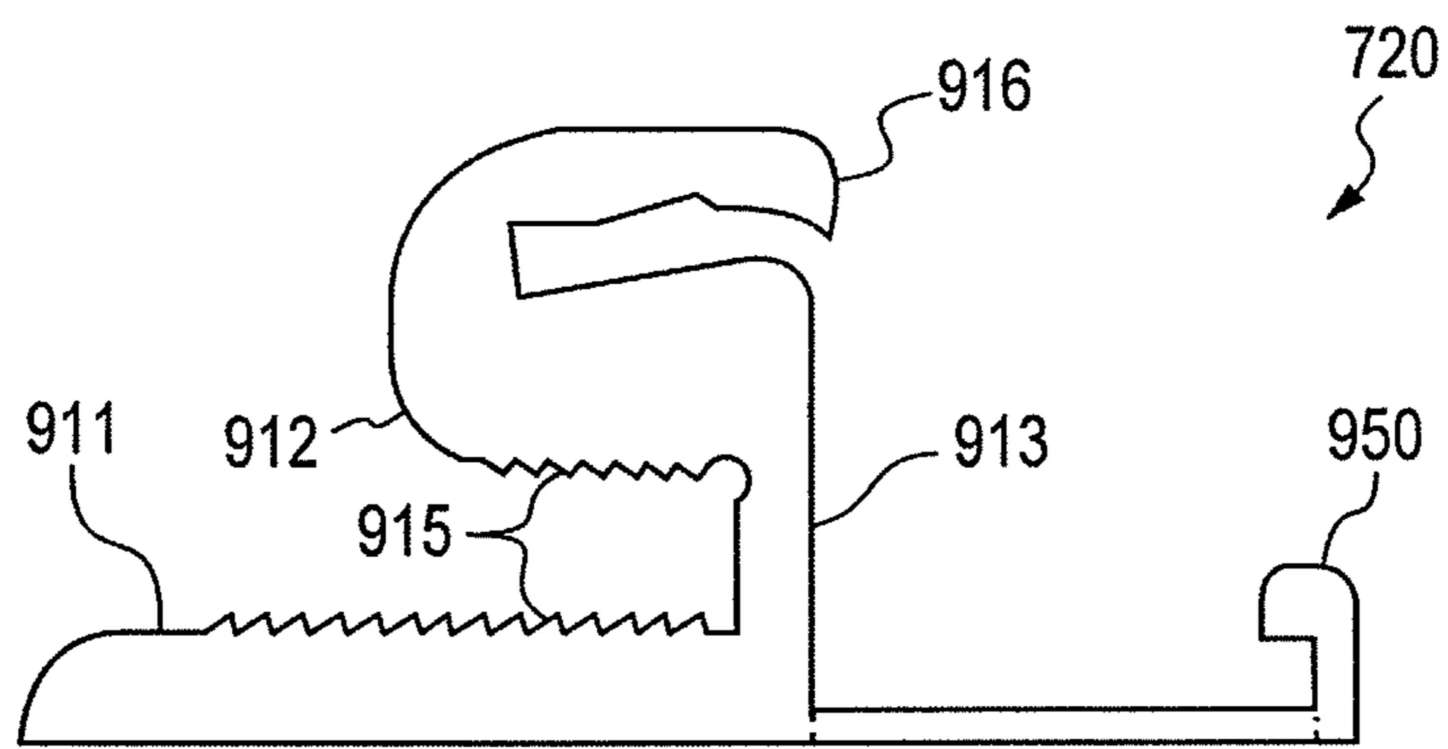
FIG. 9B
