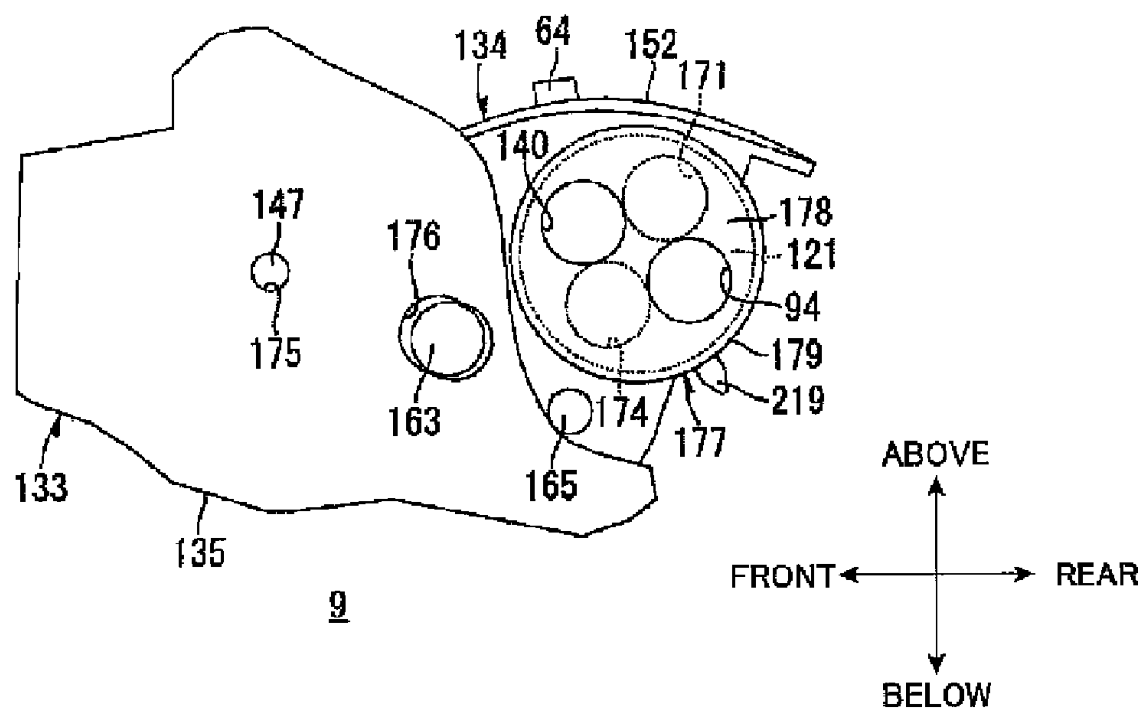
FIG.18B
