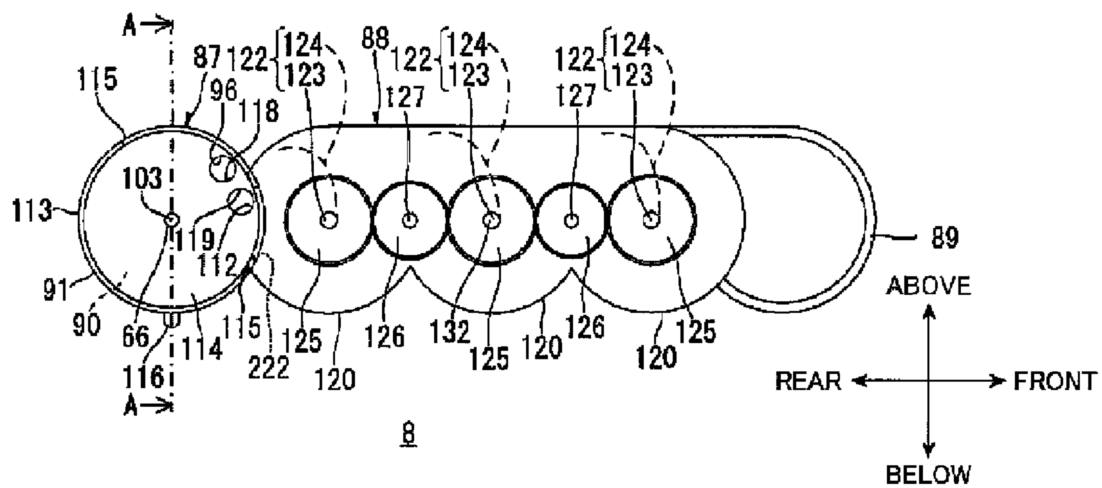
FIG. 14B
