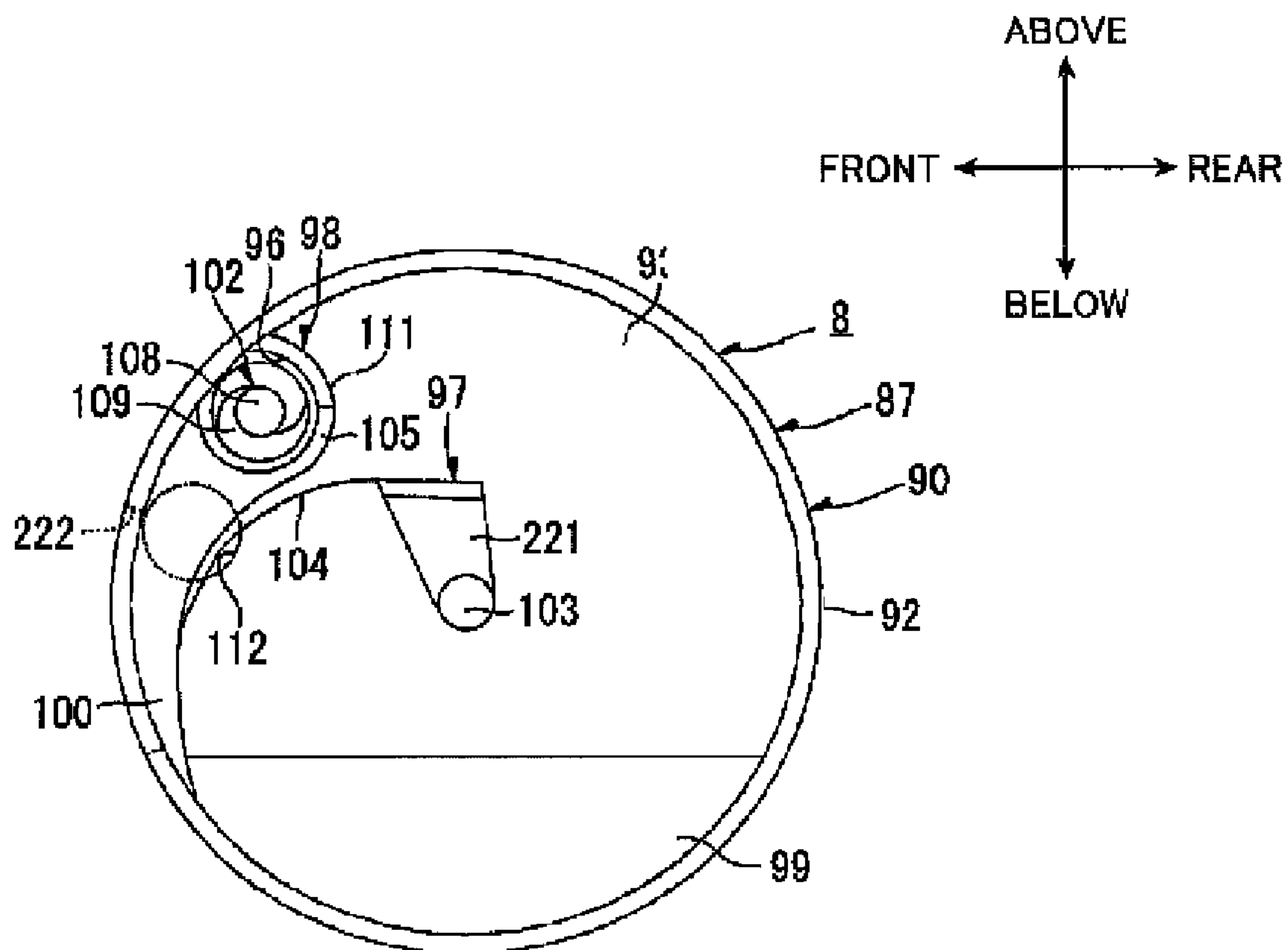
FIG. 16
