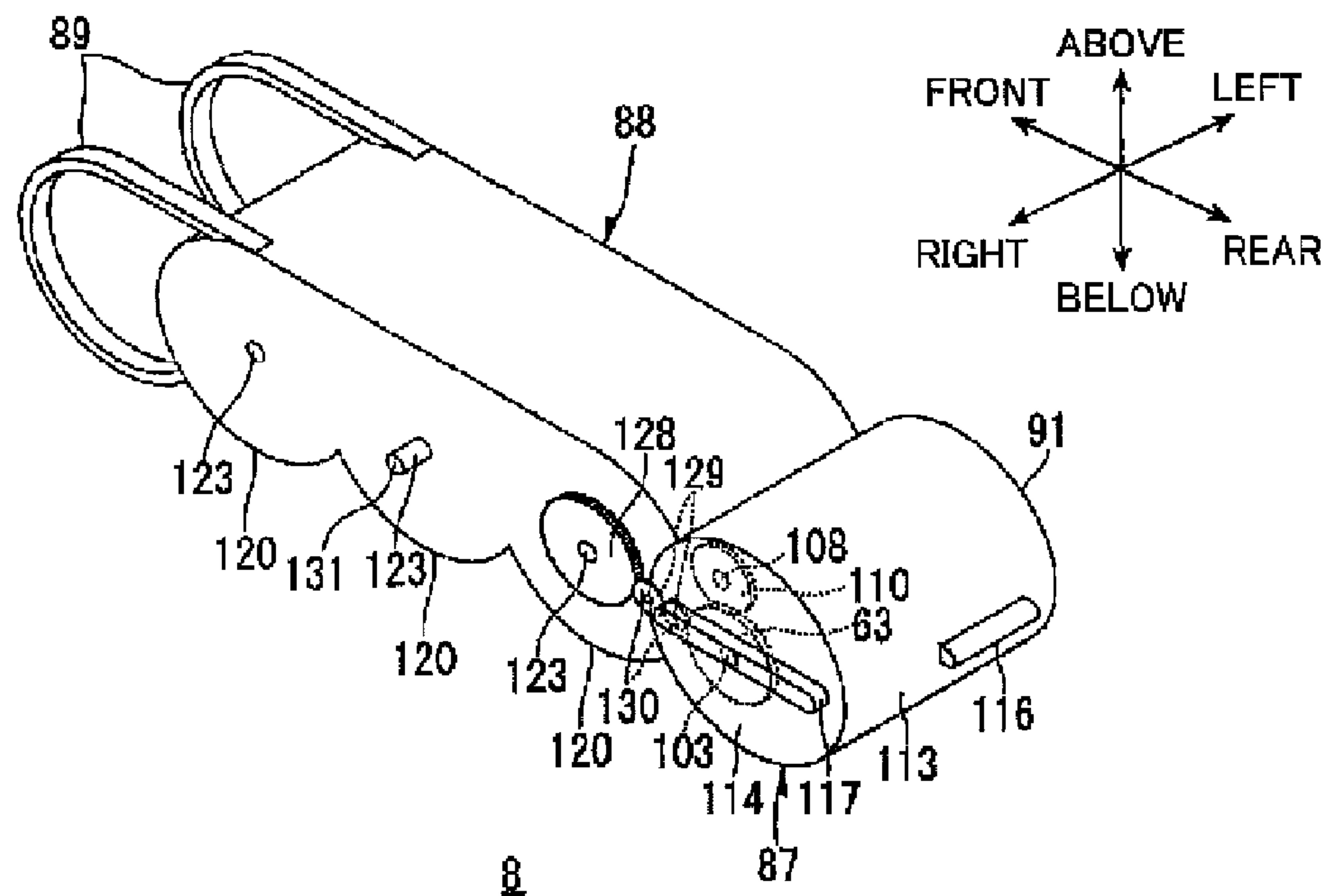
FIG. 11B
