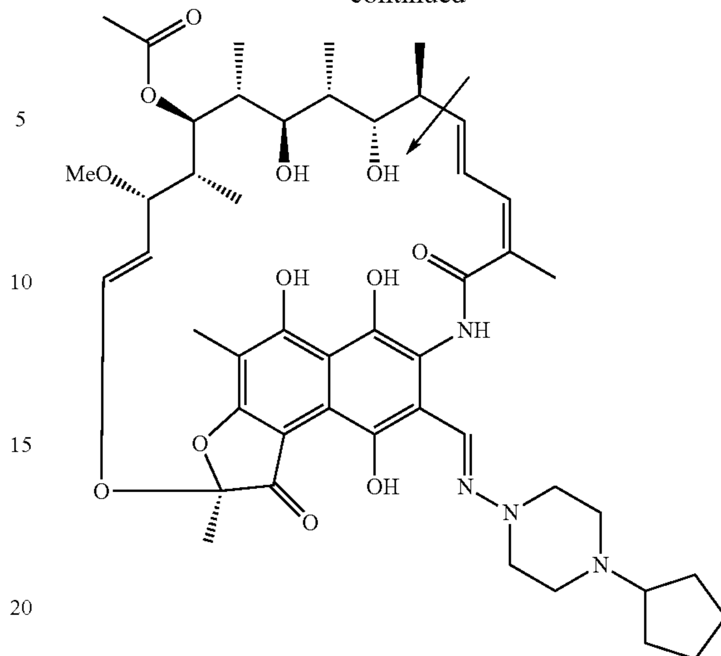
Rifapentin
