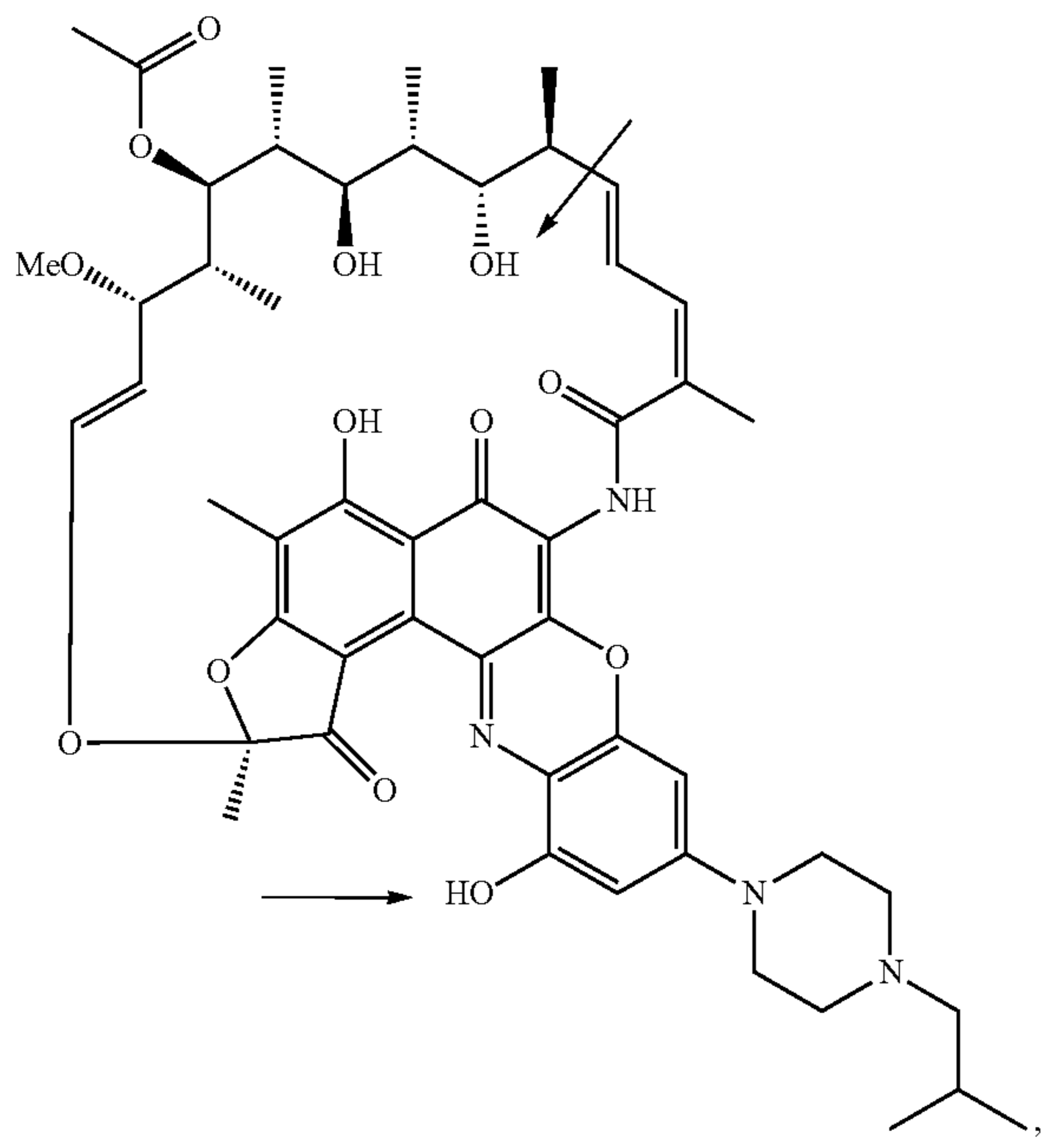
Rifalazil
