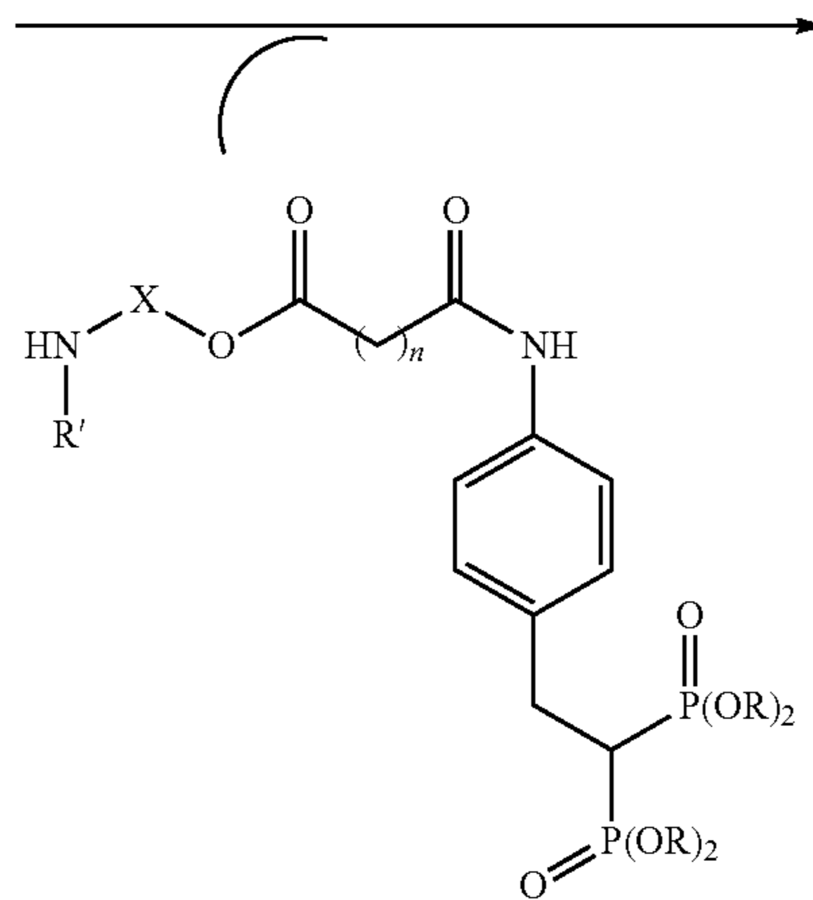
XXXc n = 2 XXXd n = 3
