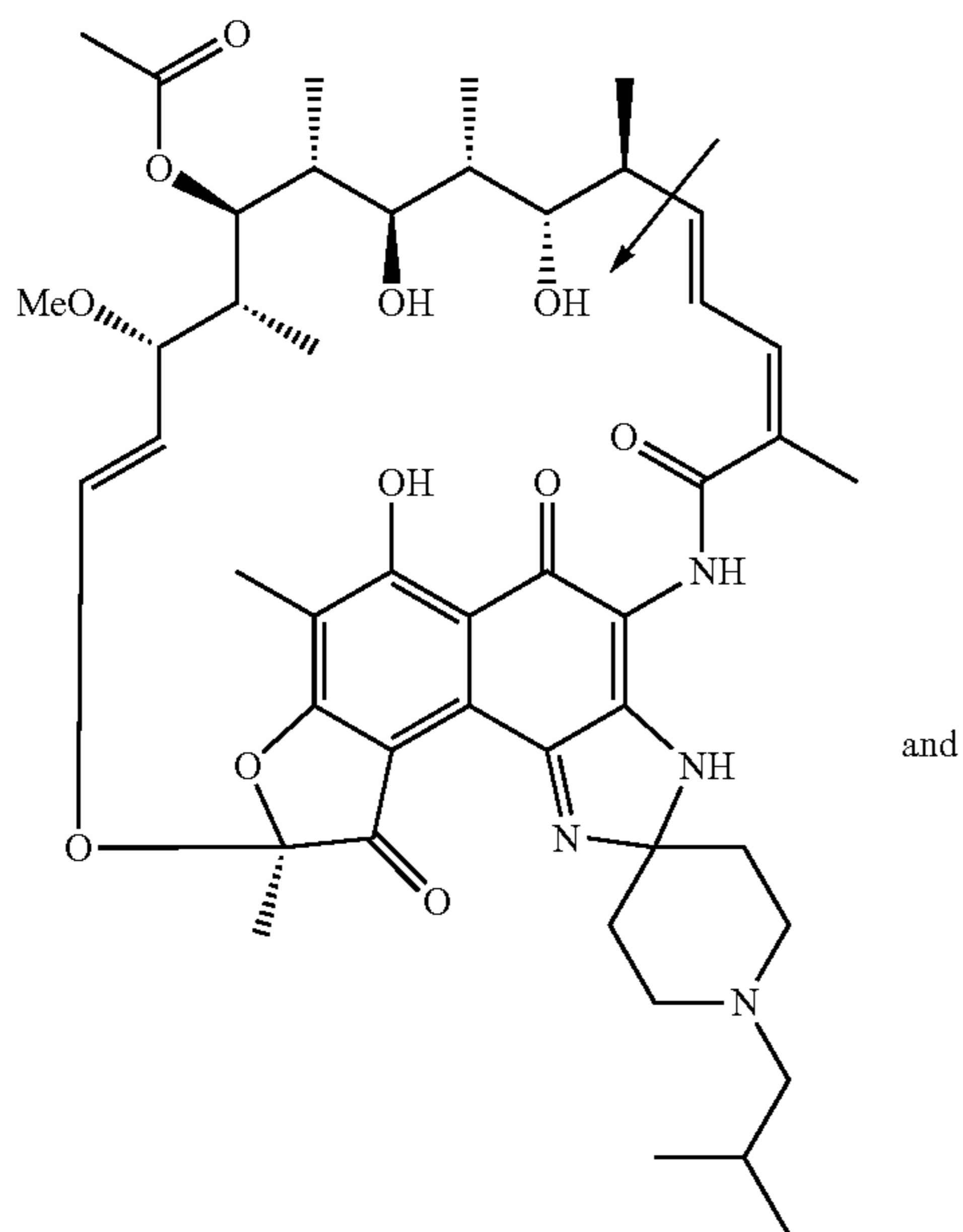
Rifabutin
