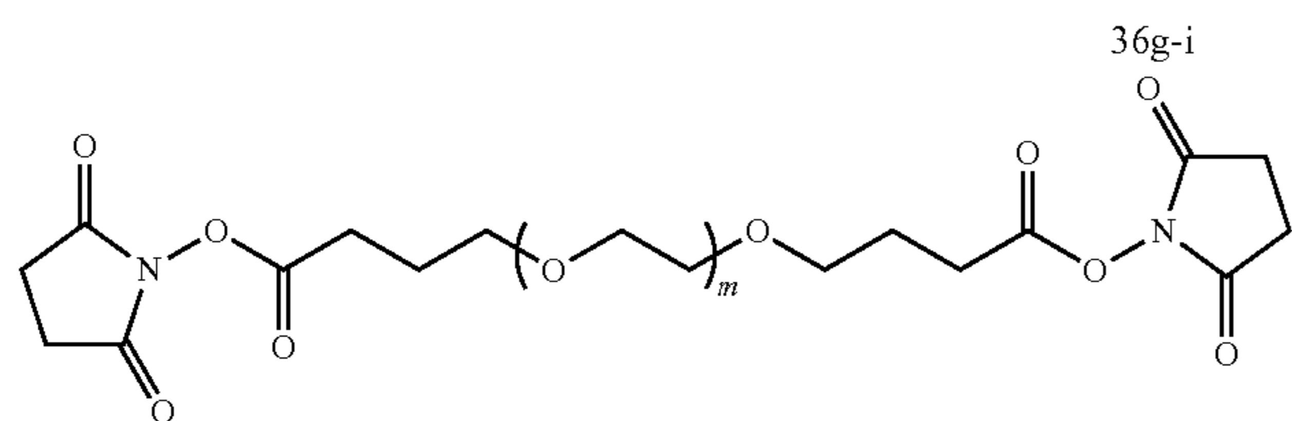
PEG-DiSBA (MW = 3400 Da)
