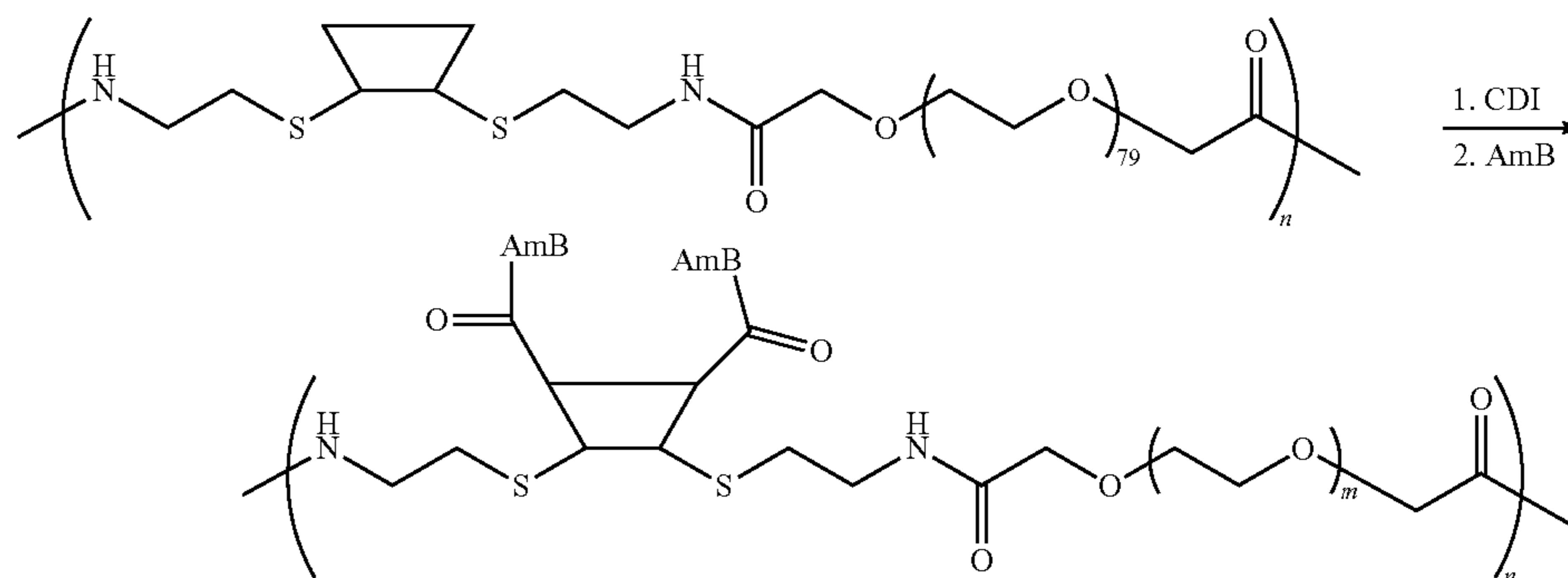
Scheme LII
