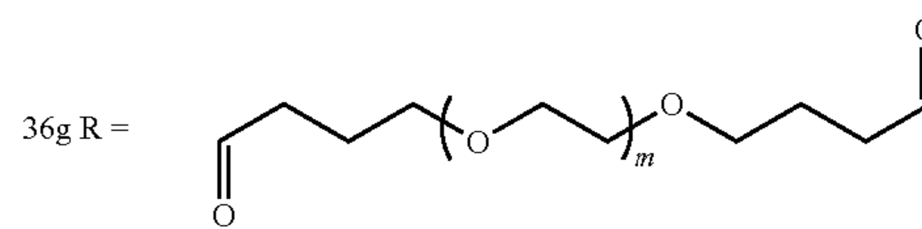
Poly(CDDCys-BA-PEG)
