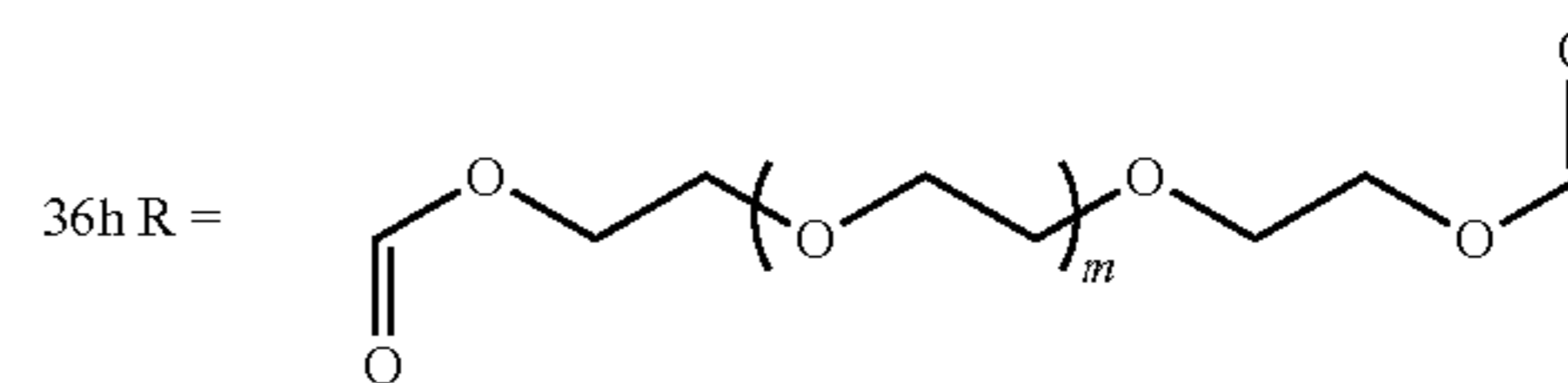
Poly(CDDCys-CB-PEG)
