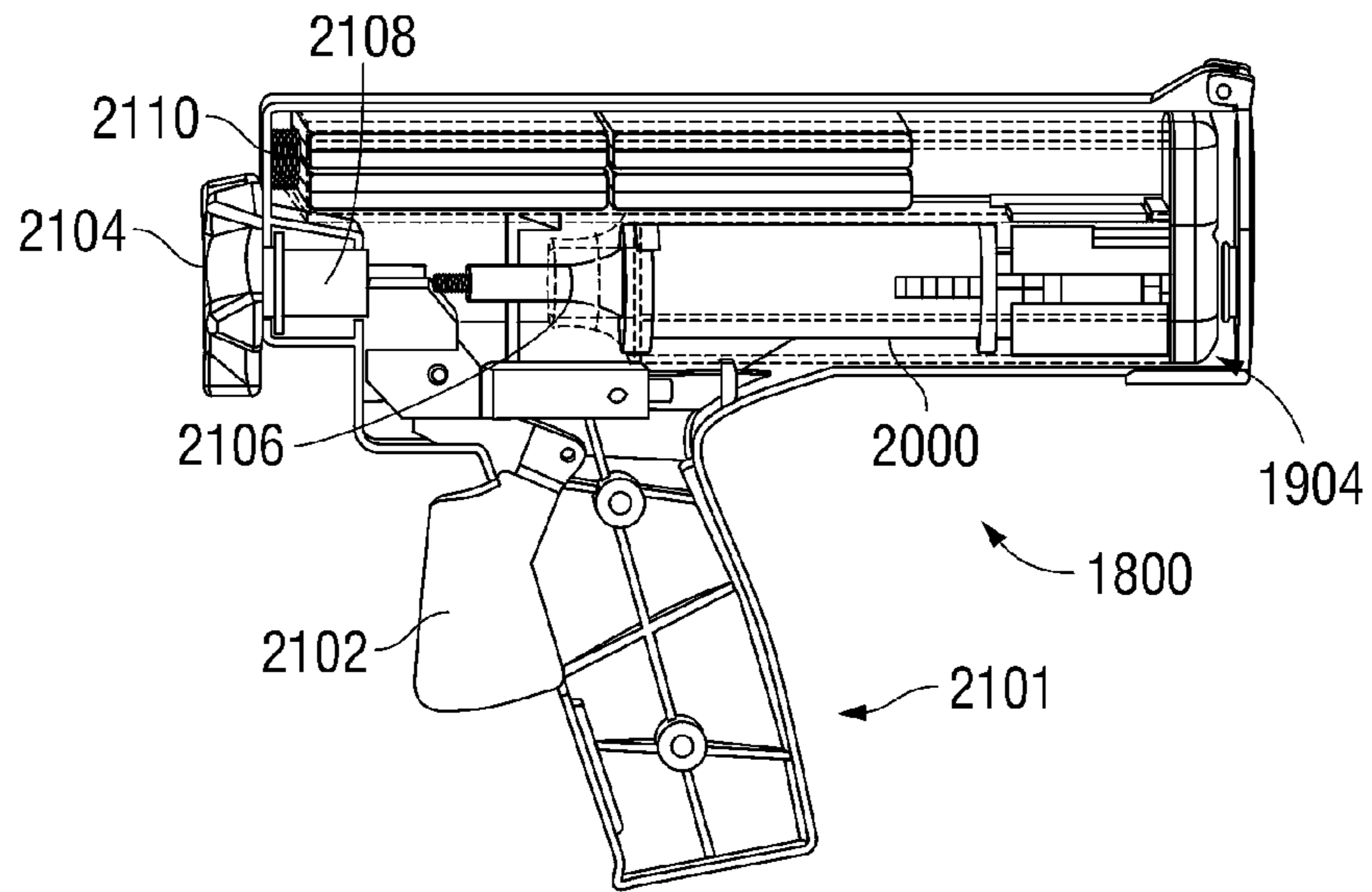
FIG. 21
