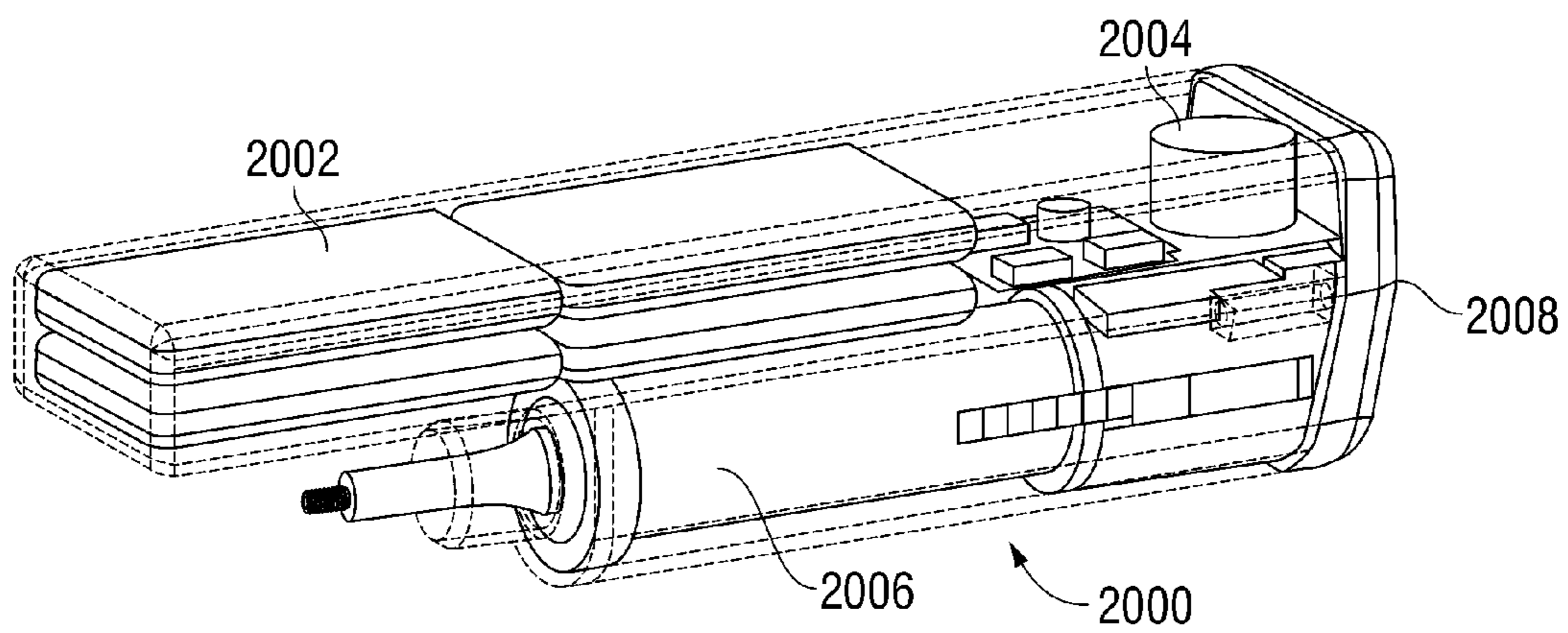
FIG. 20
