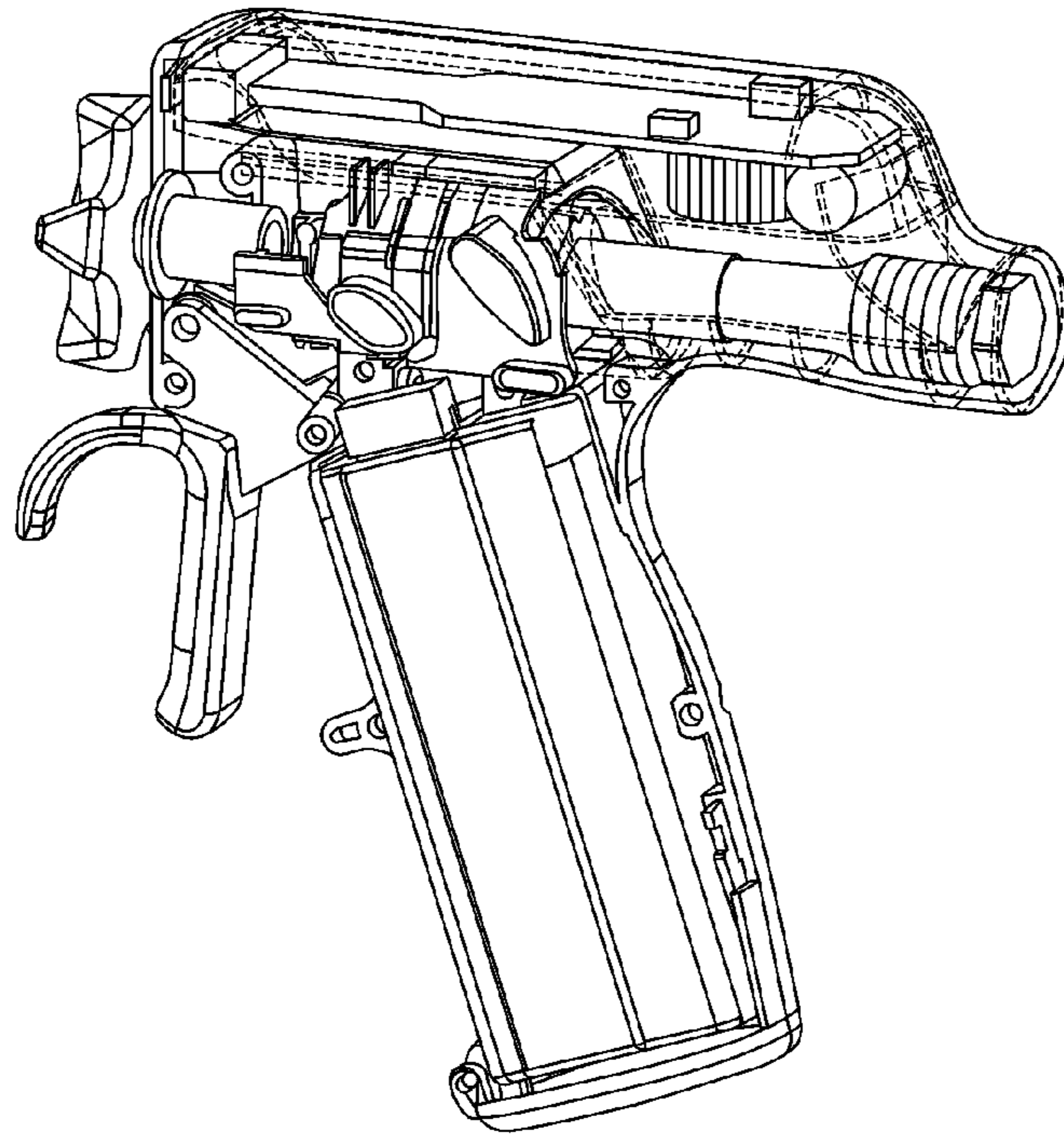
FIG. 27
