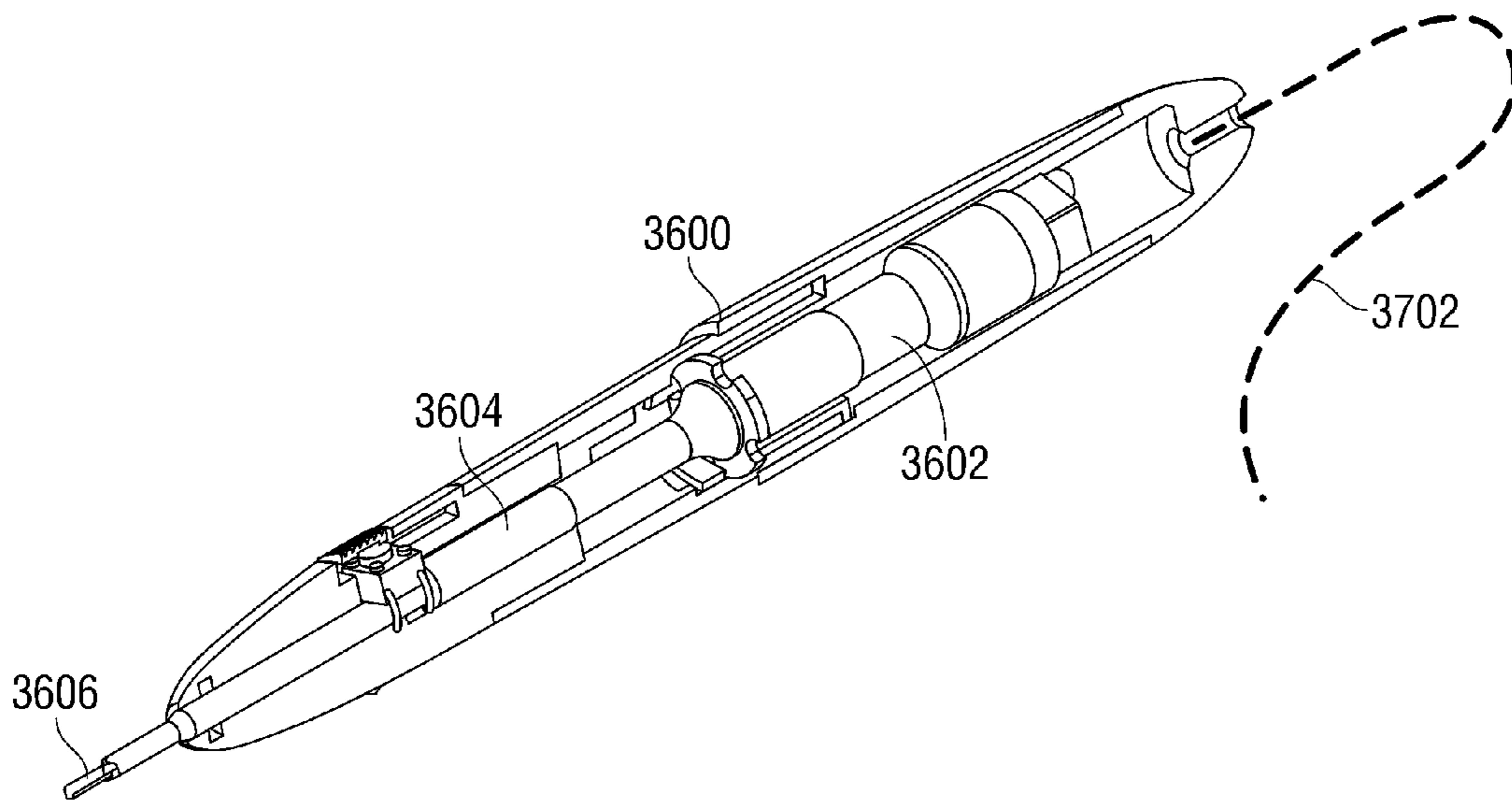
FIG. 36
