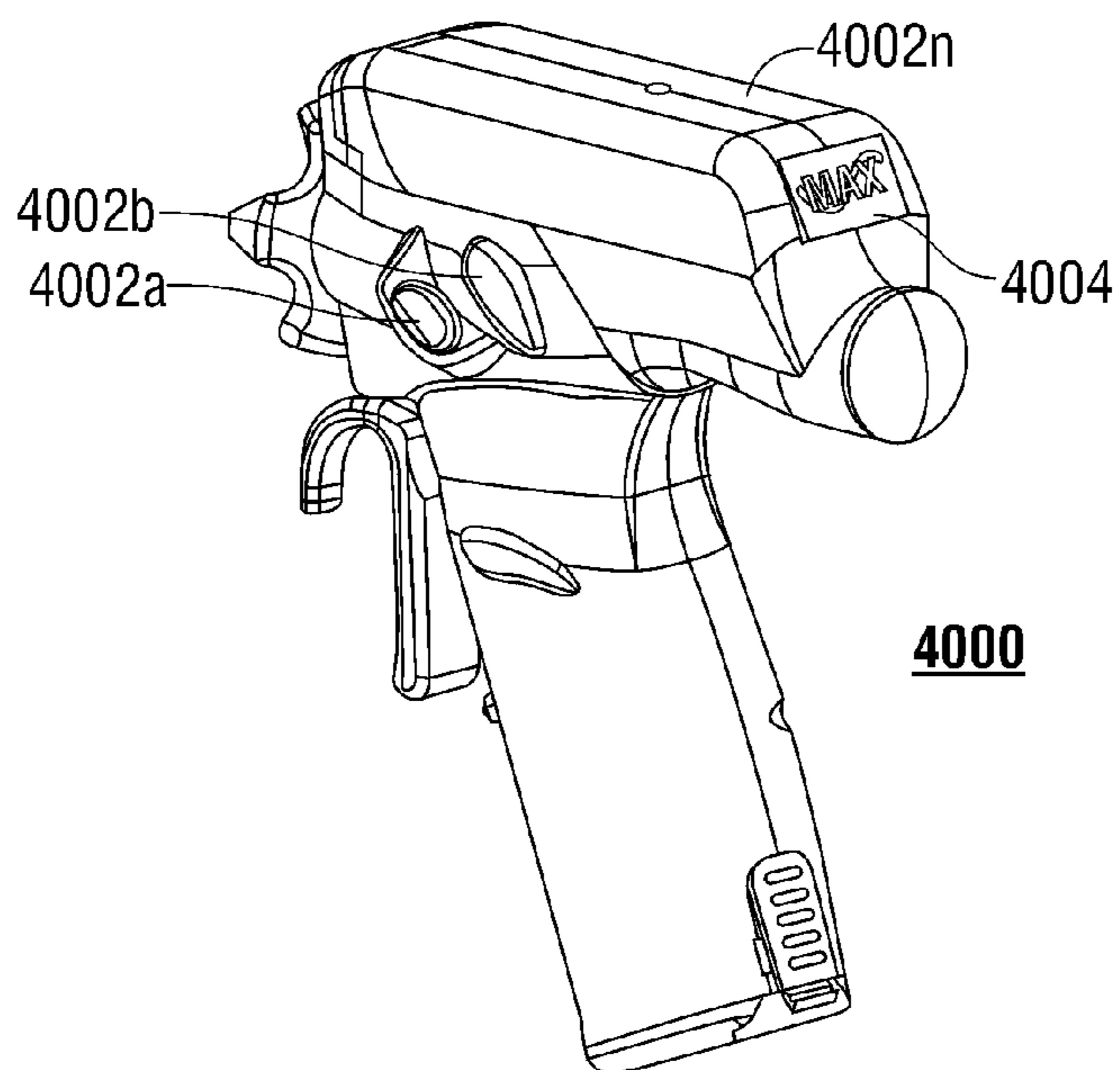
FIG. 40
