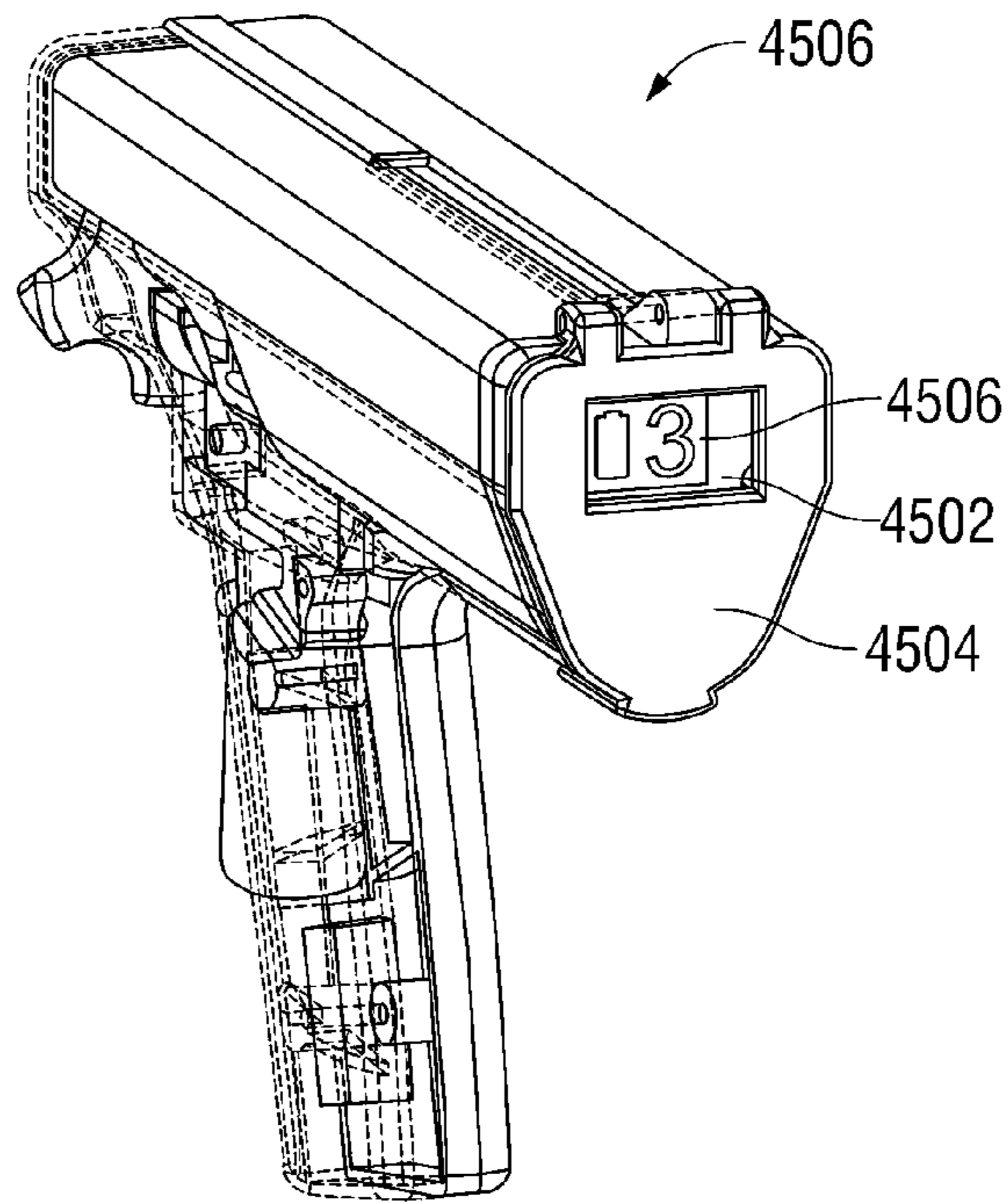
FIG. 45
