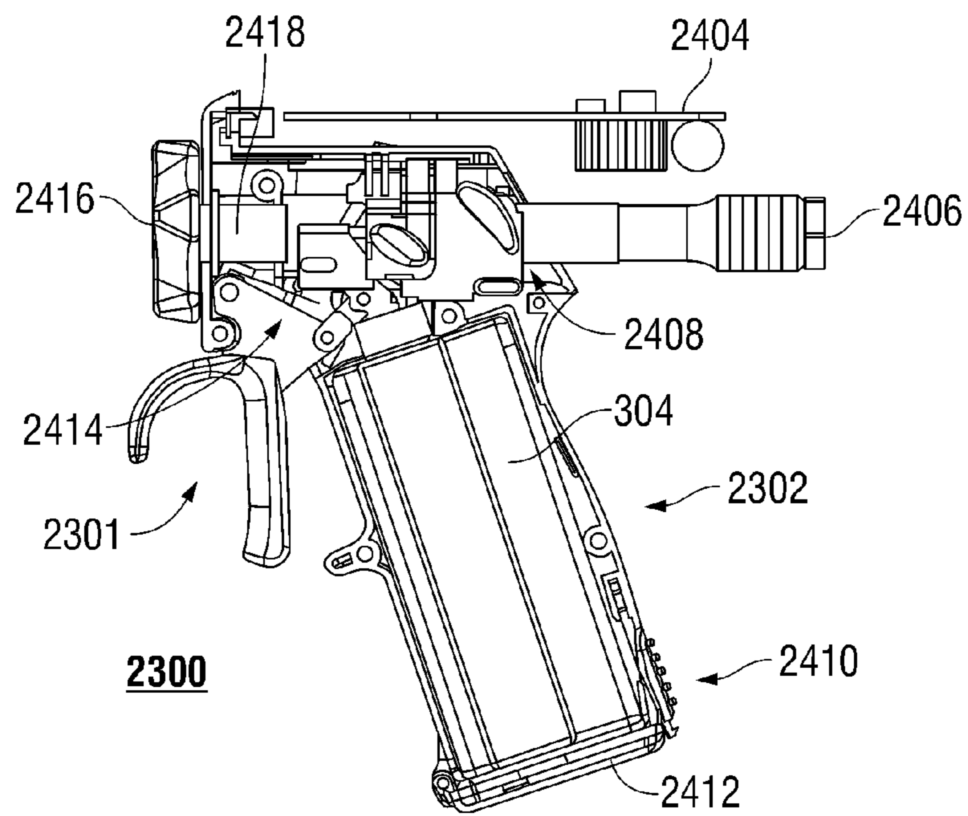
FIG. 24
