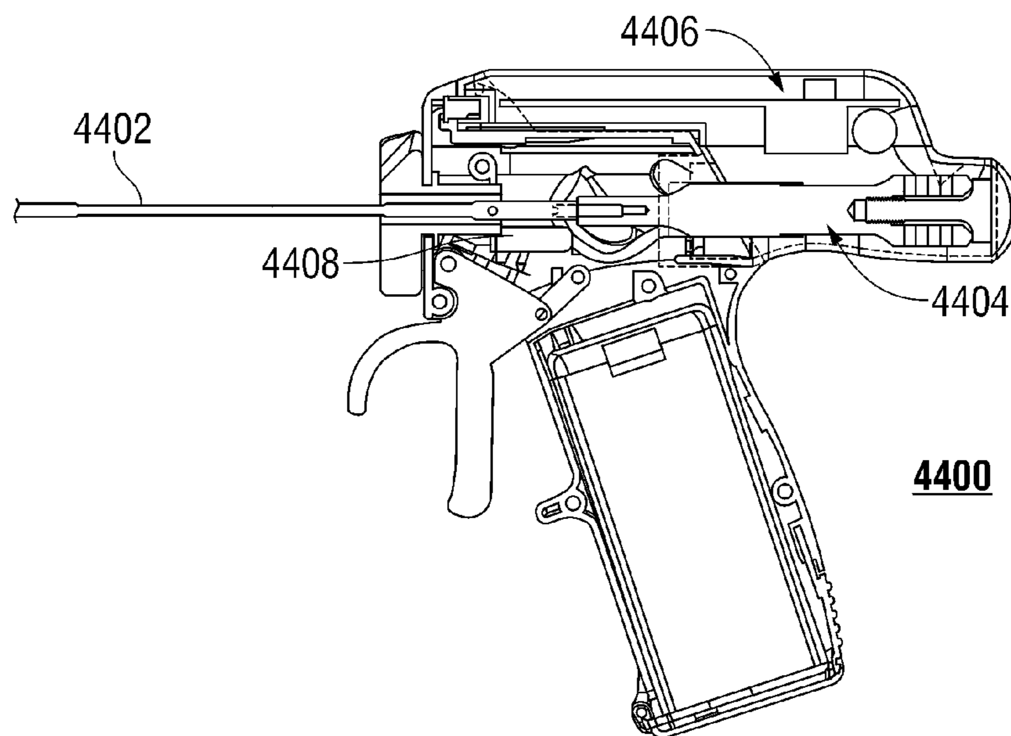
FIG. 44
