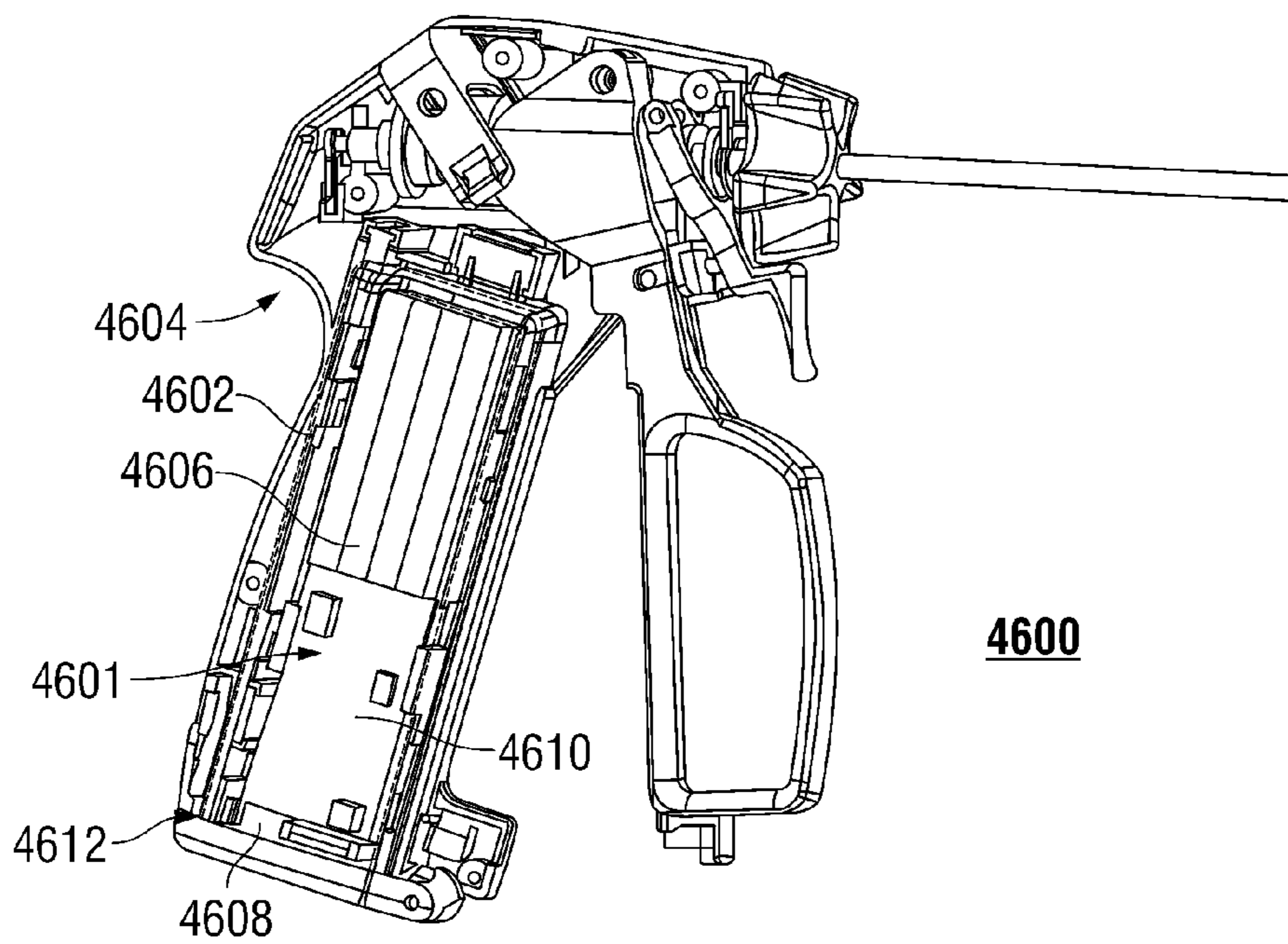
FIG. 46
