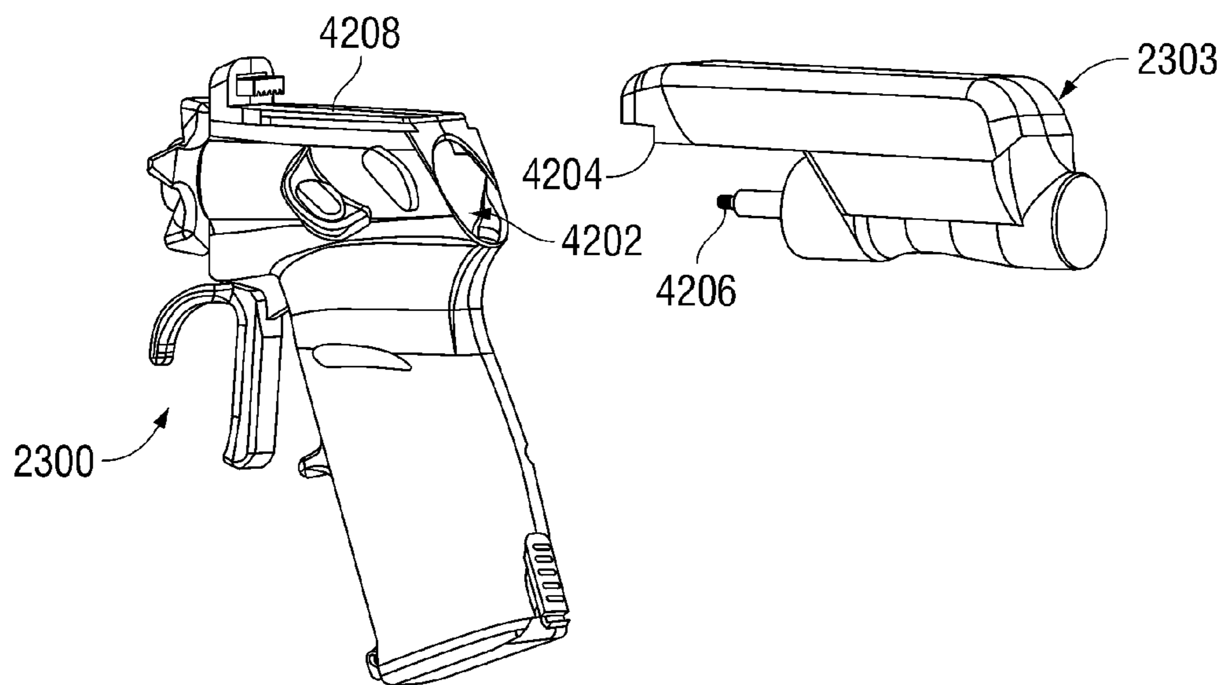
FIG. 42
