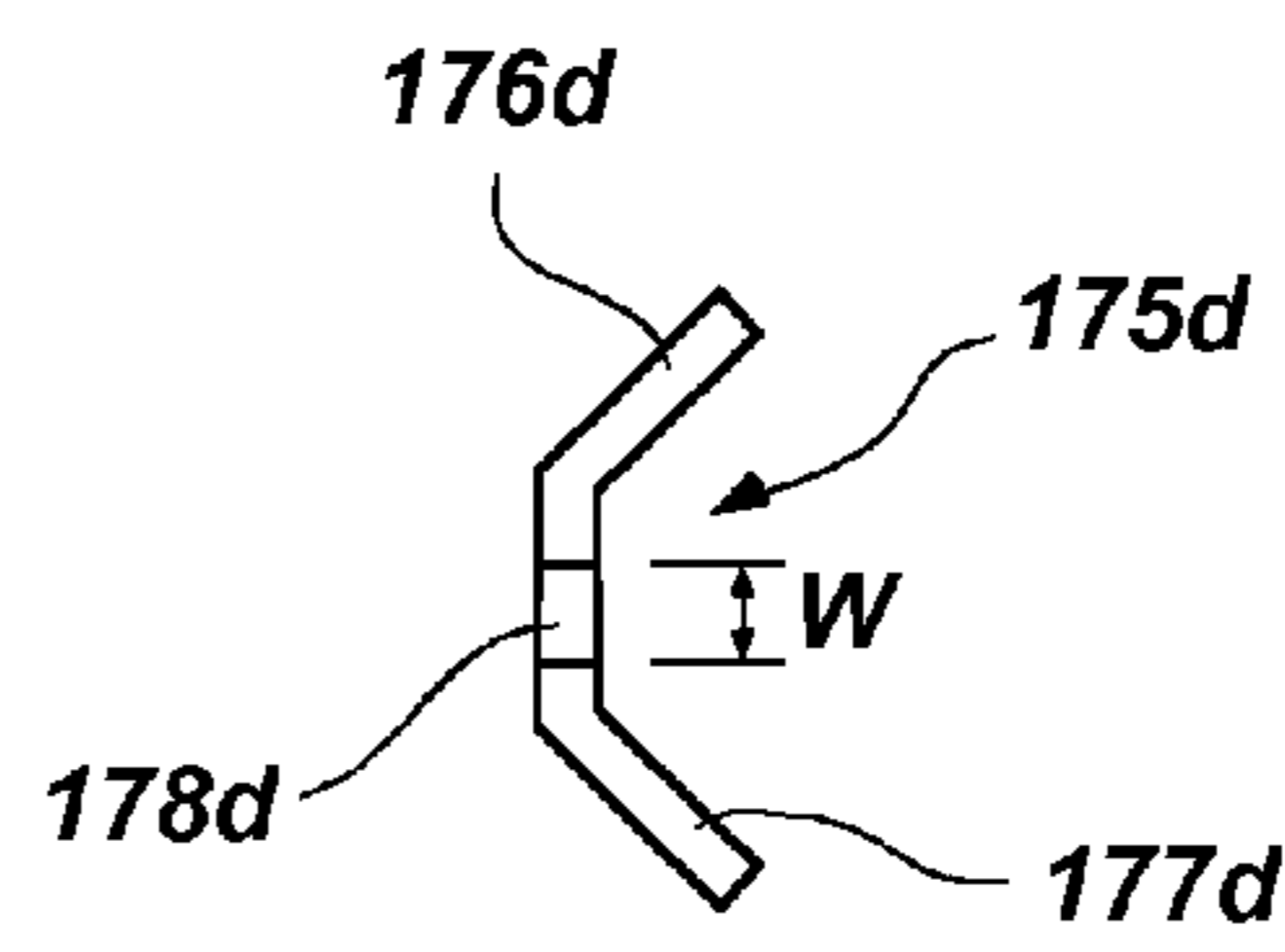
FIG. 7D
