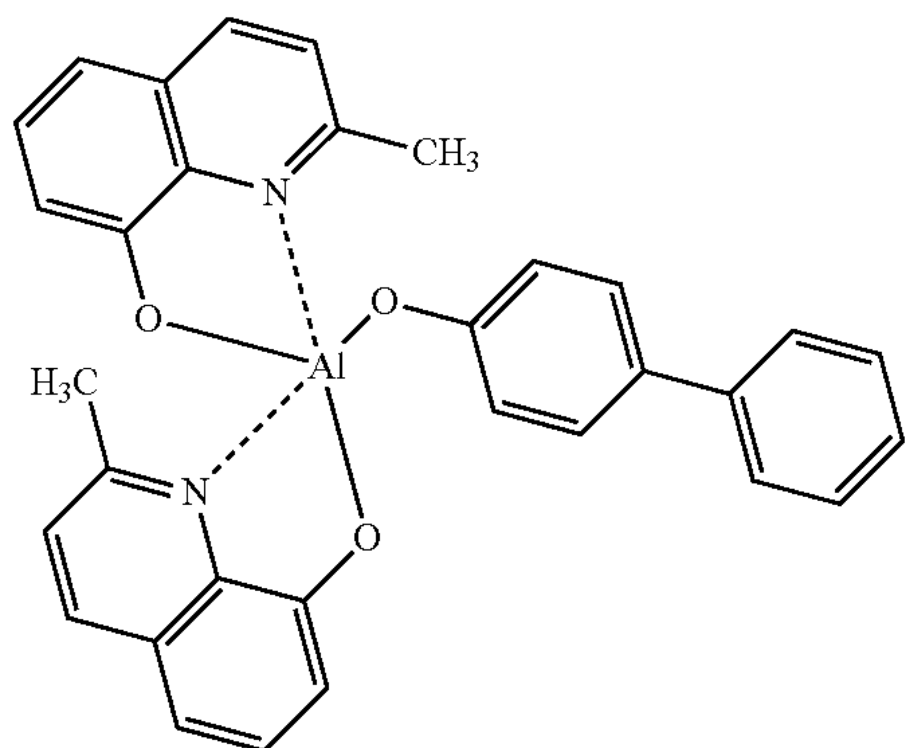
BALq
