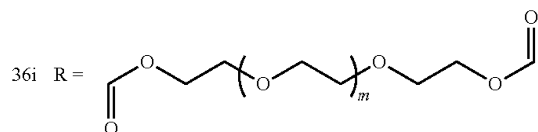
Poly(CDDCys-CB-PEG)
