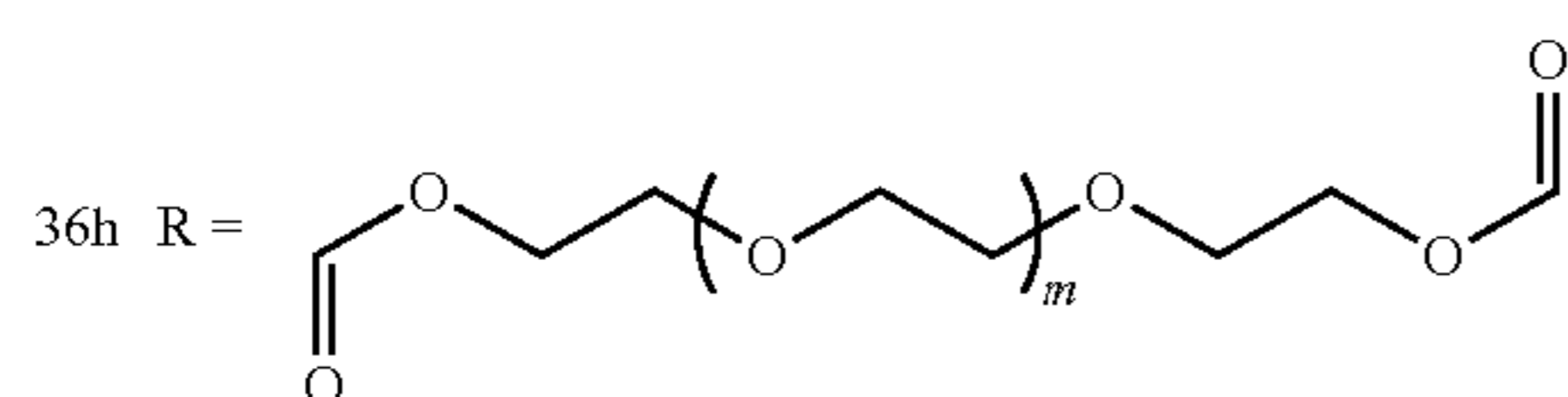
Poly(CDDCys-CB-PEG)
