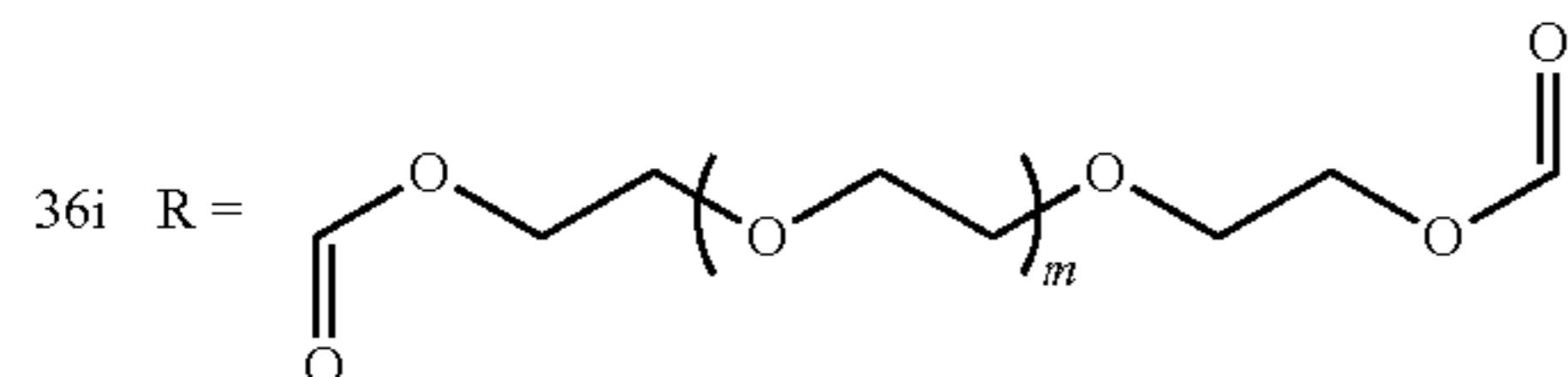
Poly(CDDCys-CB-PEG)
