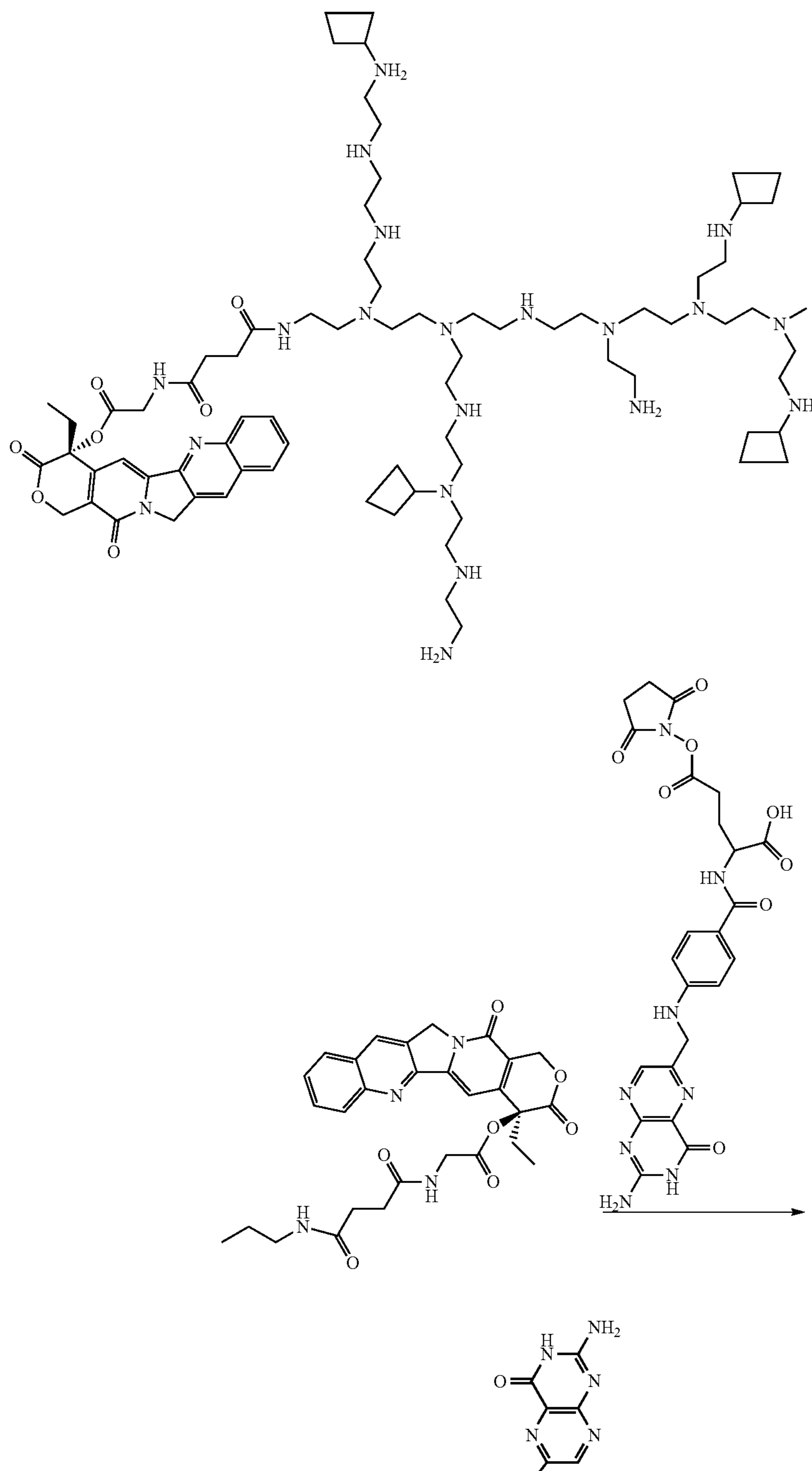
Scheme LI
