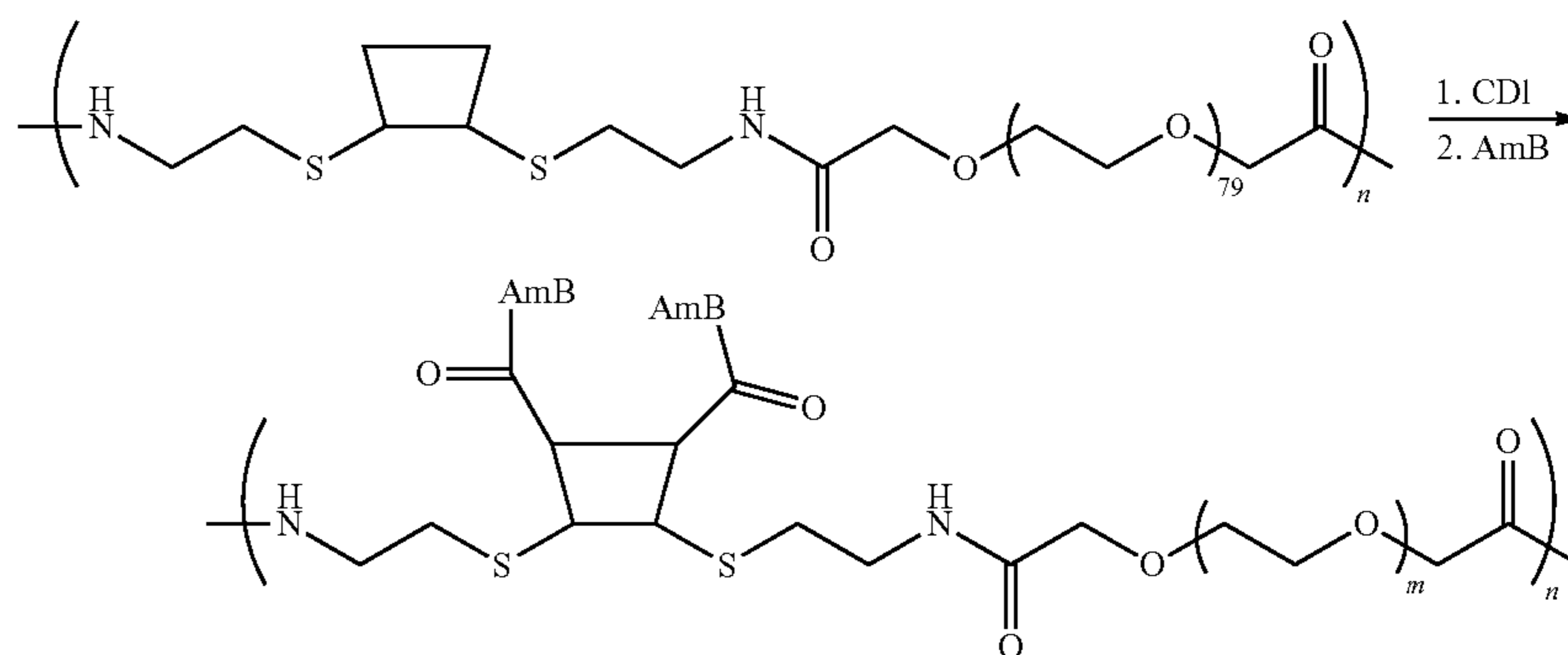
Scheme LII
