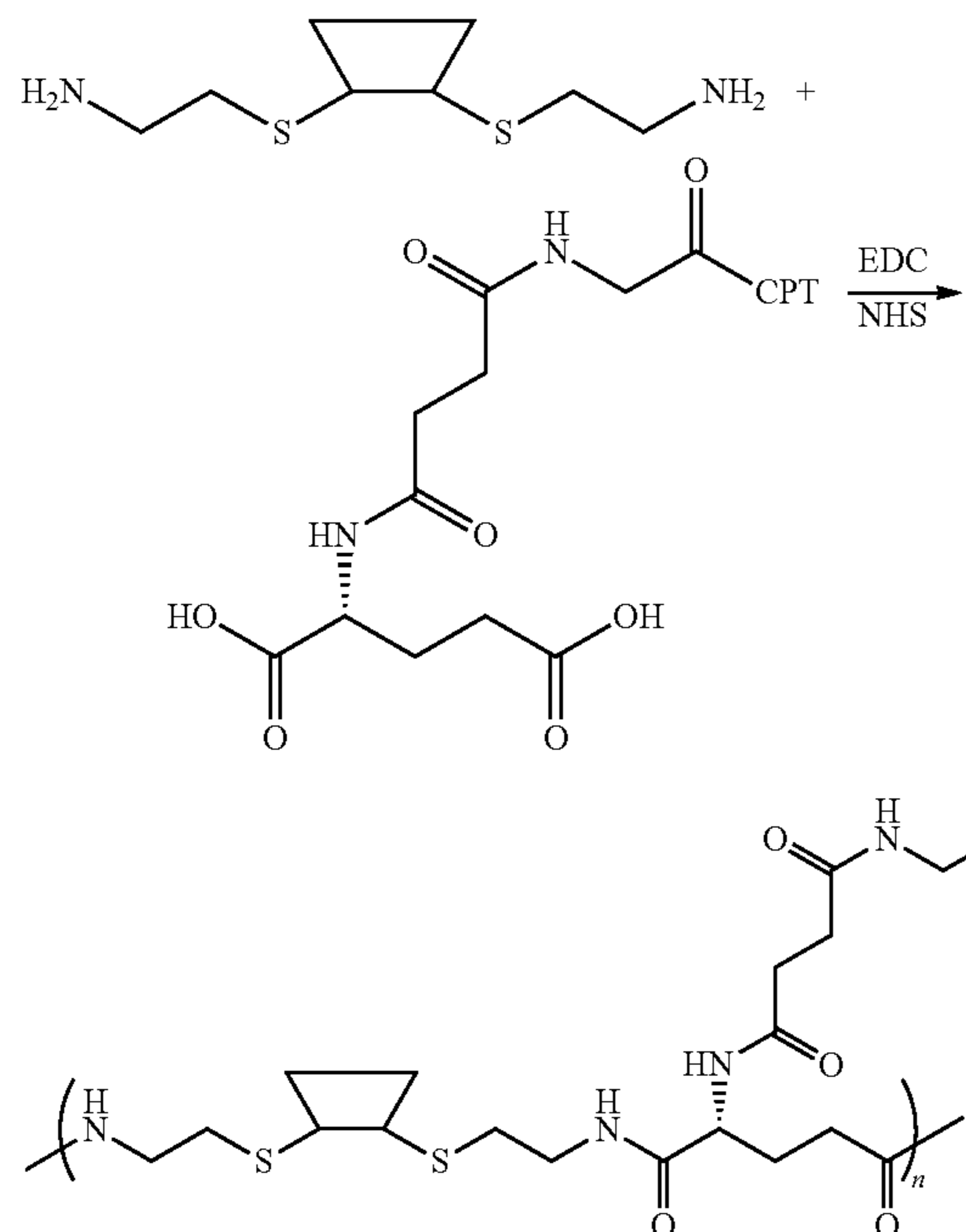
Scheme VI
