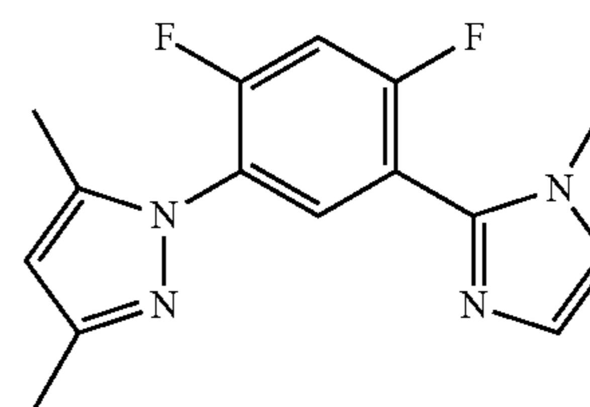
DMPz-DFPh-MIz
