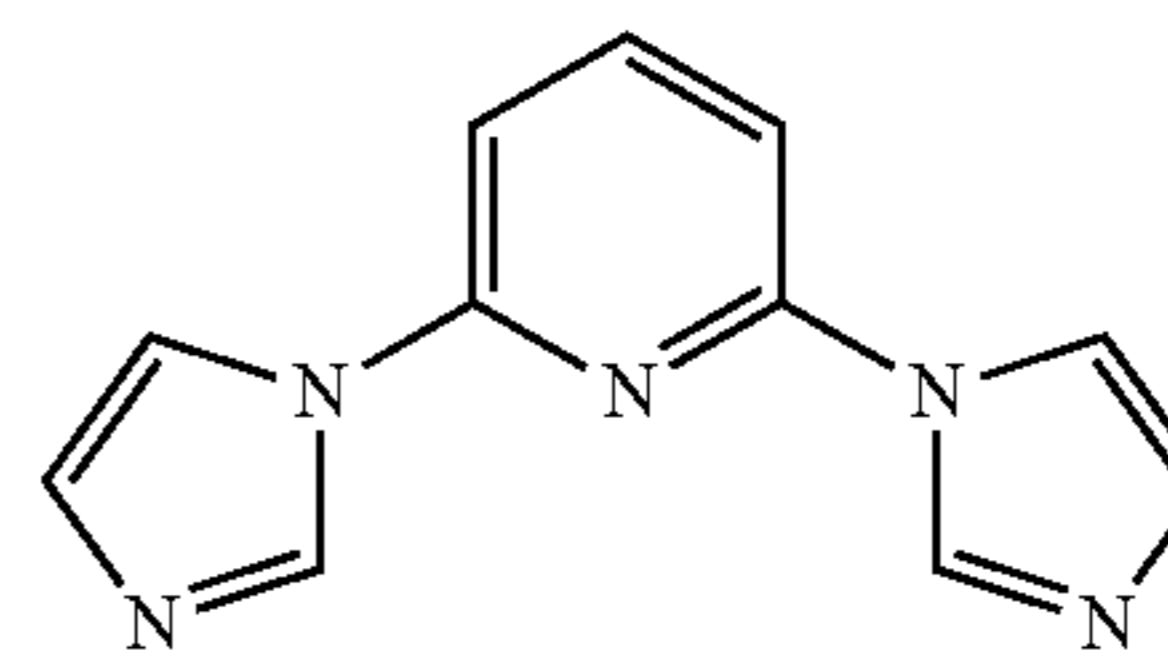
DIz-Py
