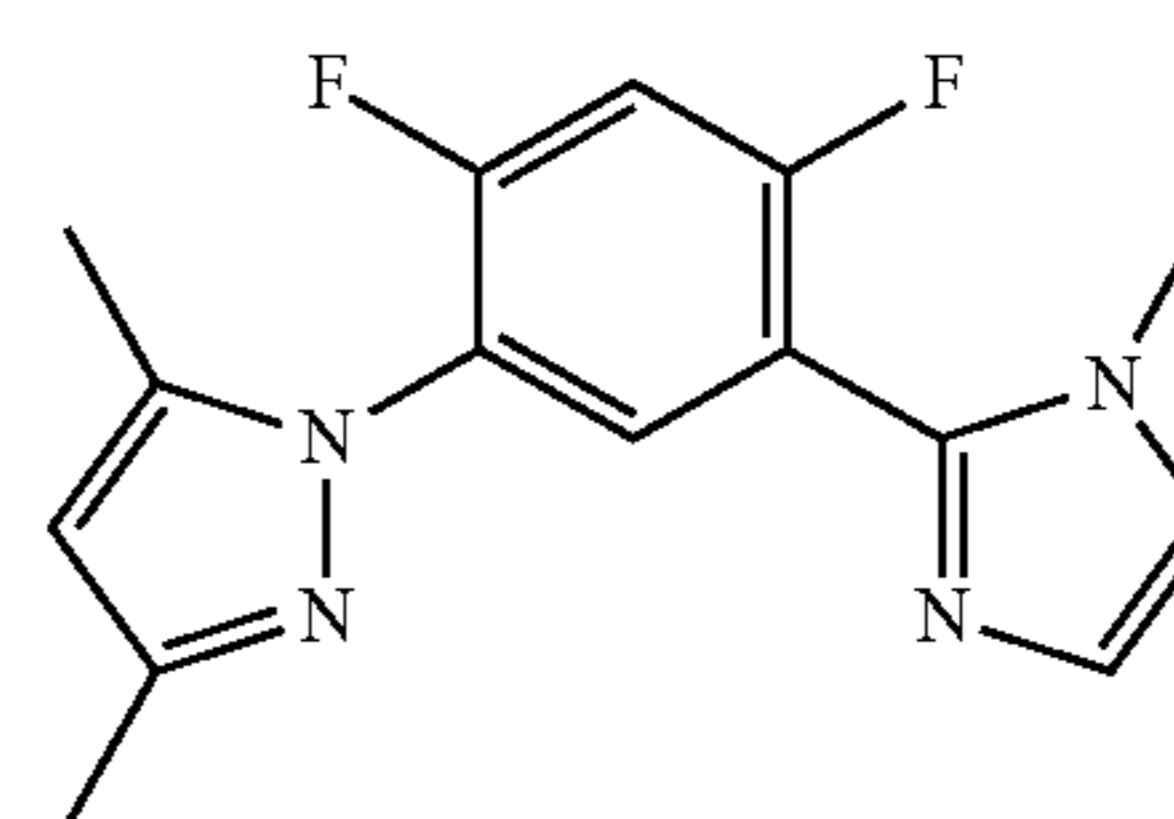
DMPz-DFPh-MIz
