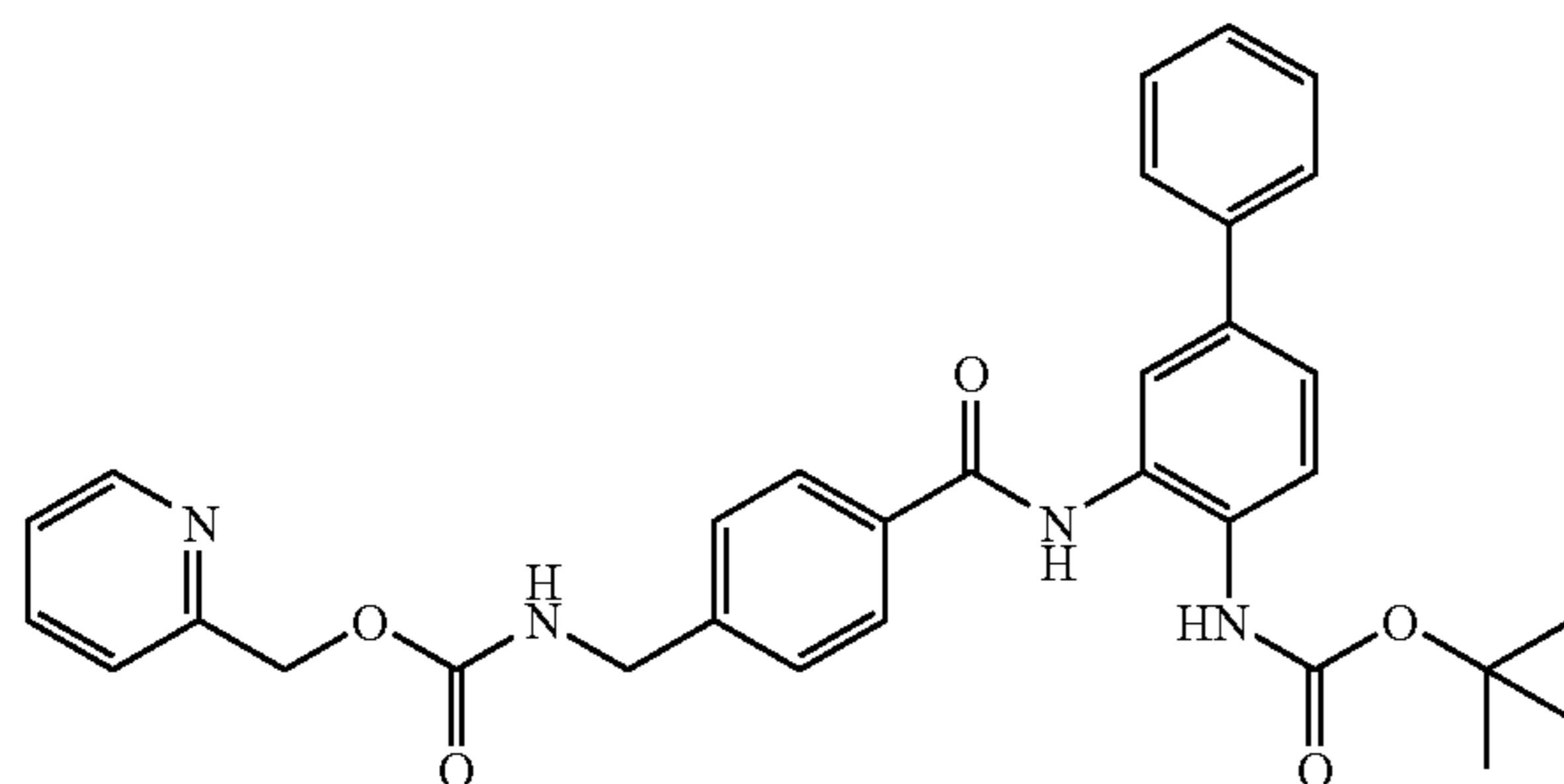
1,1-dimethylethyl{3-(((4-(((pyridin-2-ylmethyl)oxy)carbonyl)amino)methyl)phenyl)carbonyl)amino)biphenyl-4-yl}carbamate
