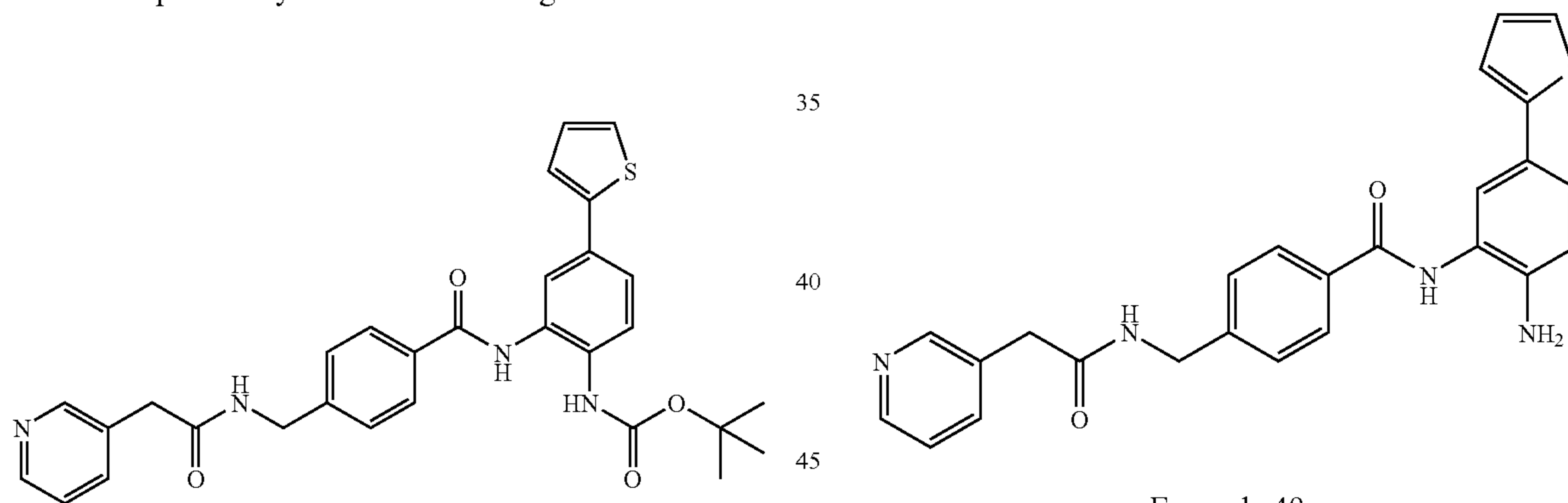
N-[2-amino-5-(2-thienyl)phenyl]-4-[(pyridin-3-ylacetyl)amino]methyl]benzamide
