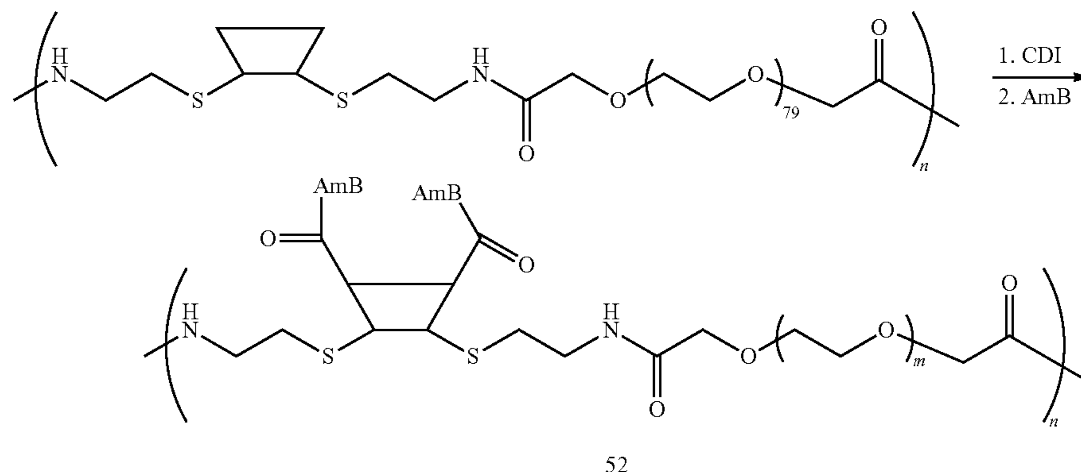
Scheme LII
