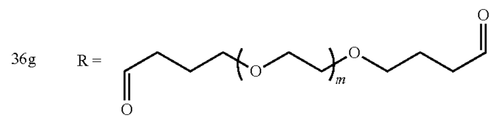
Poly(CDDCys-BA—PEG)
