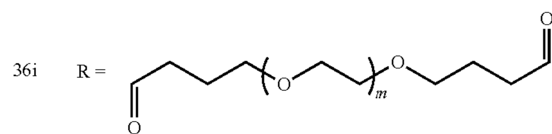
Poly(CDDCys-CB—PEG)
