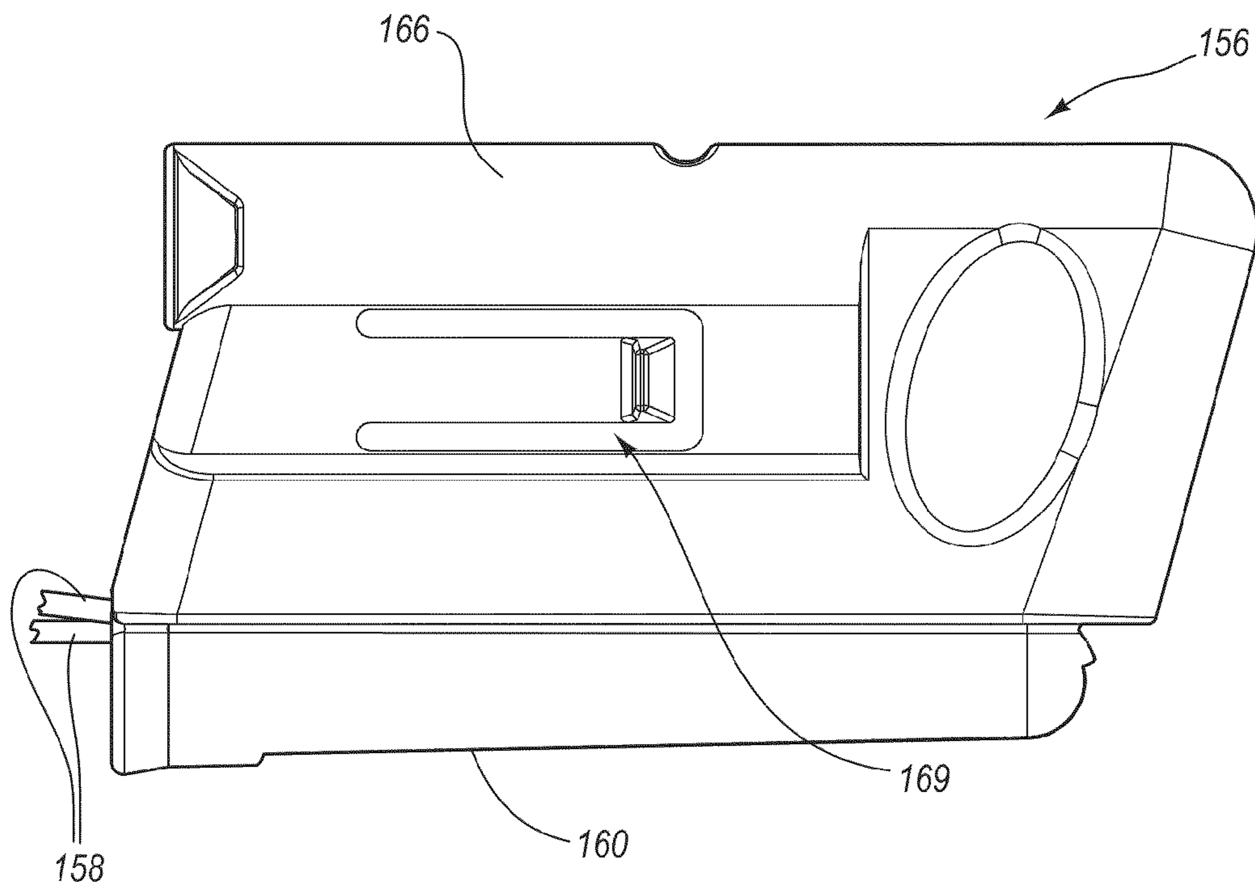
FIG. 13C
