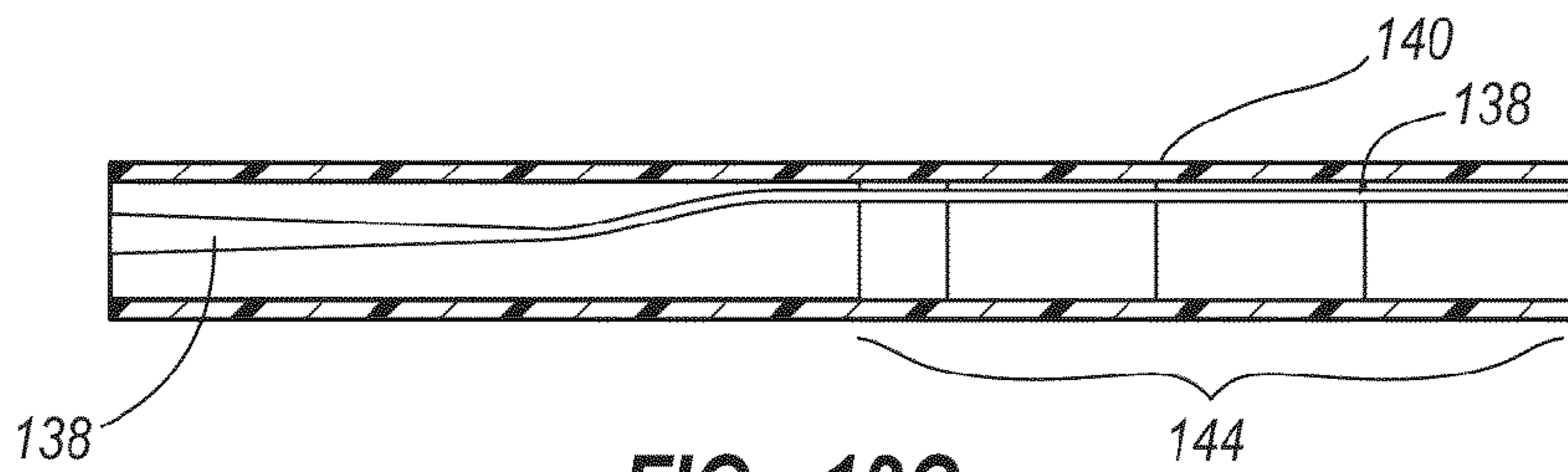
FIG. 12C
