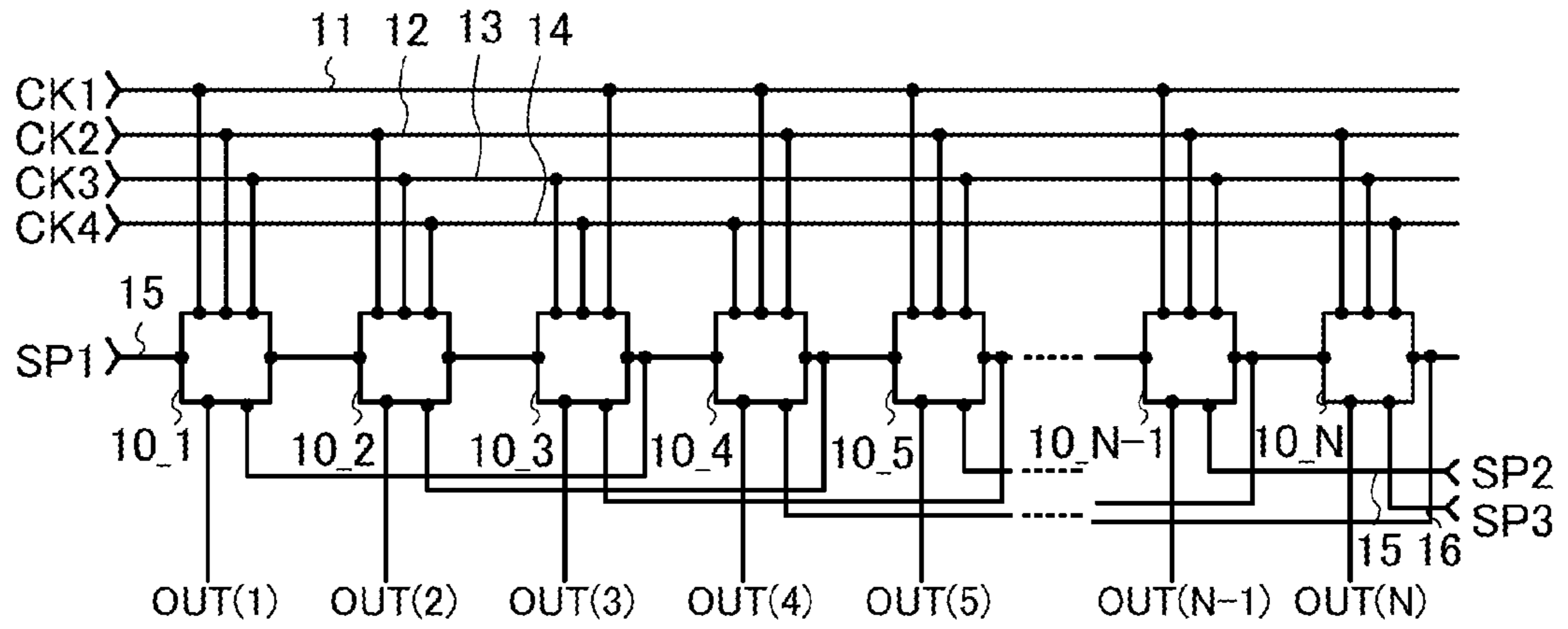
FIG. 16A
