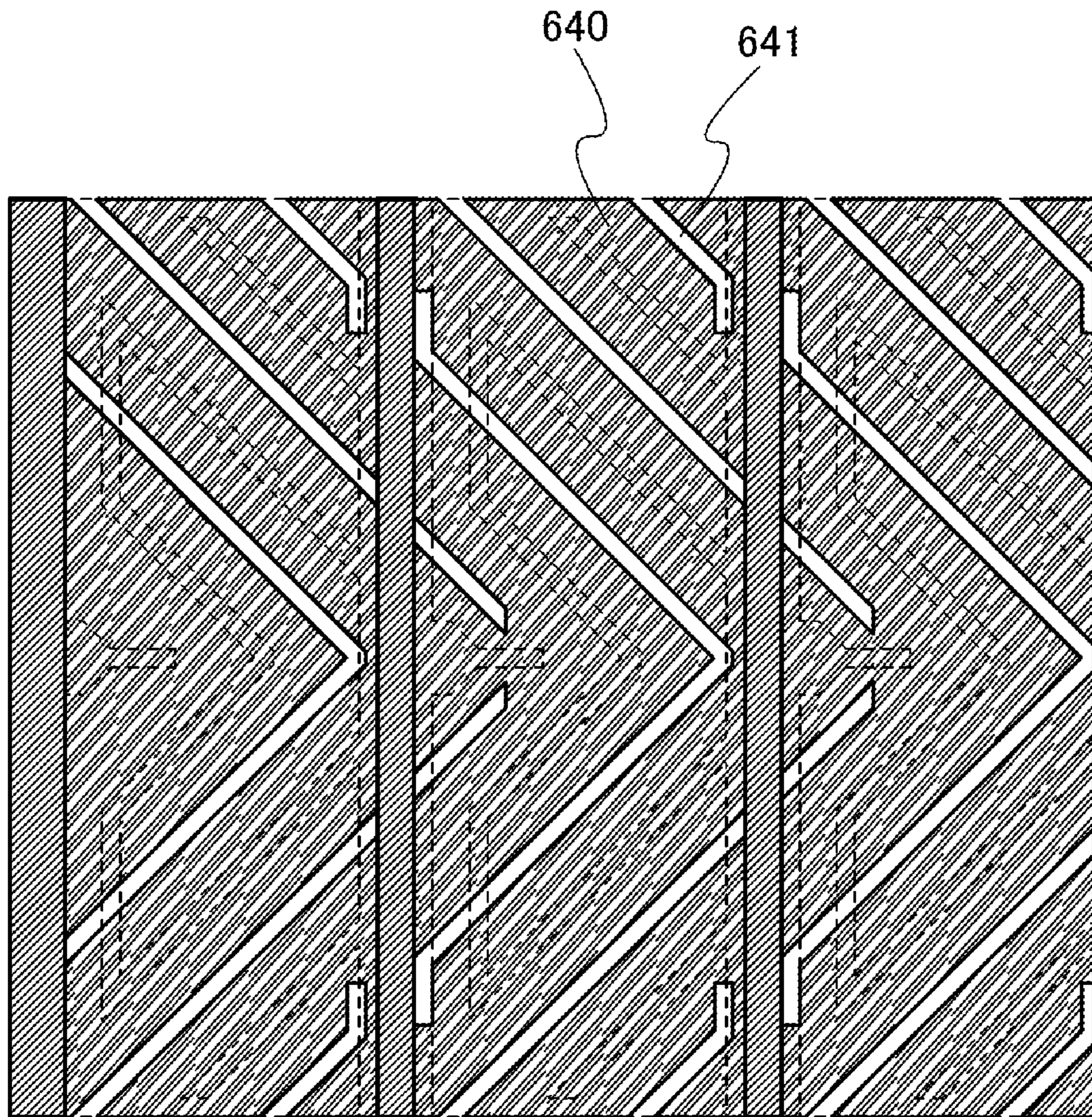
FIG. 30
