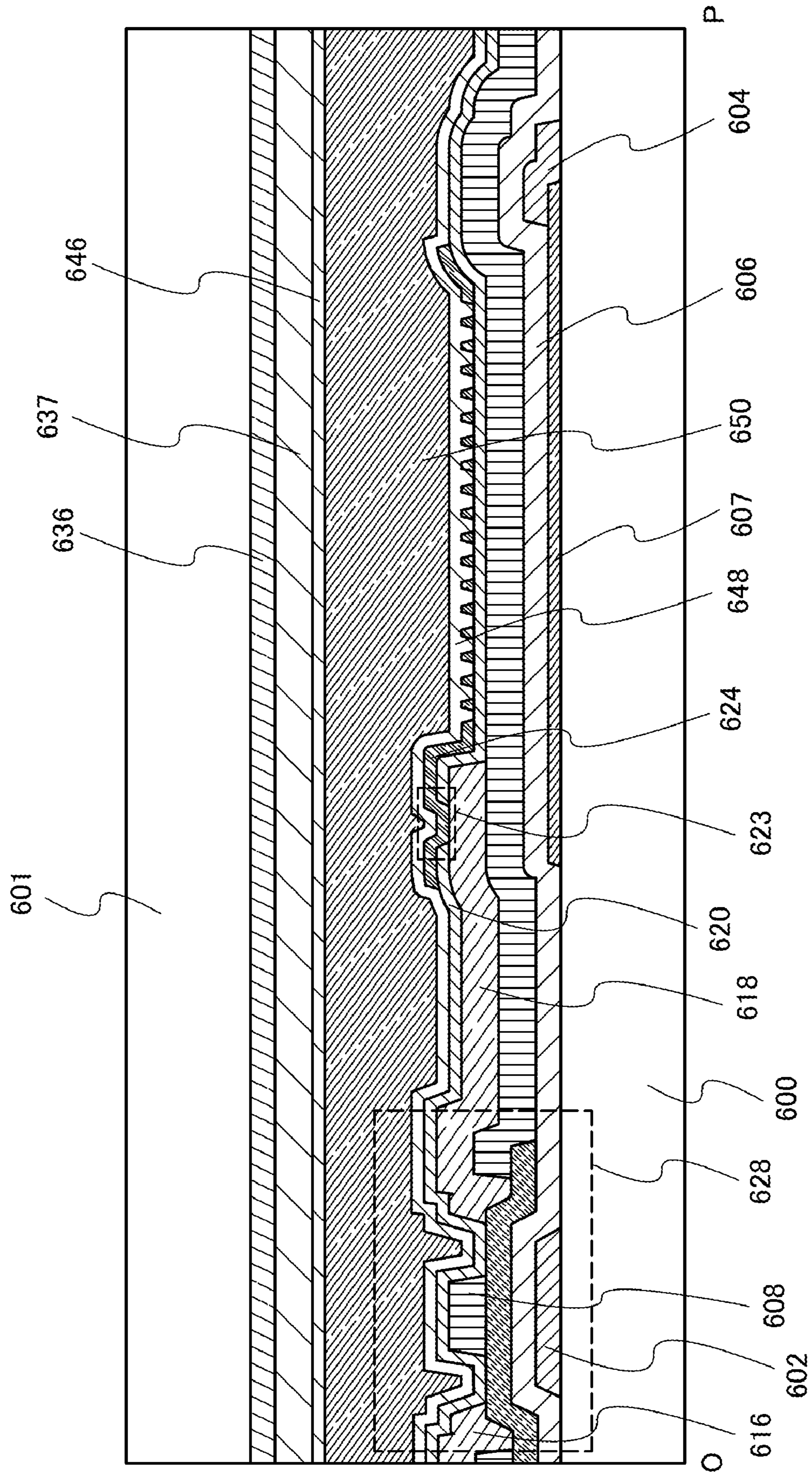
FIG. 32
