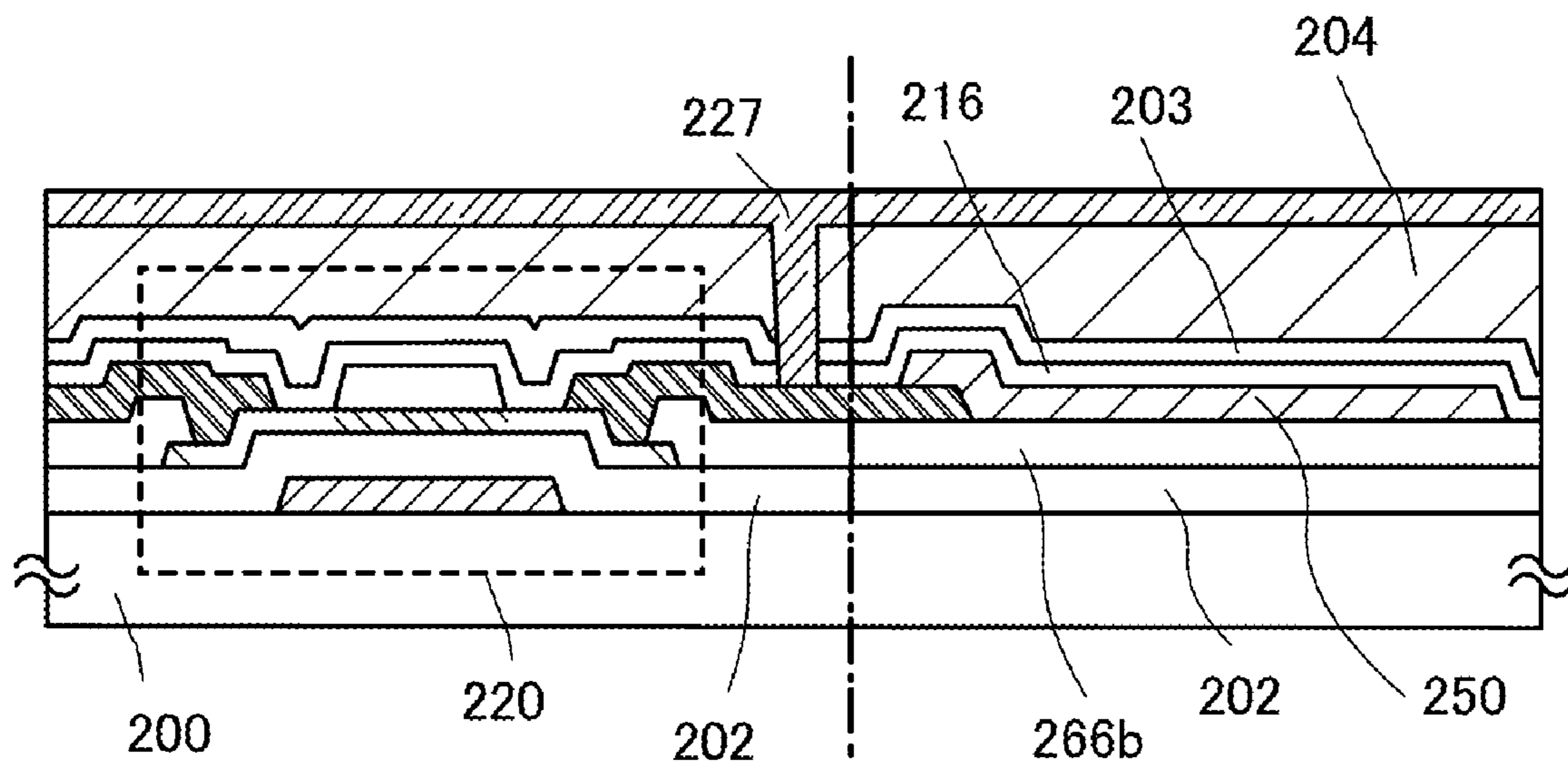
FIG. 9A
