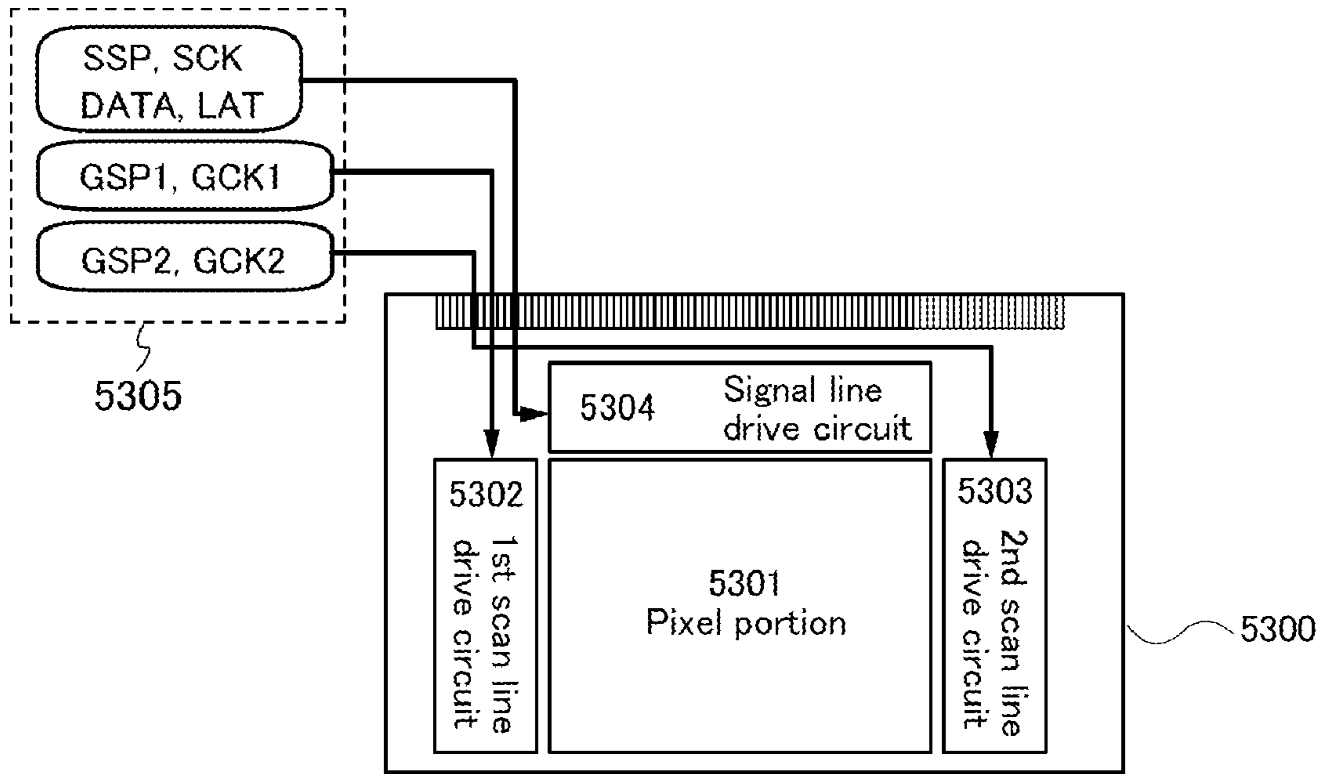
FIG. 14B
