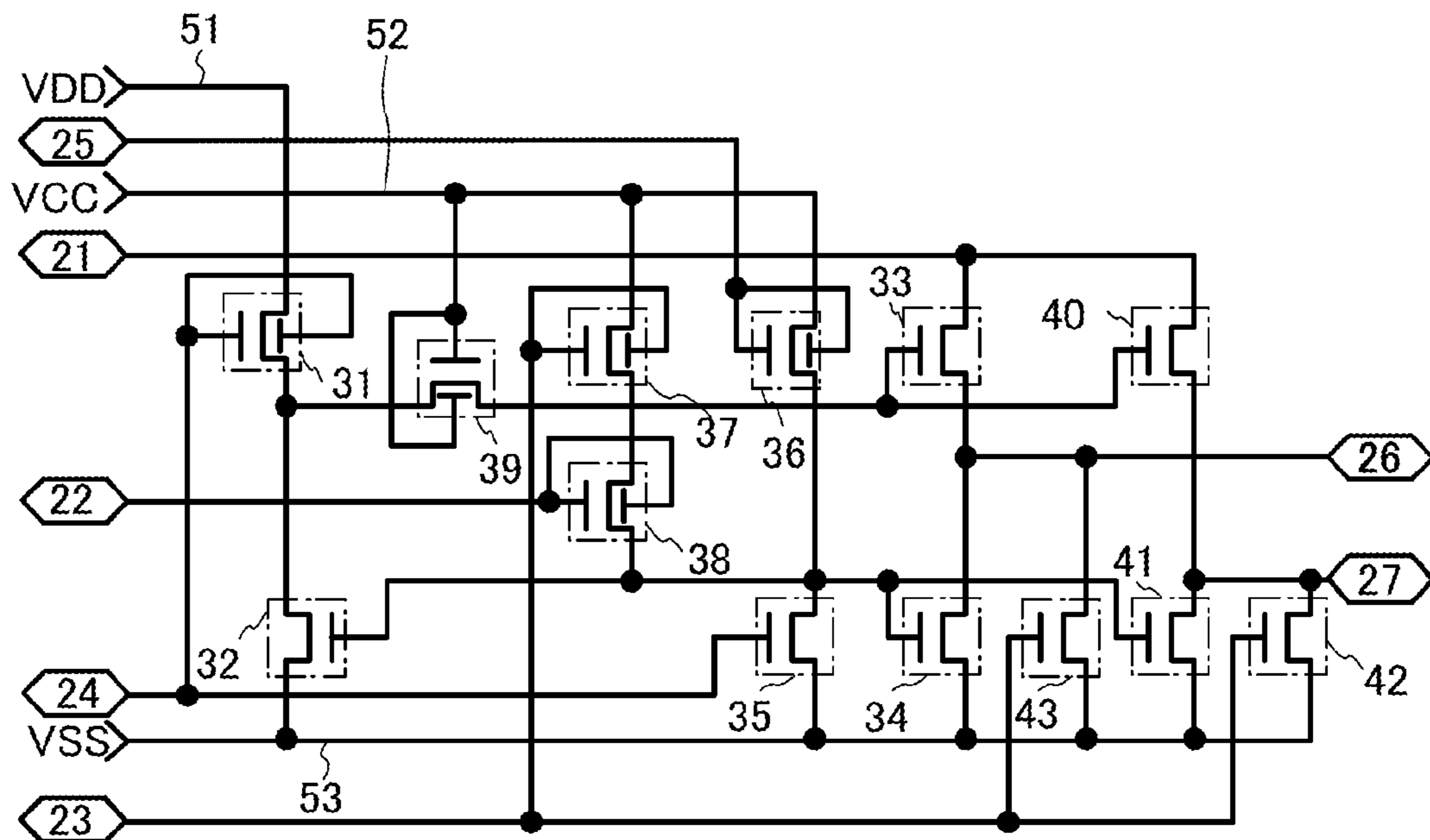
FIG. 16D
