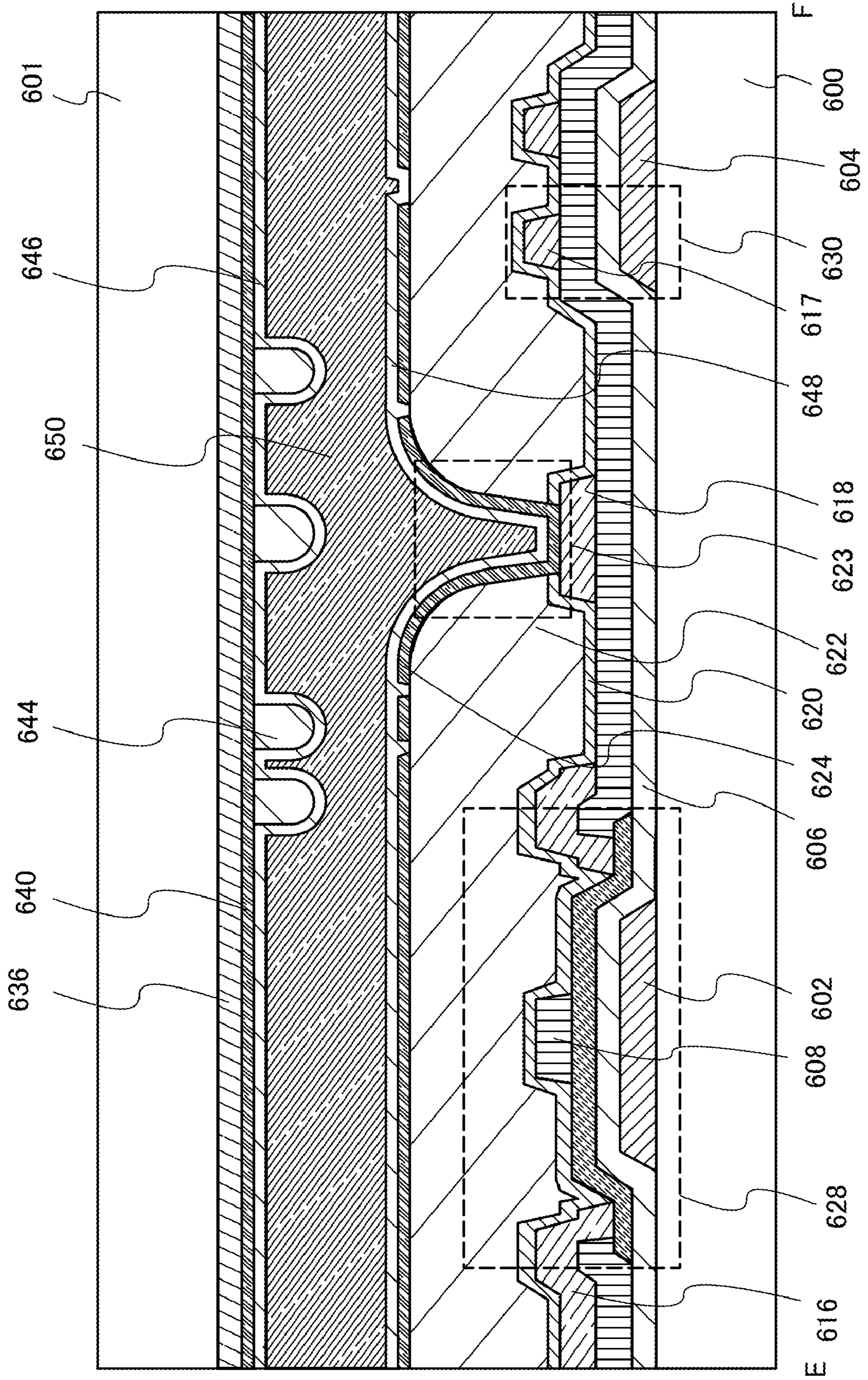
FIG. 24
