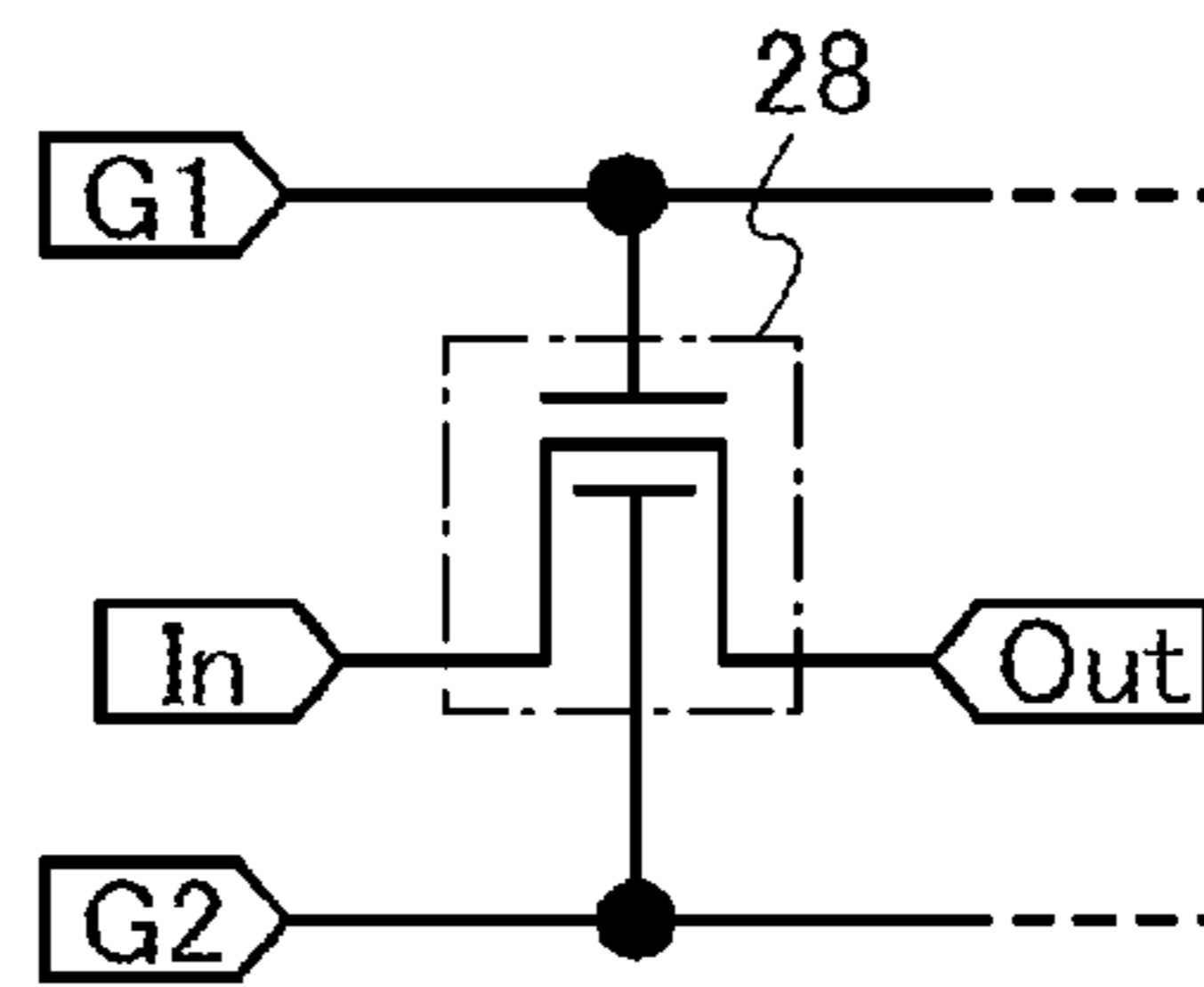
FIG. 16C
