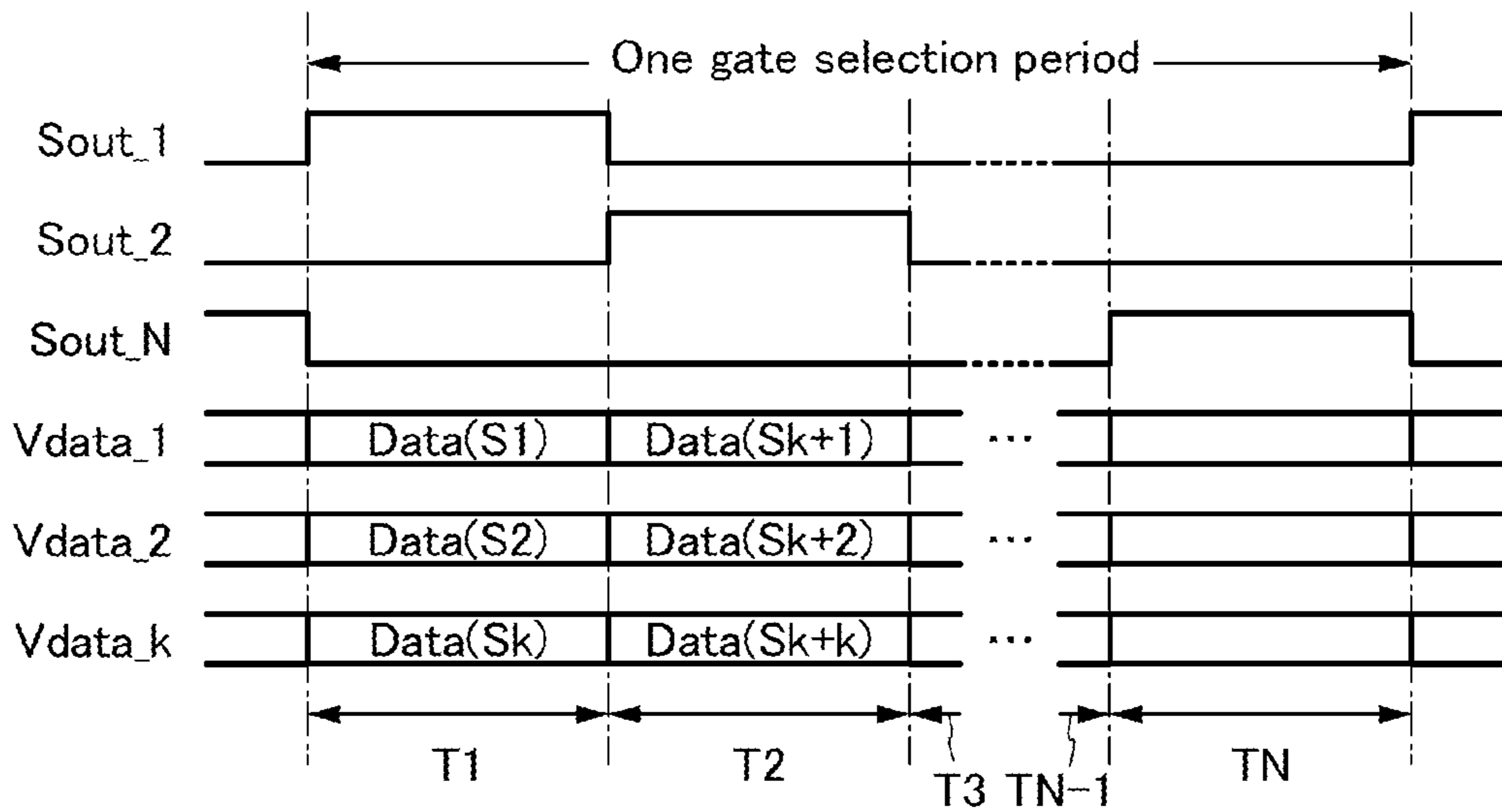
FIG. 15B
