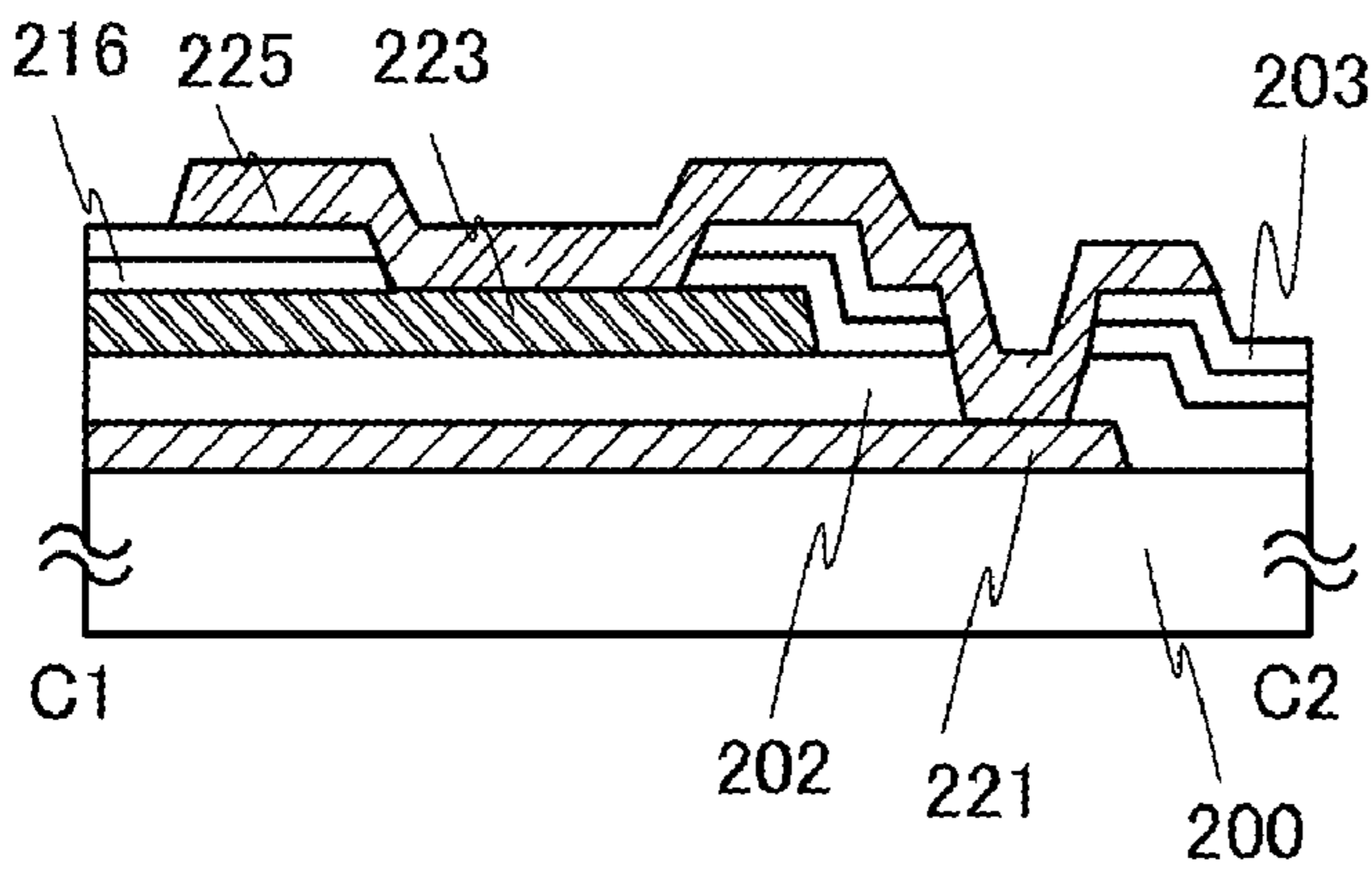
FIG. 4B1
