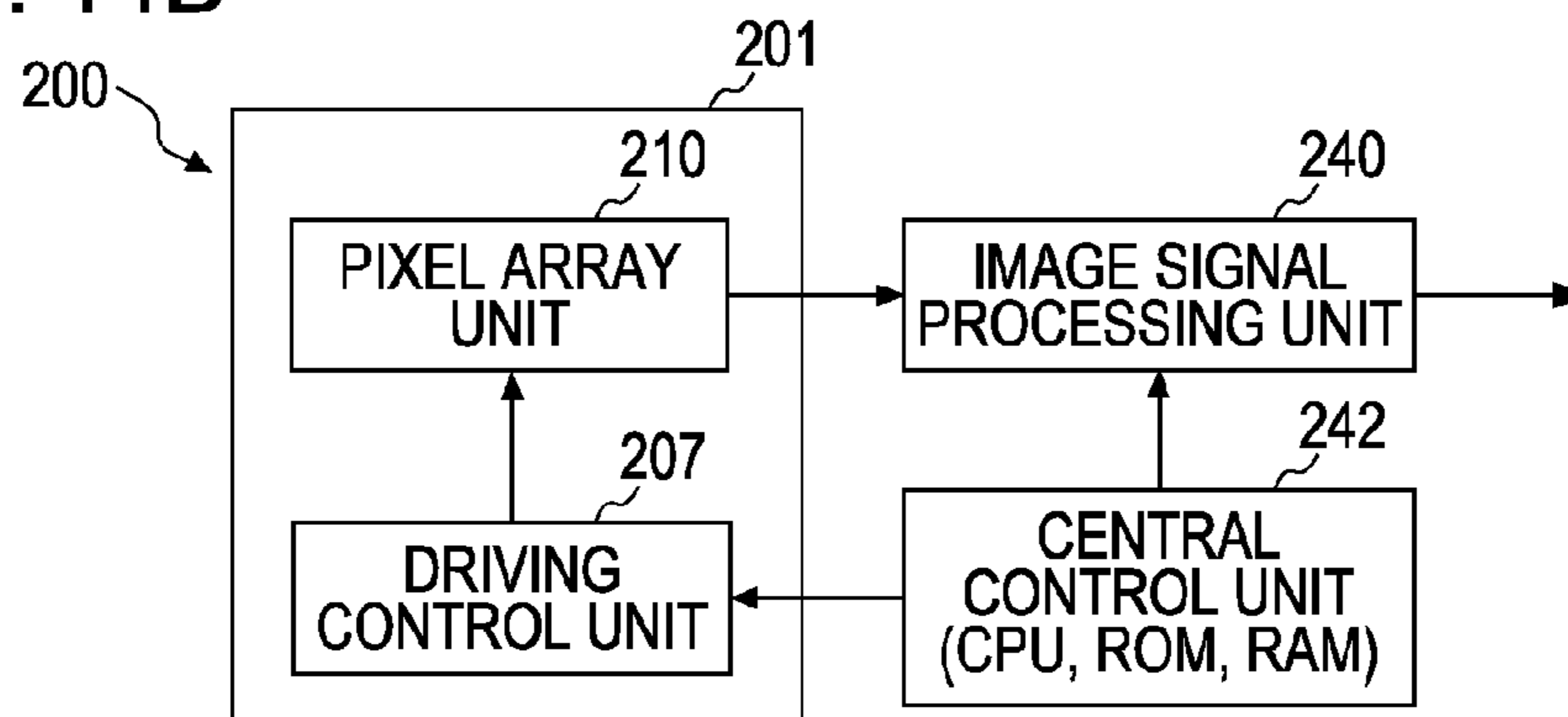
FIG. 14B
