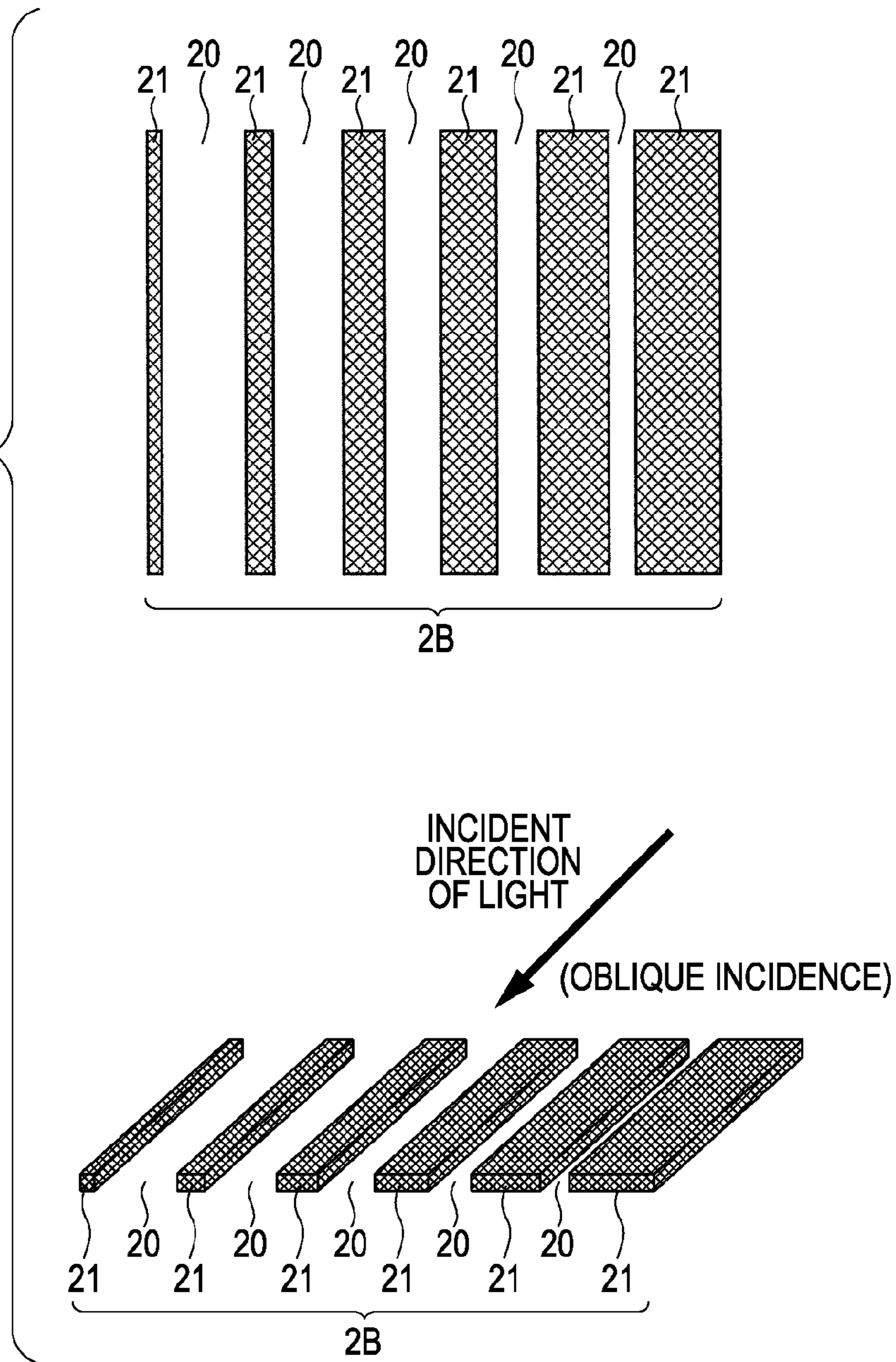
FIG. 10C
