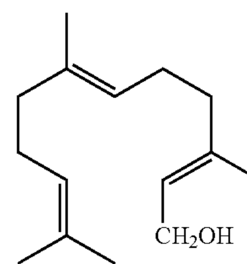
farnesol
