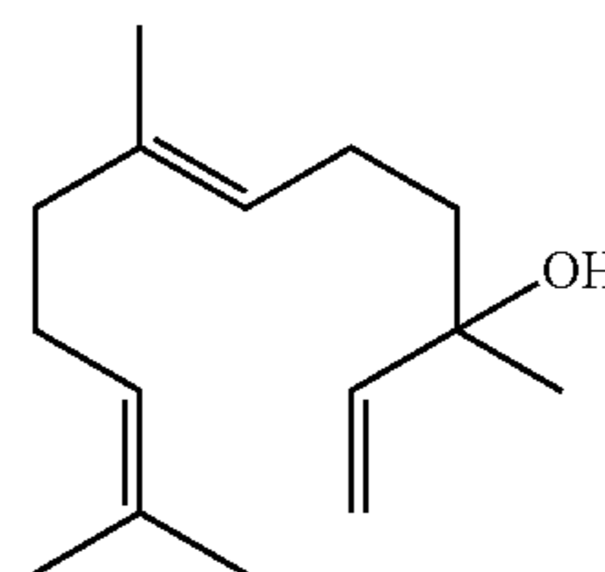
nerolidol
