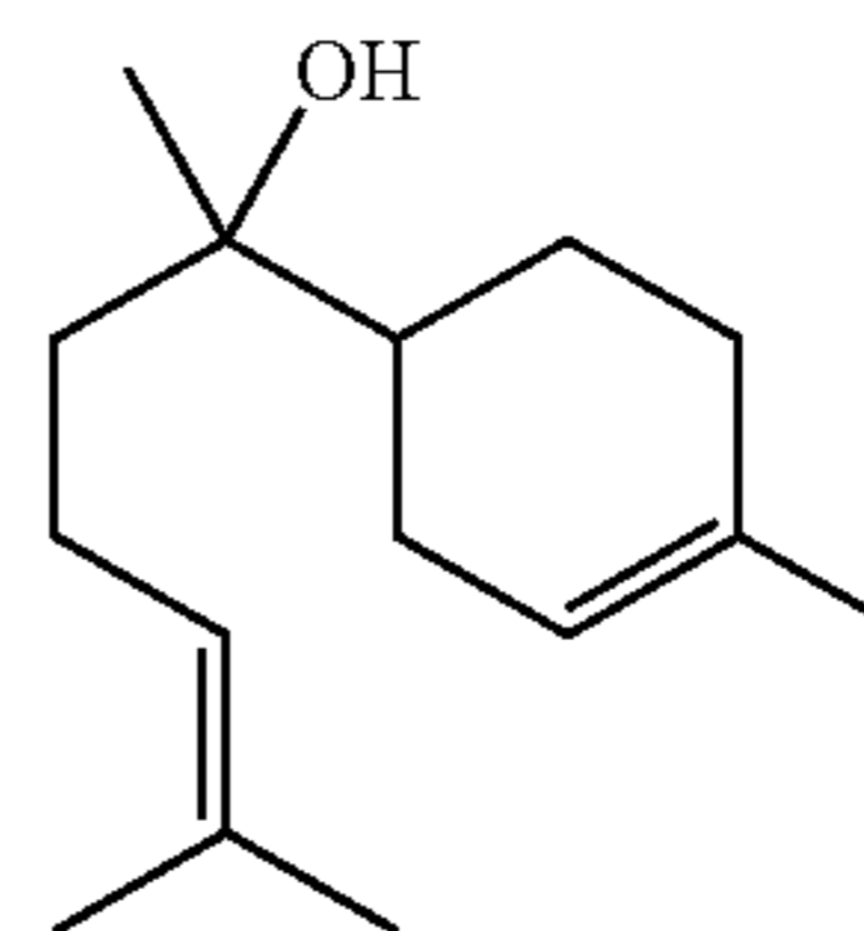
bisabolol
