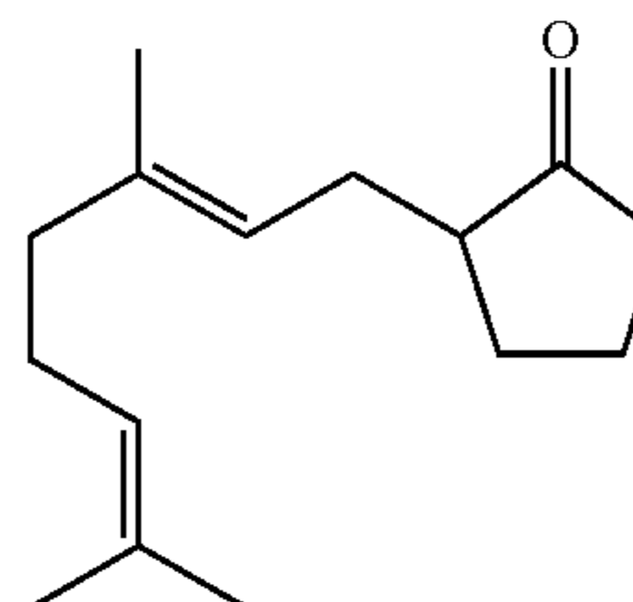
apritone
