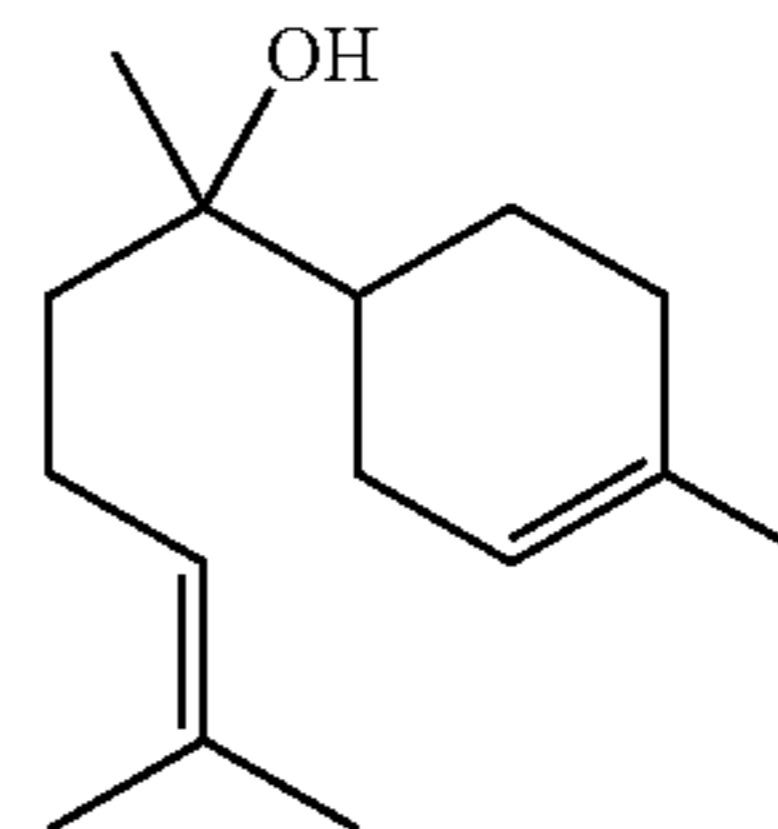
bisabolol
