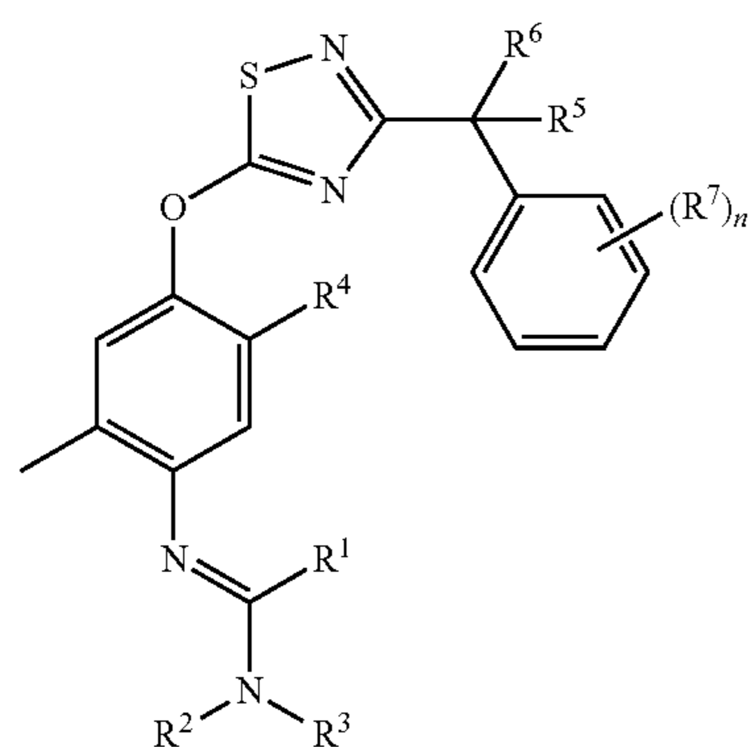
E-isomer
