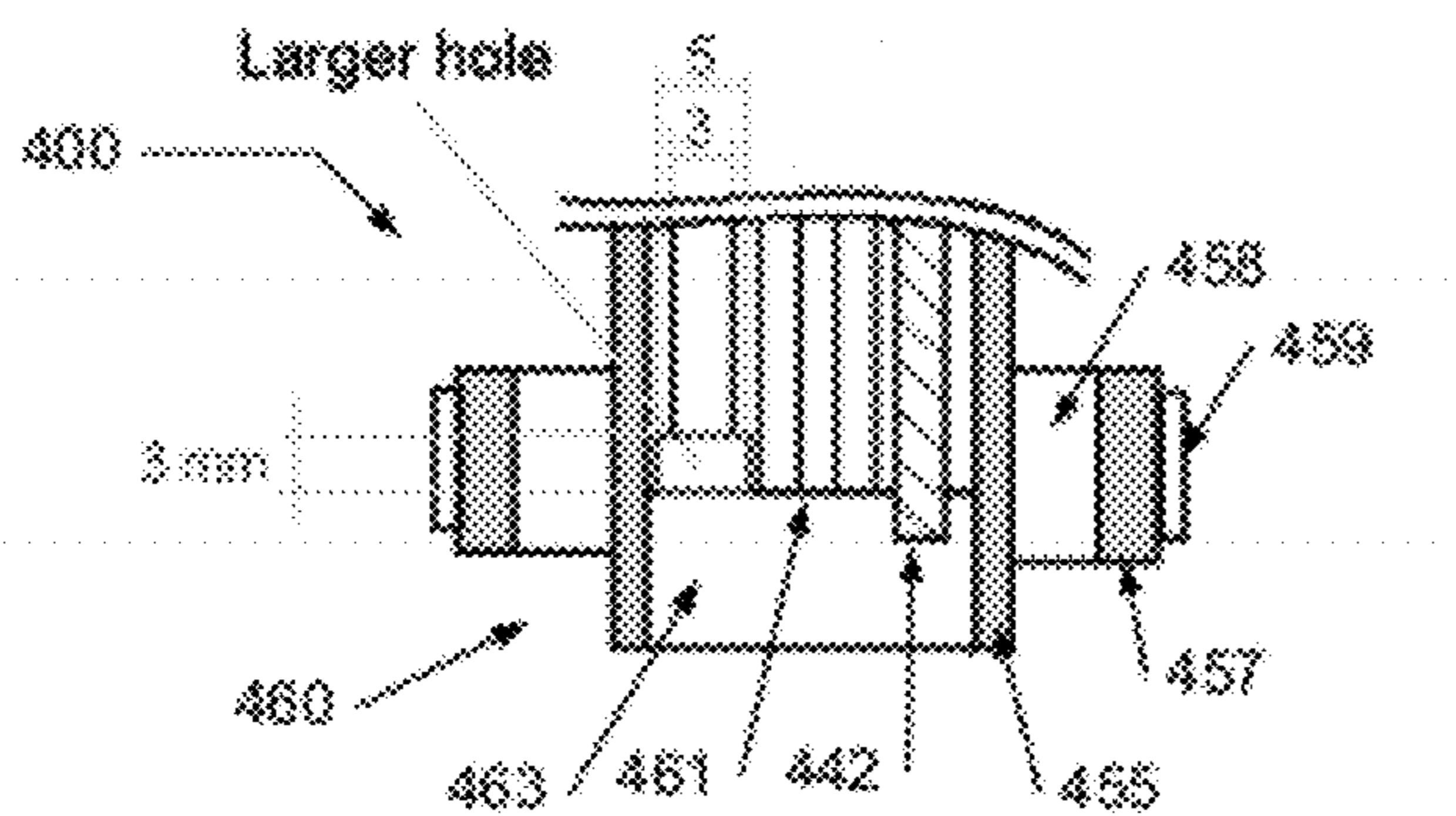
A-A view
