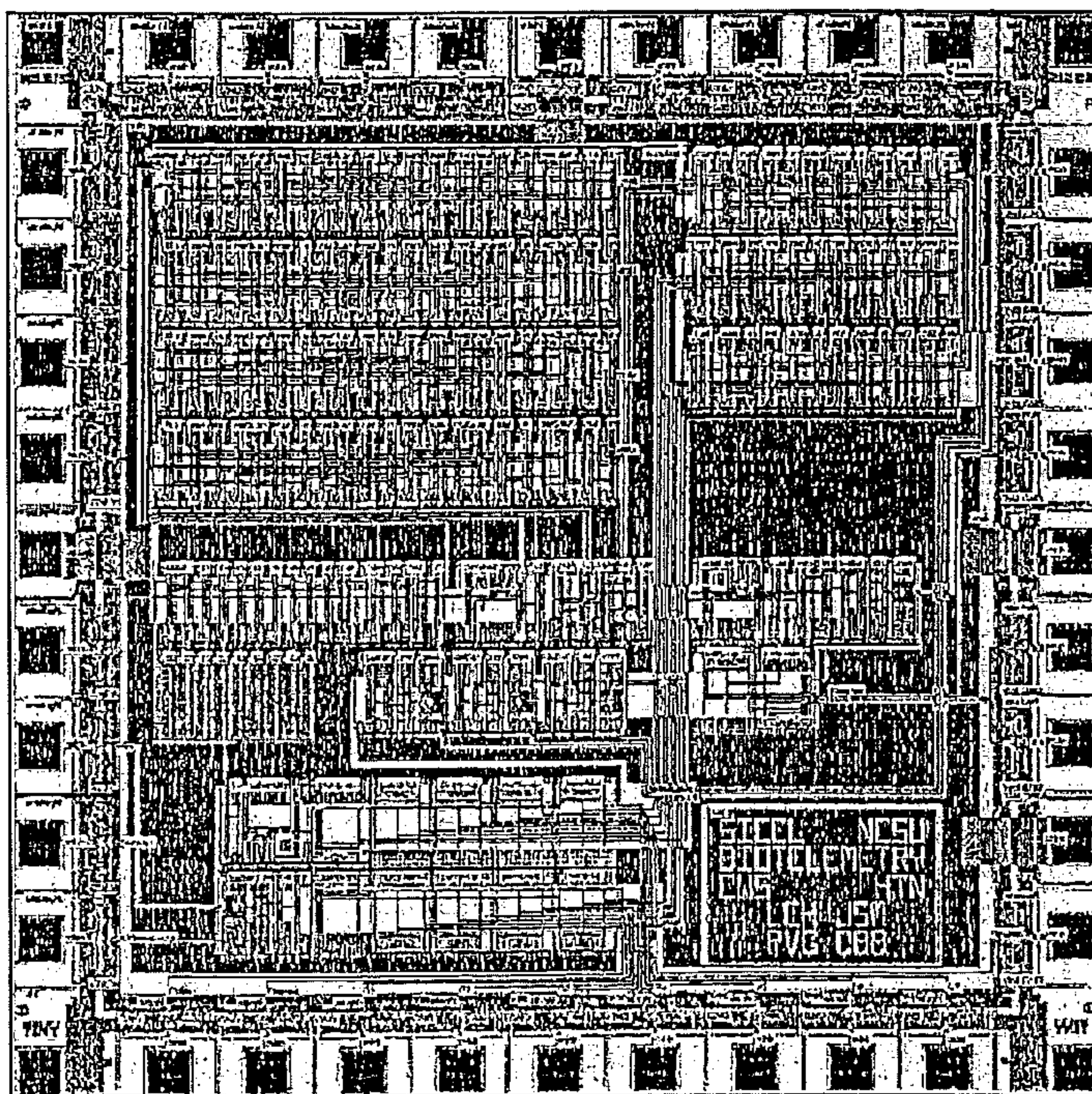
IC LAYOUT
