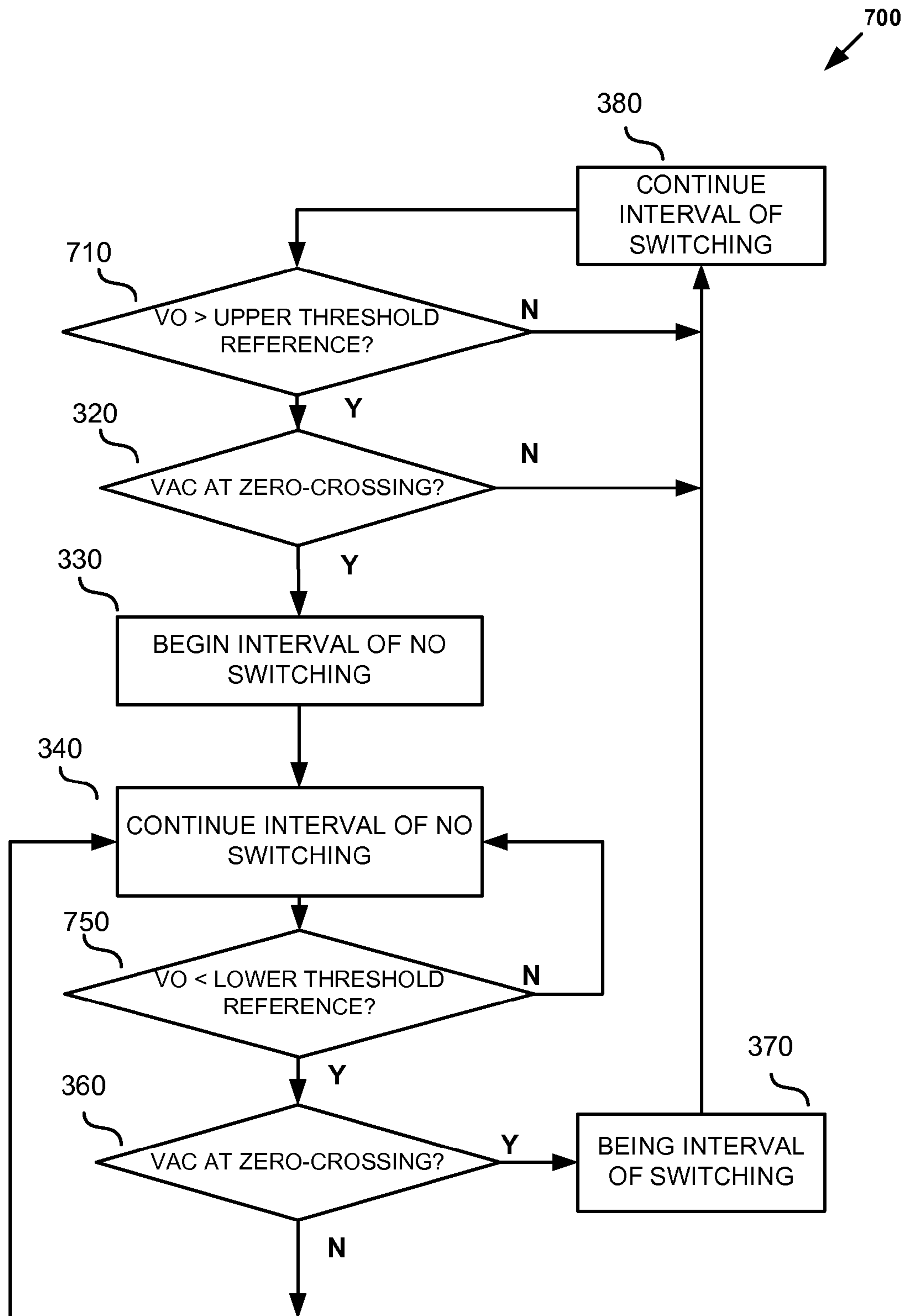
FIG. 7
