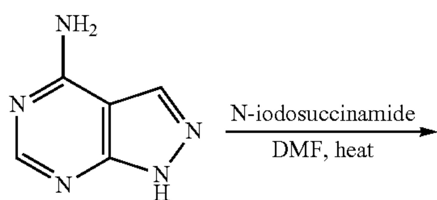
Scheme I.
