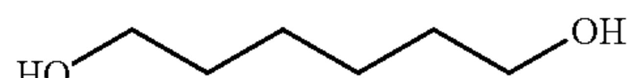
1,6-Hexanediol
