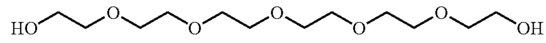
Hexaethylene glycol
