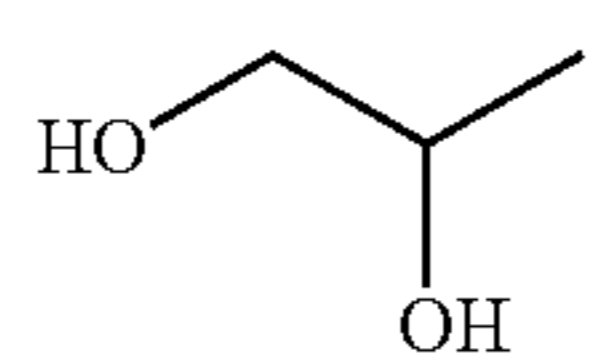
1,2-Propanediol
