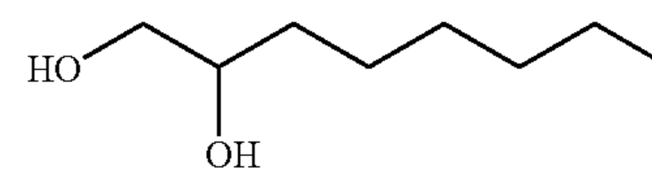
1,2-Octanediol
