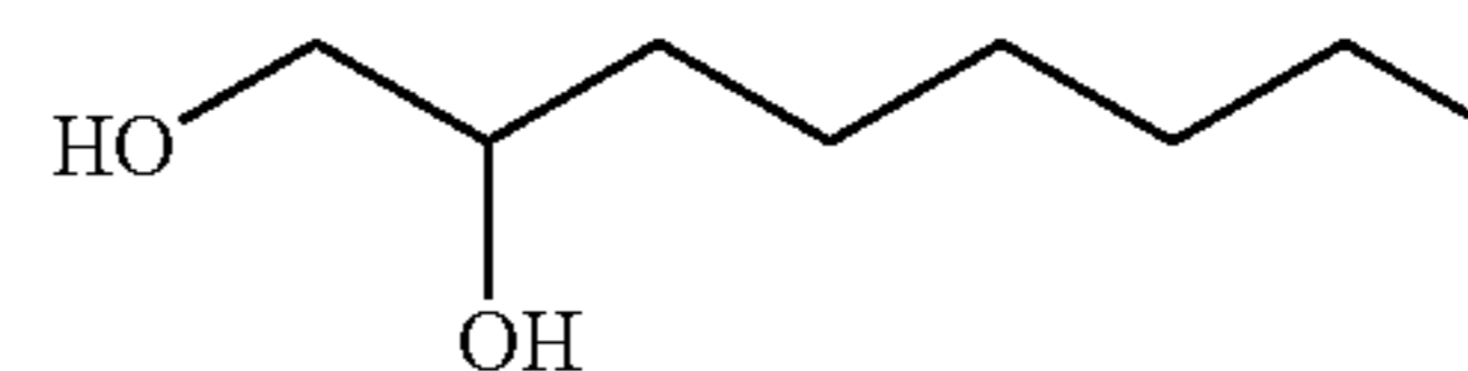
1,2-Octanediol
