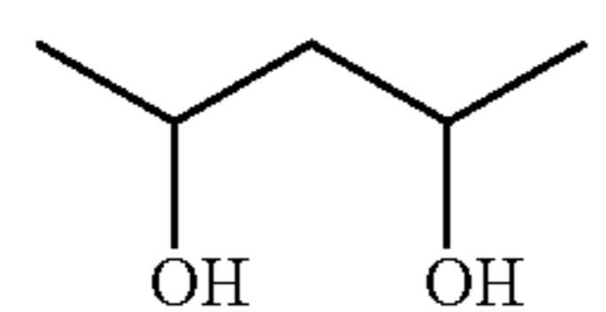
2,4-Pentanediol
