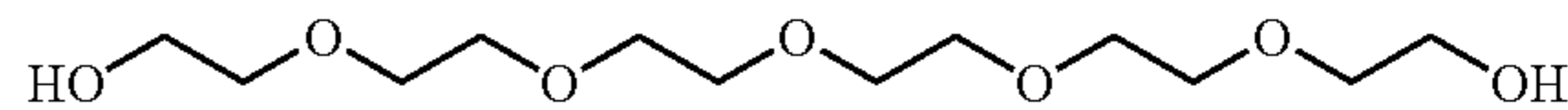
Hexaethylene glycol
