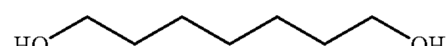
1,7-Heptanediol
