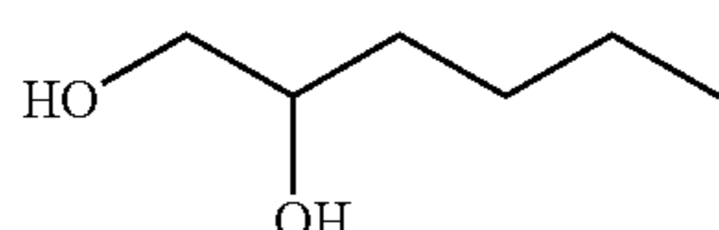
1,2-Hexanediol
