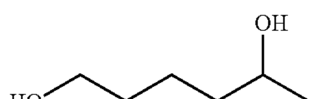
1,5-Hexanediol
