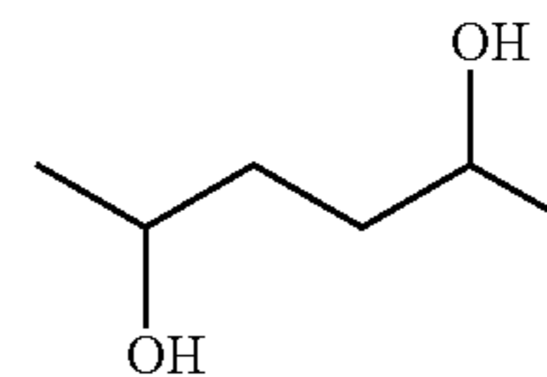
2,5-Hexanediol
