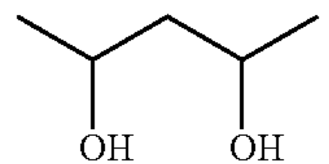
2,4-Pentanediol
