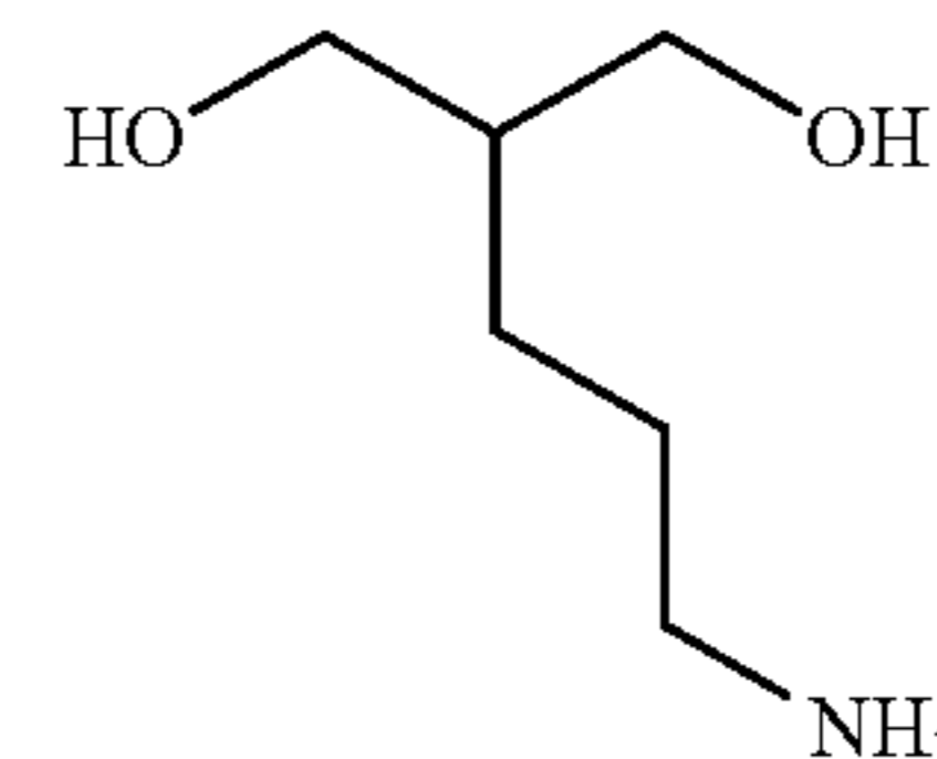
2-(1-Aminopropyl)-1,3-propanediol
