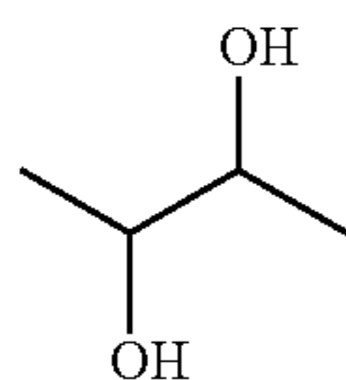
2,3-Butanediol
