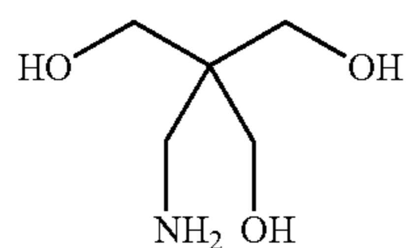
2-Amino-2-(hydroxymethyl)-1,3-propanediol
