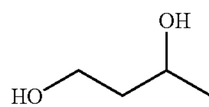
1,3-Butanediol
