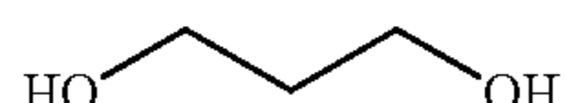
1,3-Propanediol
