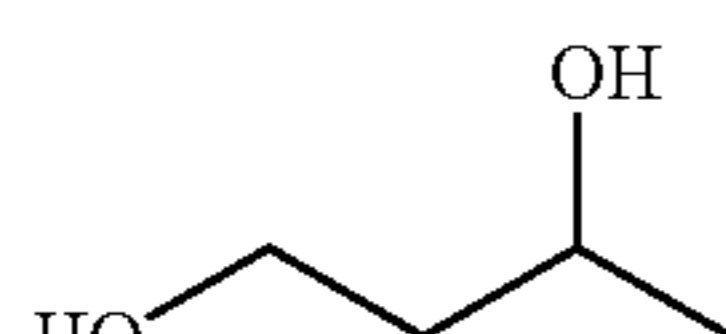
1,3-Butanediol
