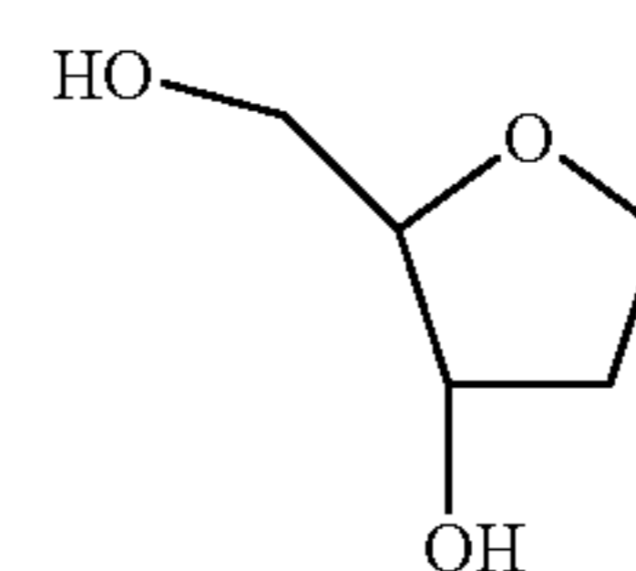
1,2-Dideoxyribose
