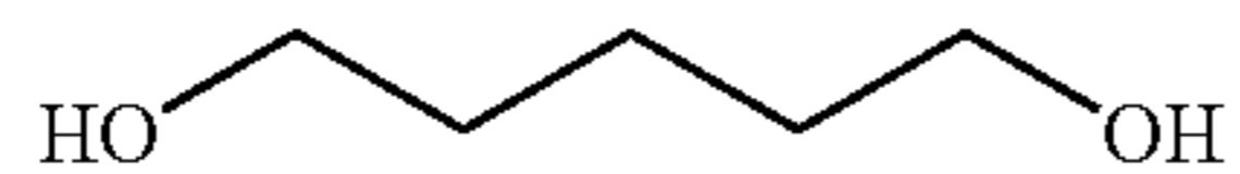
1,5-Pentanediol
