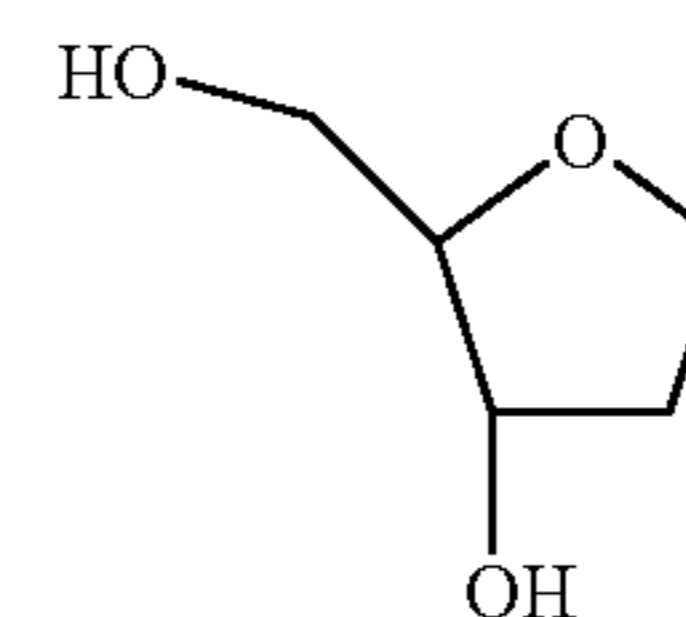
1,2-Dideoxyribose
