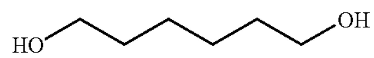
1,6-Hexanediol
