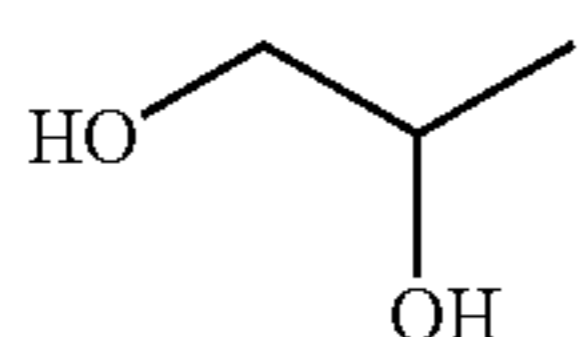
1,2-Propanediol
