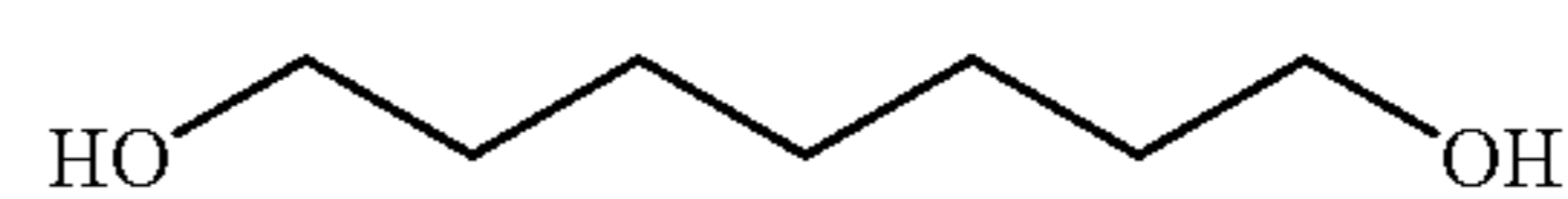
1,7-Heptanediol
