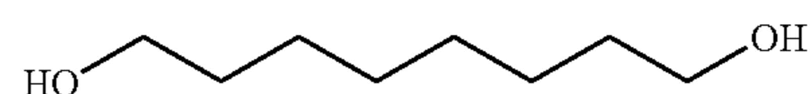
1,8-Octanediol
