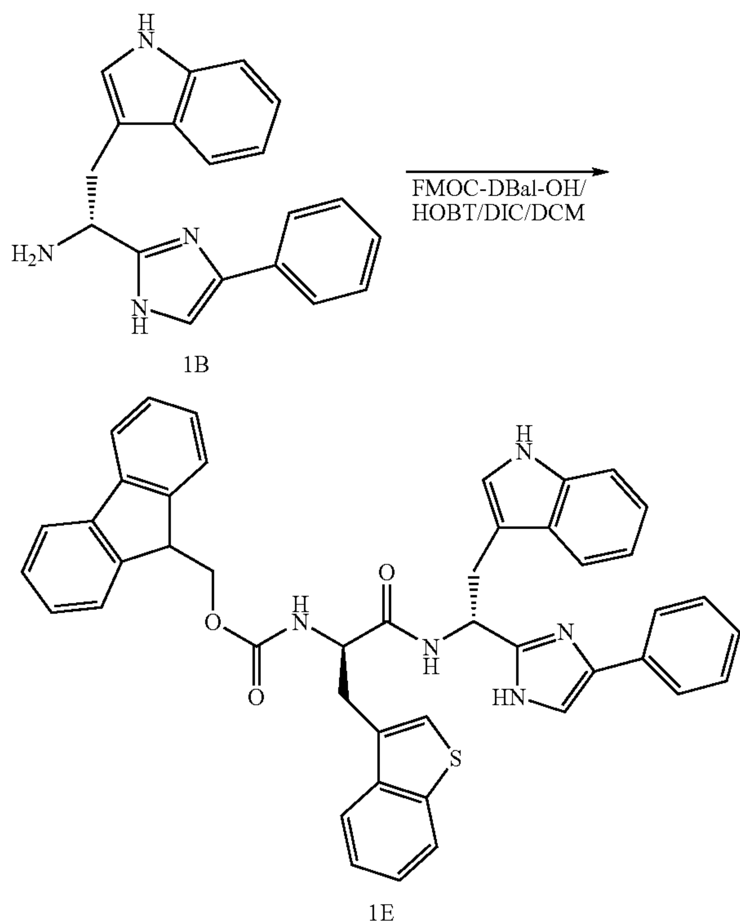
Scheme 1E
