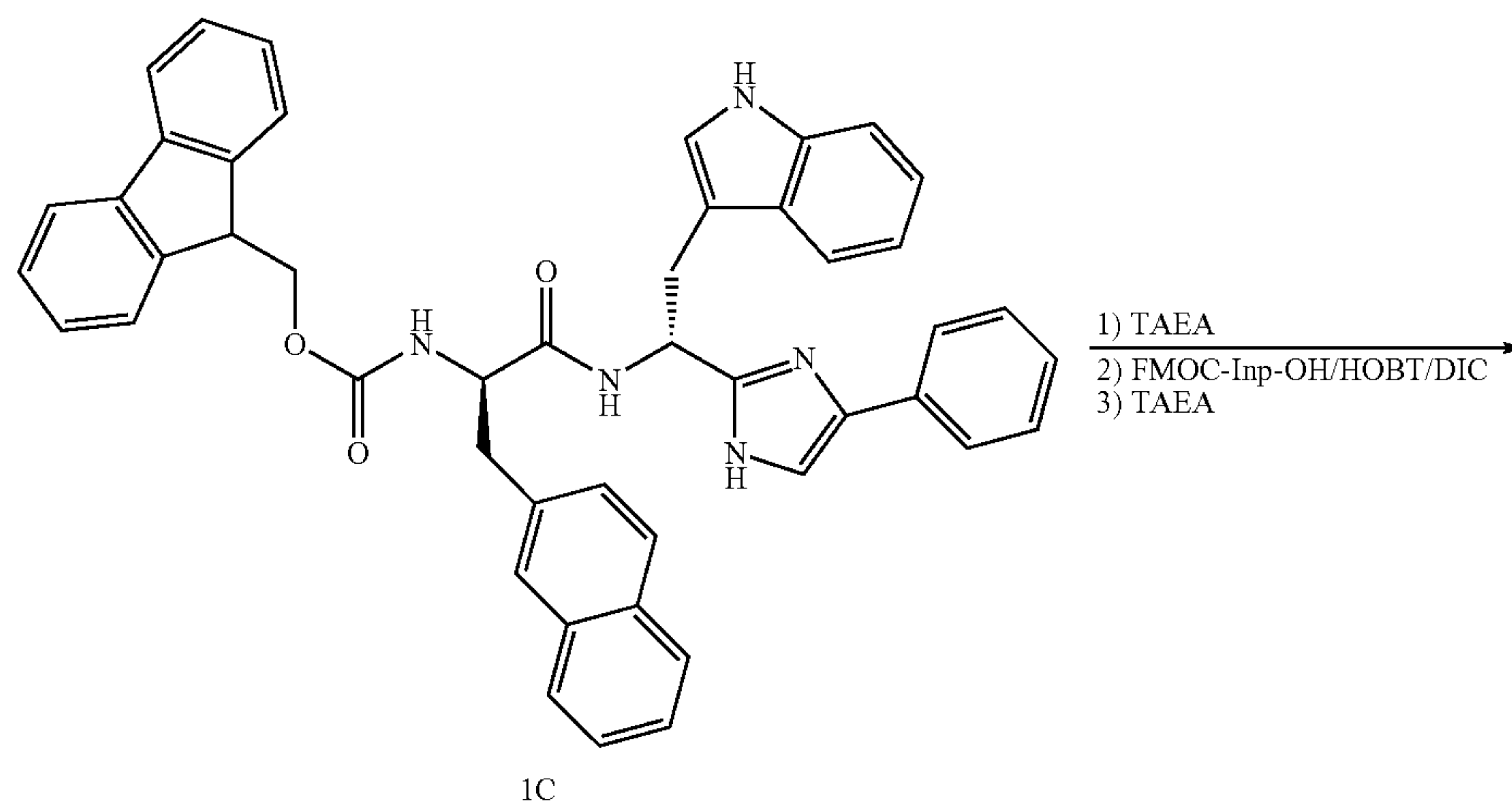
Scheme 1G
