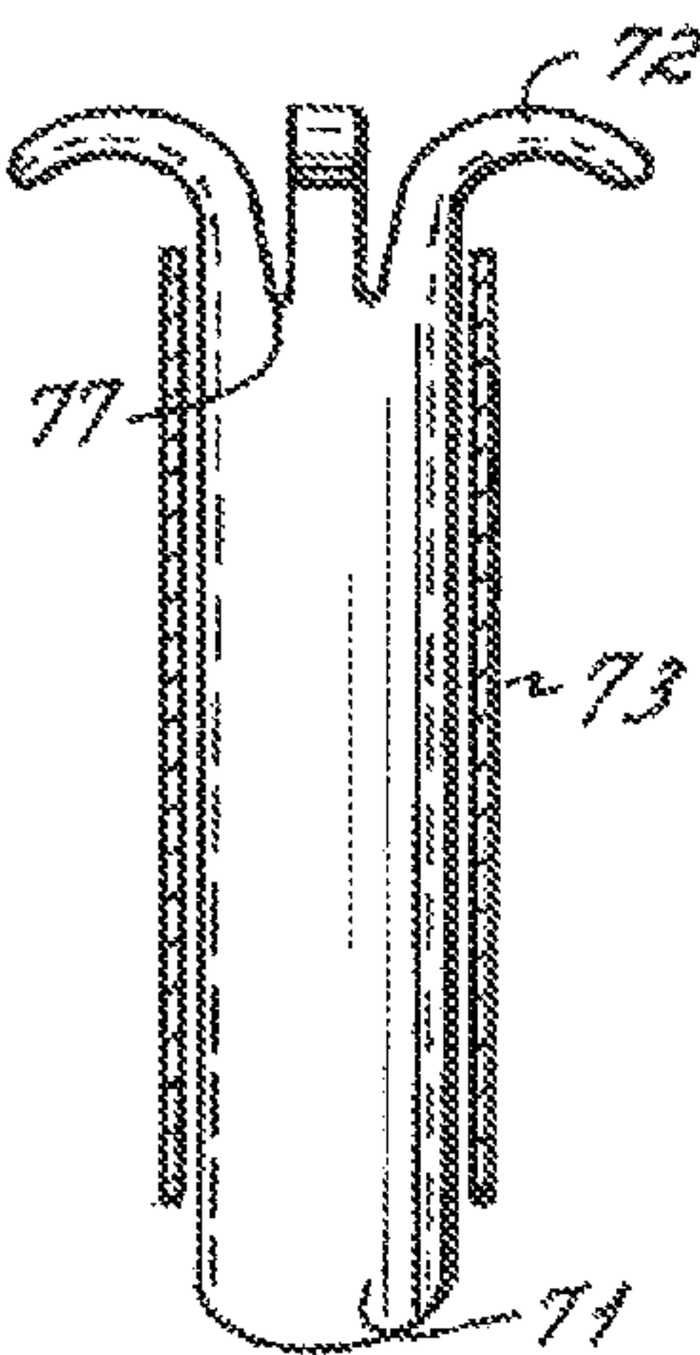
FIG. 7A
