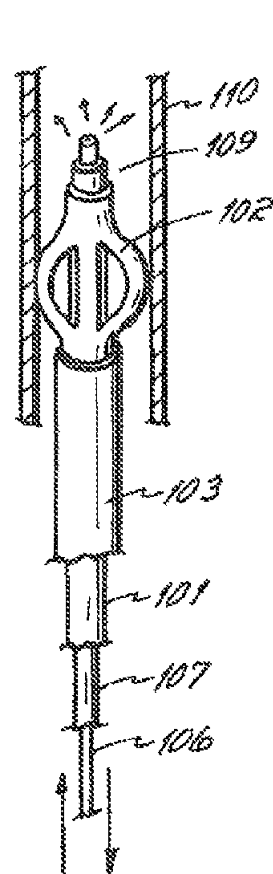
FIG. 10A
