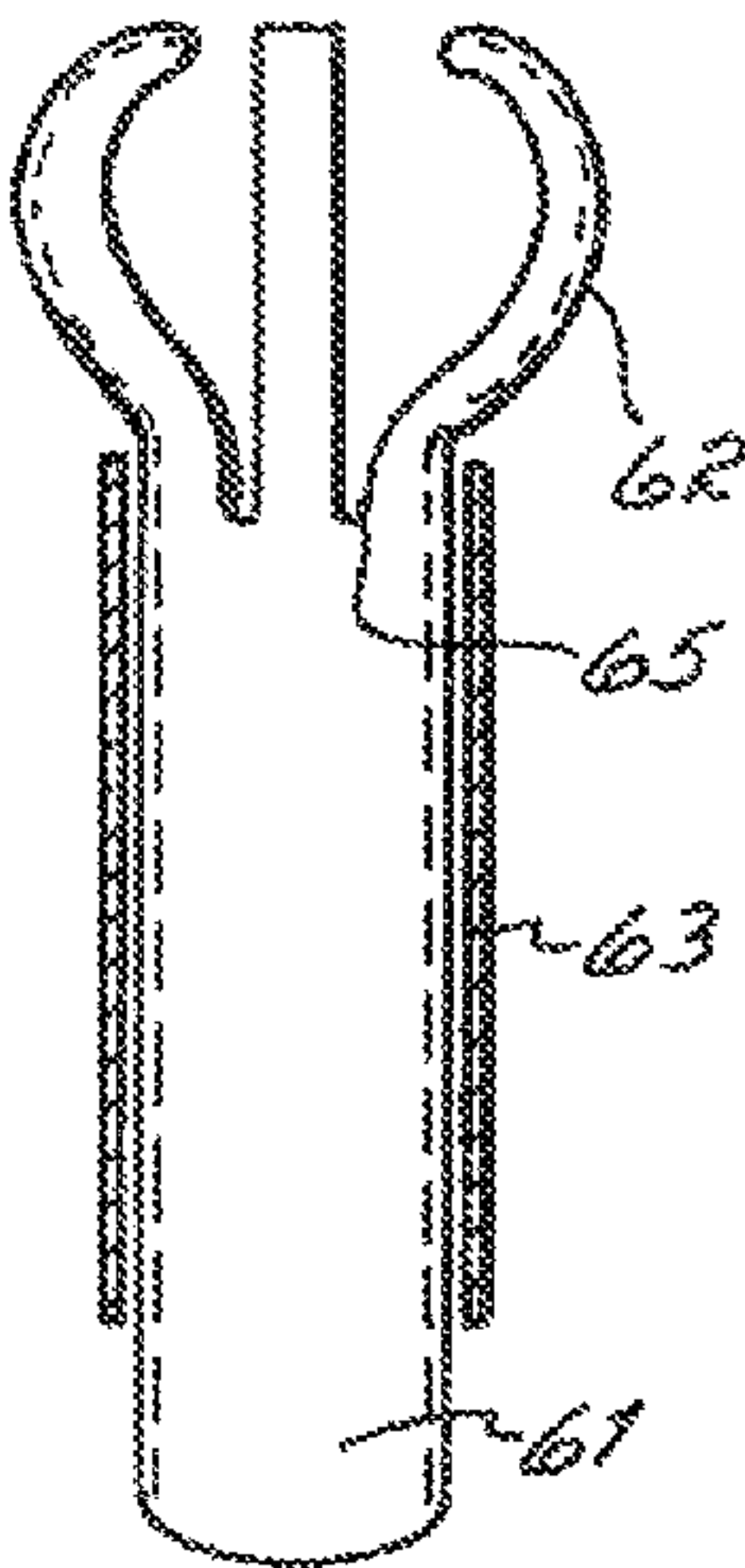
FIG. 6A
