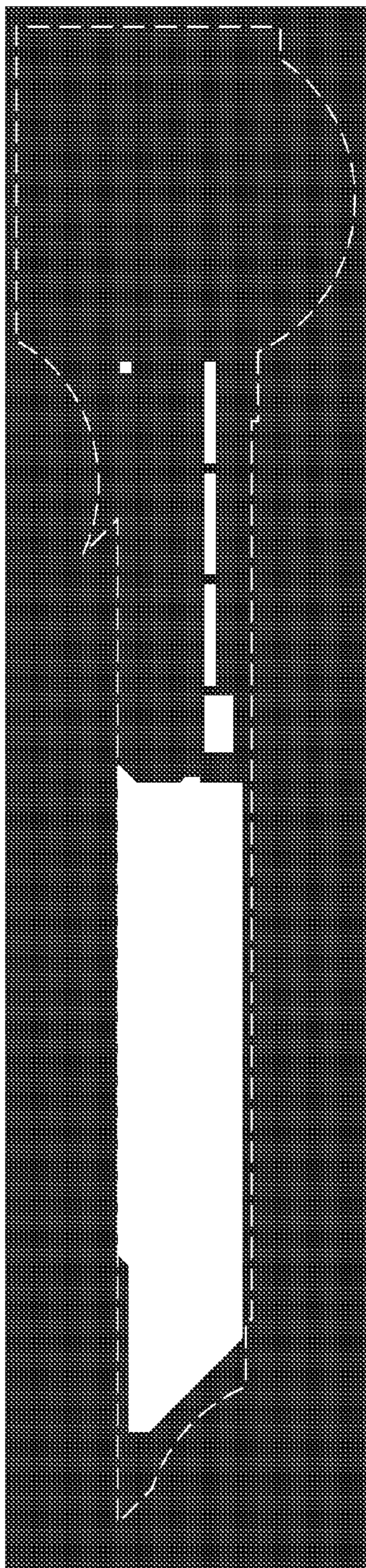
p+ mask
