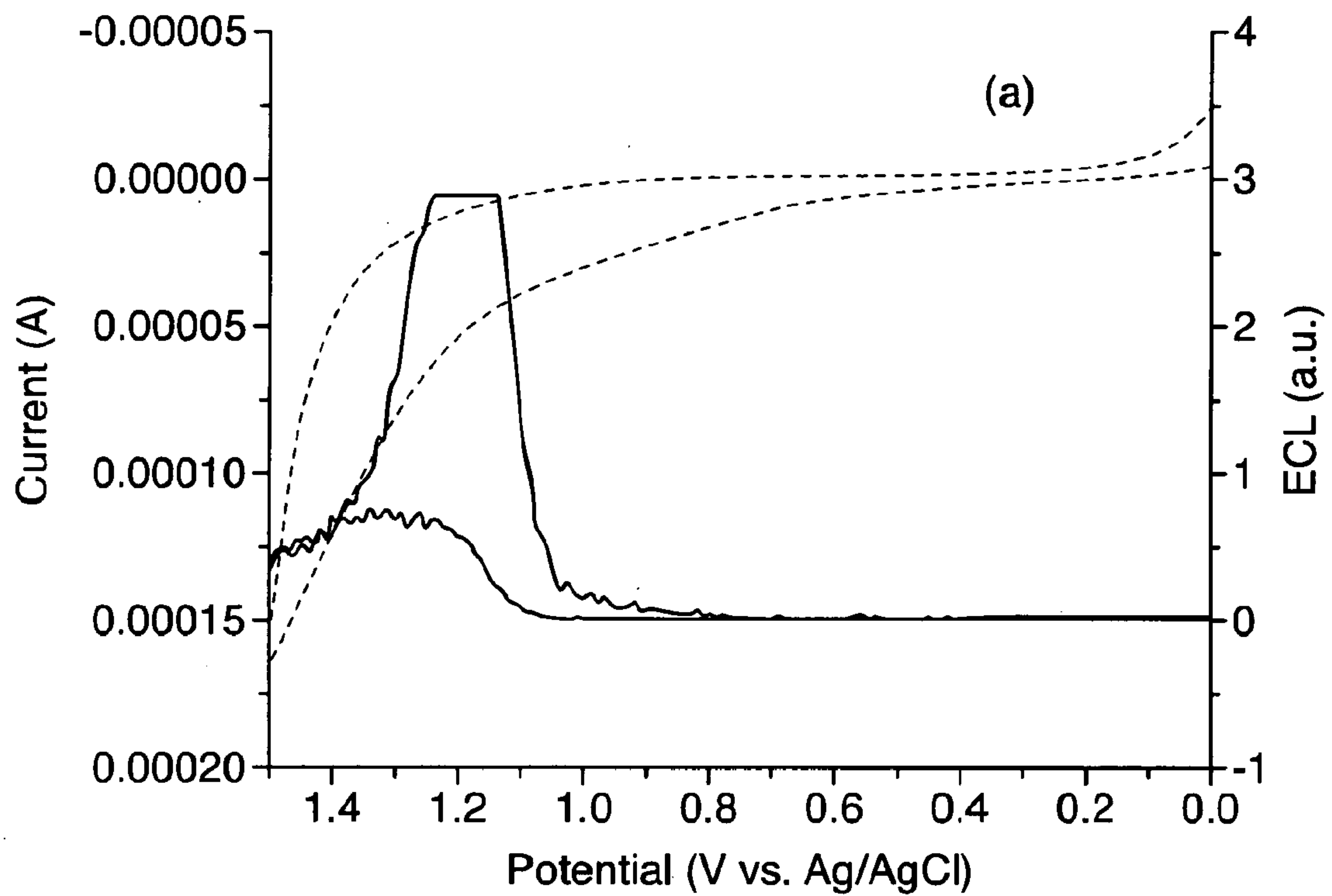
FIG. 5A
