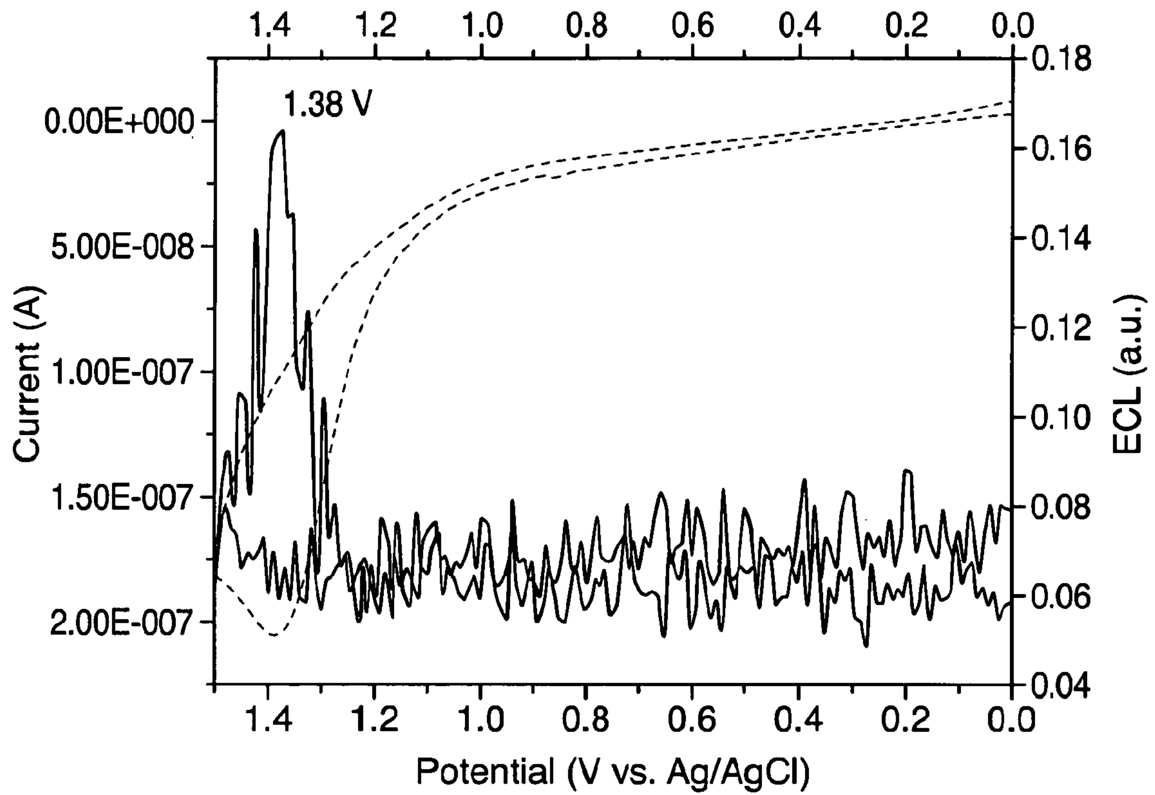
FIG. 6A
