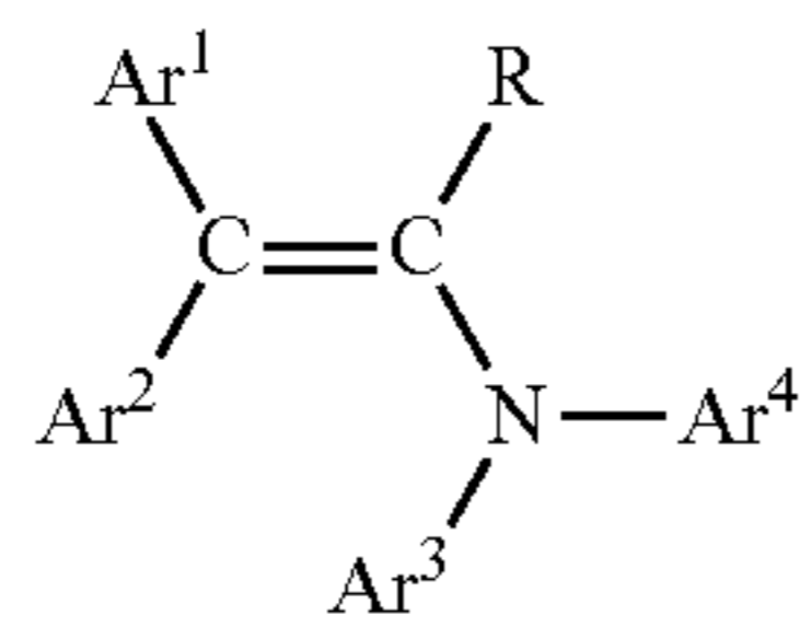
enamines
