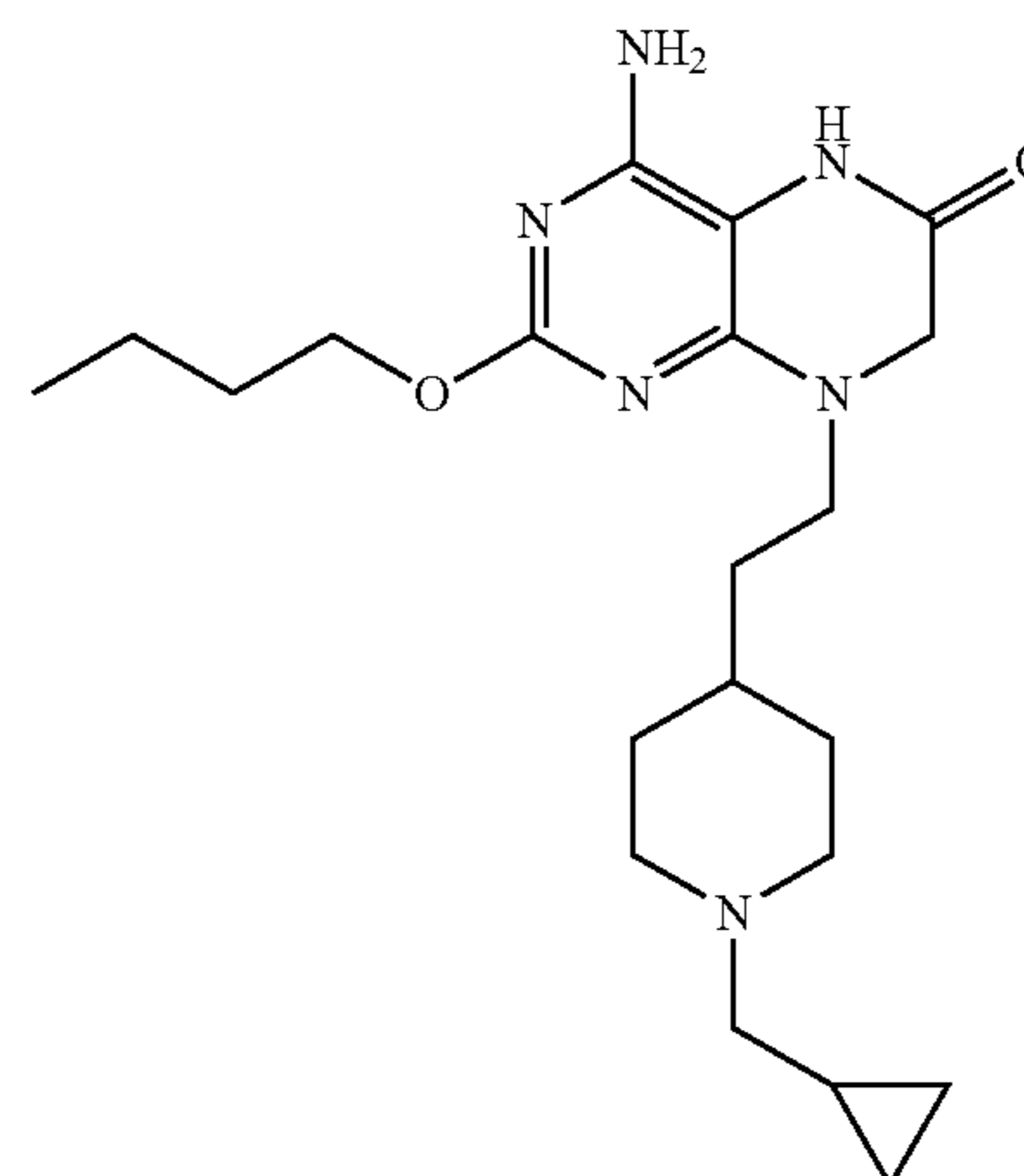
Example 113
