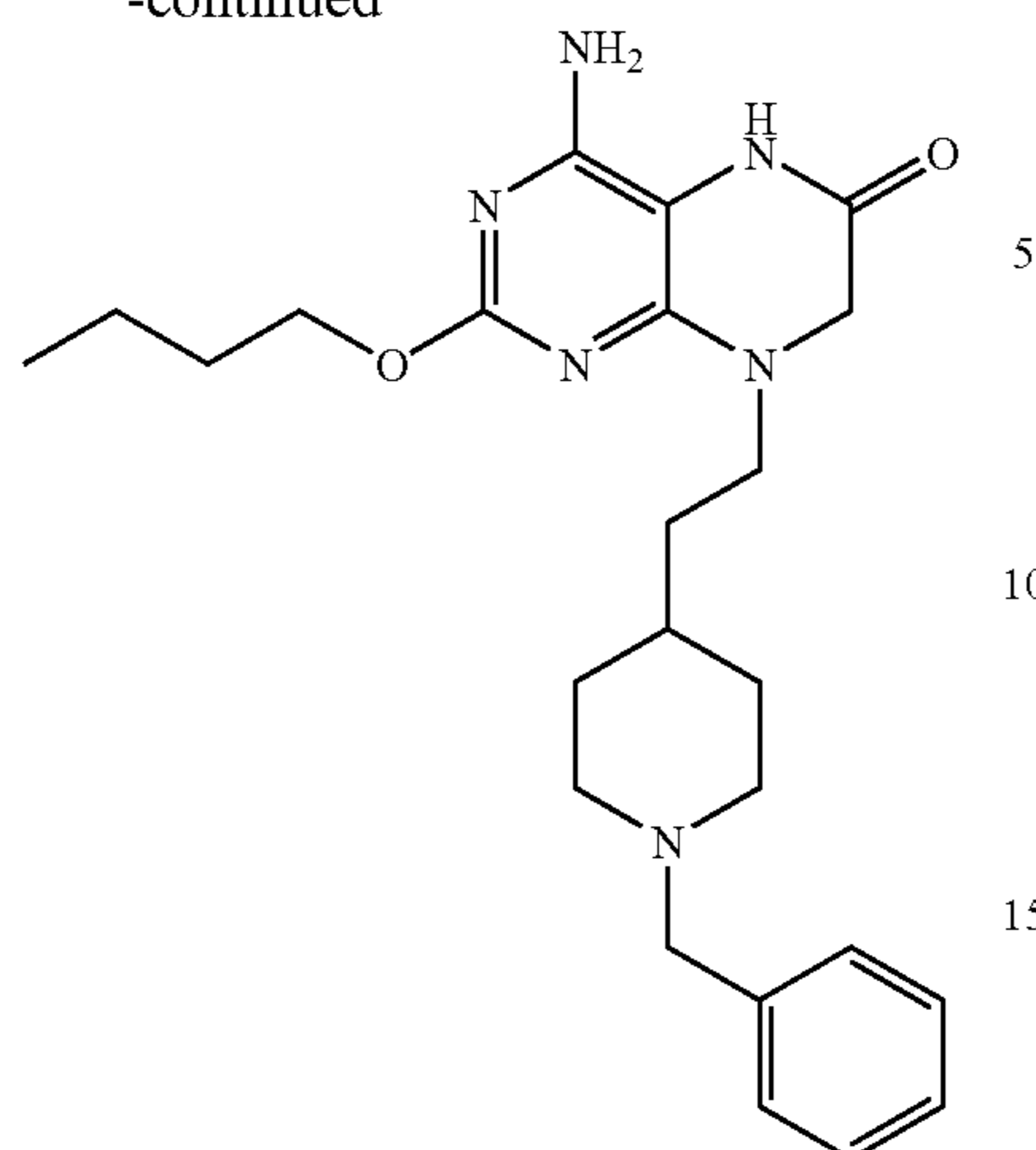
Example 108
