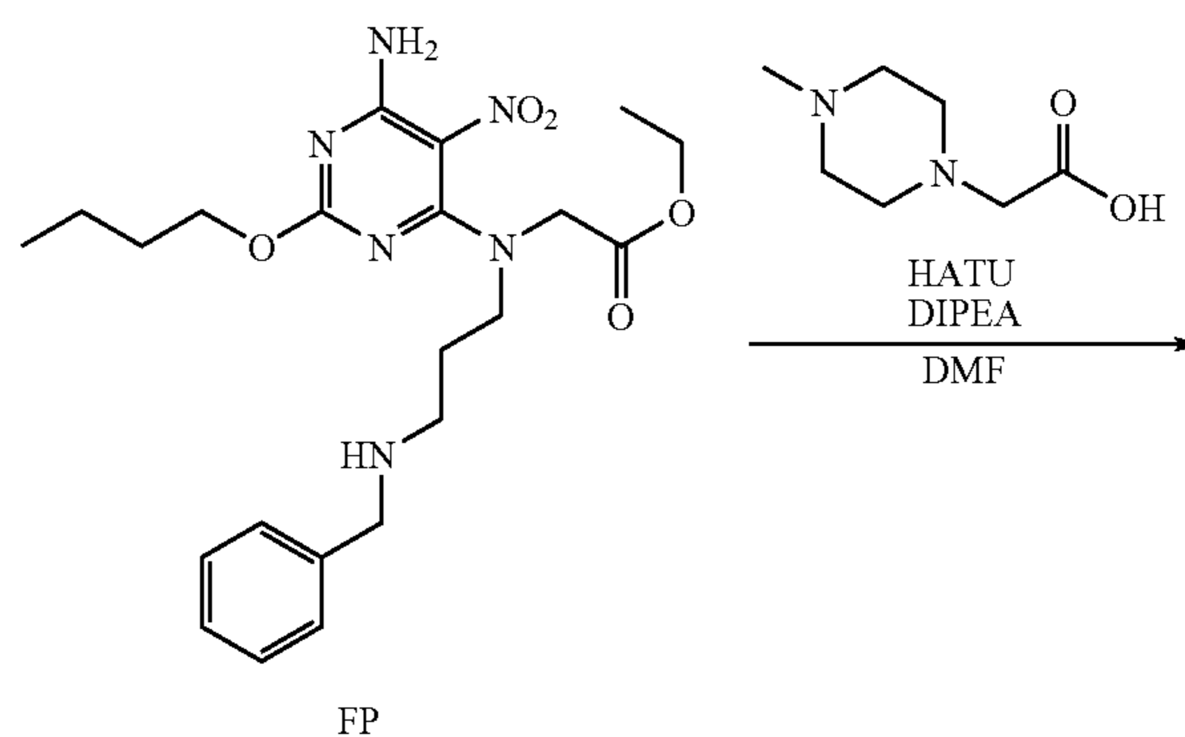
Scheme 107:
